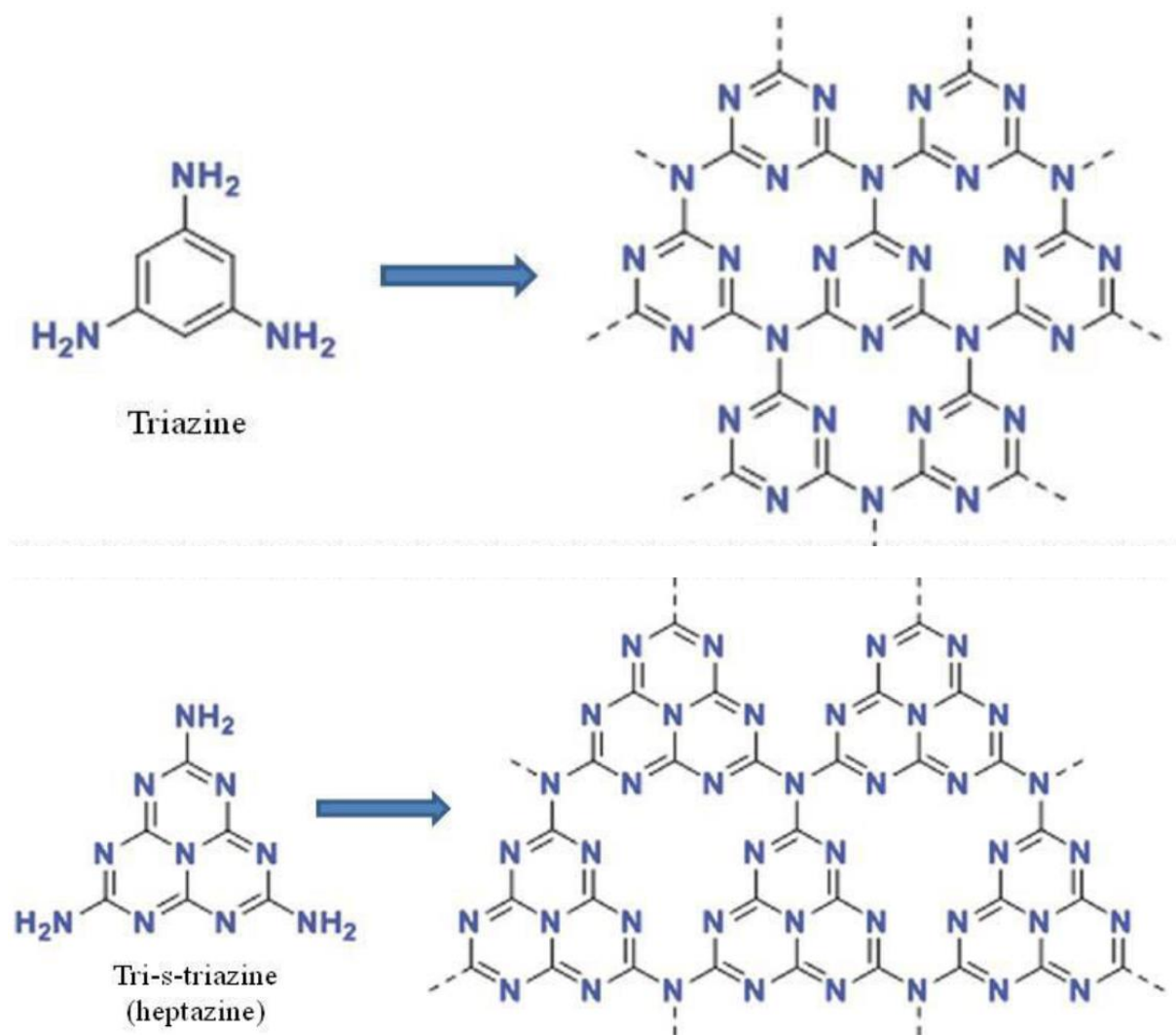
Figure 1.17 : Représentations des différentes unités constituantes du g\text{-C}_3\text{N}_4 69 .
