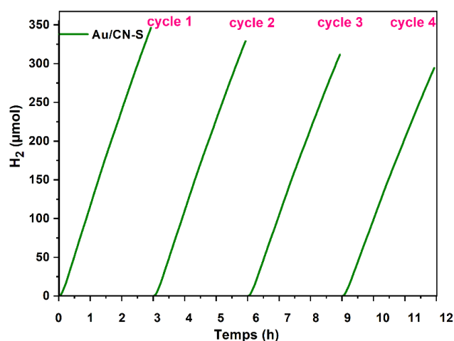
Figure 2.15 : Production cumulée de H 2 lors des tests de recyclabilité du nanocomposite Au/CN-S.
