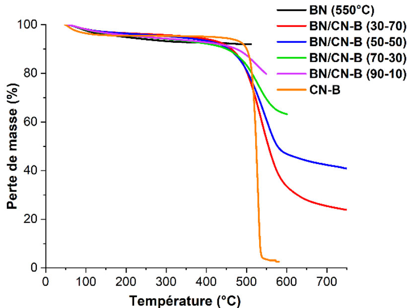
Figure 5.13 : Analyses thermogravimétriques des différents composites BN/CN-B, réalisées sous flux d'air ( 25\text{ mL}\cdot\text{min}^{-1} ) avec une rampe de montée en température de 15^\circ\text{C}/\text{min} .
