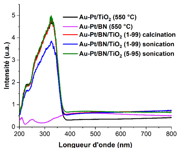
Figure 5.23 : Spectres d'absorption UV-Vis des nanocomposites Au-Pt/BN/TiO 2 .
