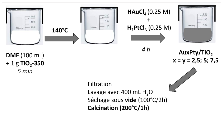
Figure 4.11 : Schéma de la synthèse par réduction thermique dans le DMF des catalyseurs monométalliques.
