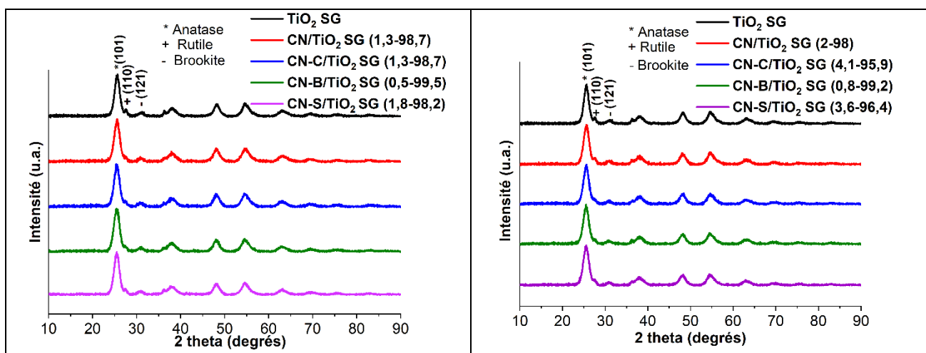
Figure 2.20 : Diagrammes normalisés de diffraction des rayons X du \text{TiO}_2 SG et des nanocomposites \text{CN}/\text{TiO}_2 SG et \text{CN-X} ( X=C, B, S )/ \text{TiO}_2 SG.
