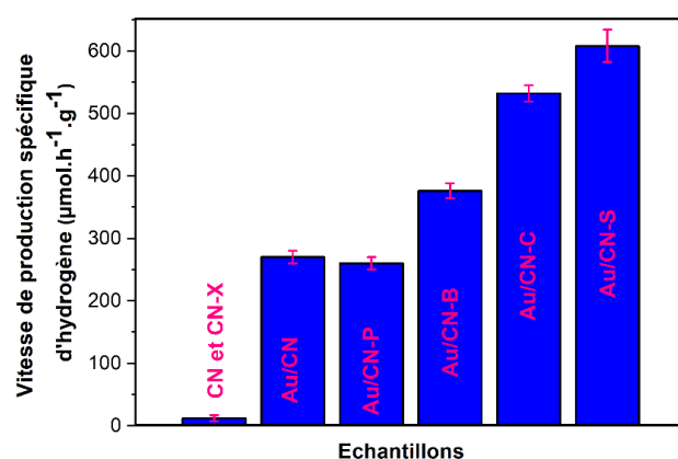
Figure 2.14 : Histogramme montrant les vitesses de production de H 2 sous irradiation solaire (1122 W.m -2 ), avec un flux de N 2 (100 ml.min -1 ), 1 vol.% de TEOA (agent sacrificiel) et 200 mg du catalyseur par les nanocomposites Au/CN et Au/CN-X (C, B,P,S), avec une incertitude expérimentale relative de 8 %.
