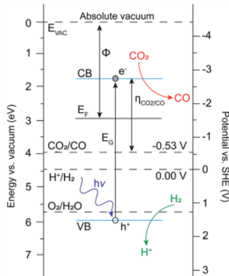
Figure 5.3 : Structure de bandes du BN poreux et potentiels redox d'H 2 O et CO 2 35 .
