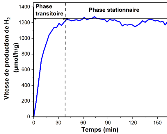
Figure 2.3 : Evolution de la production d'H 2 en fonction du temps.
