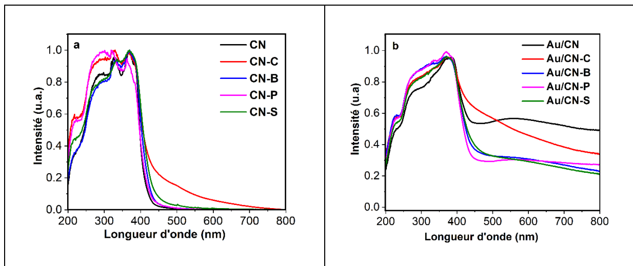
Figure 2.13 : Spectroscopie UV-Visible des CN et CN-X avant (a) et après (b) dépôt des nanoparticules d' Au.
