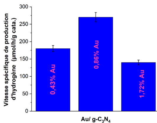
Figure 2.4 : Vitesse spécifique de production d'hydrogène par des nanocomposites Au/g-C 3 N 4 avec trois teneurs théoriques différentes en Au (0,43; 0,86 et 1,72 wt.%) sous irradiation solaire (1122 W.m -2 ), avec un flux de N 2 (100 mL.min -1 ), 1 vol.% de TEOA (agent sacrificiel) et 200 mg de catalyseur.
