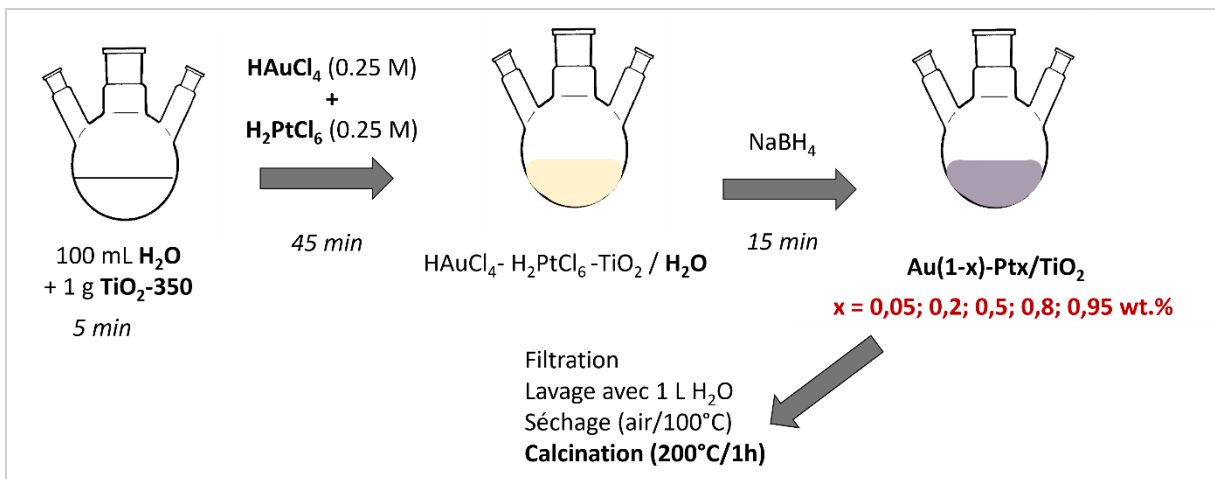
Figure 4.2 : schéma de la synthèse par imprégnation-réduction des catalyseurs bimétalliques.
