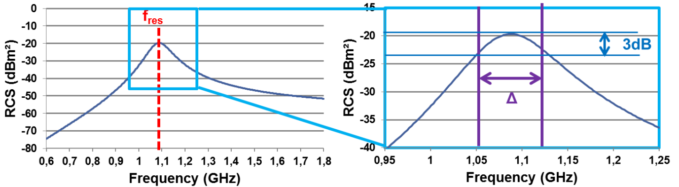
Figure 0-1: Extraction de la fréquence de résonance f_{res} et de la bande passante à -3\text{dB } \Delta
