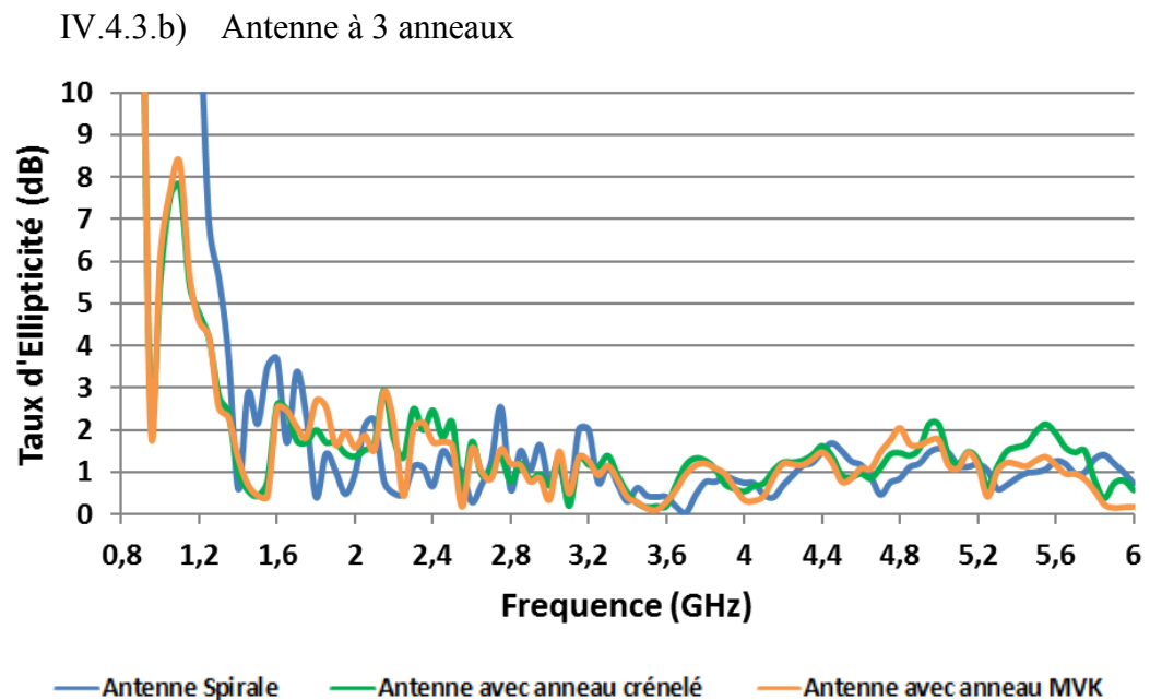
Figure IV-24: TE en dB des antennes à 3 anneaux en fonction de la fréquence dans la direction \theta=0^\circ
