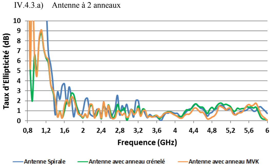
Figure IV-23: TE en dB des antennes à 2 anneaux en fonction de la fréquence dans la direction \theta=0^\circ
