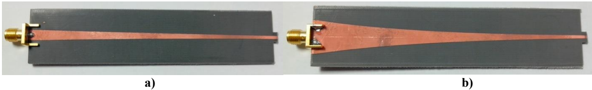
Figure II-34 : a) Profil de la ligne de transmission du balun et b) profil du plan de masse du balun Le Chapitre IV explicitera tous les détails sur l'alimentation des antennes.
