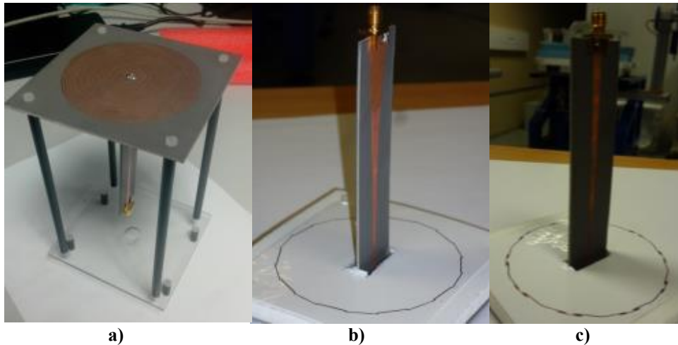
Figure IV-8: a) Antenne spirale, b) antenne spirale avec anneau à motif crénelé et c) antenne spirale avec anneau à motif VKM
