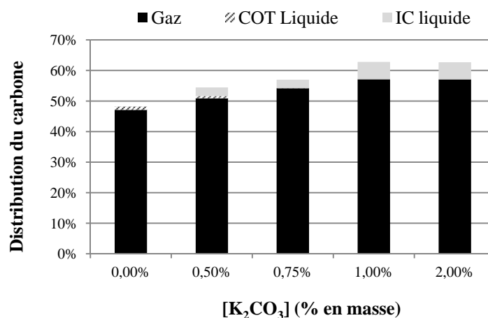
Figure 3-10 : Influence de la concentration de K_2CO_3 sur la distribution du carbone lors de la gazéification du glucose en eau supercritique (600°C, 25 MPa, 1 h, [glucose]=5% en masse, [ K_2CO_3 ]=0-2% en masse).
