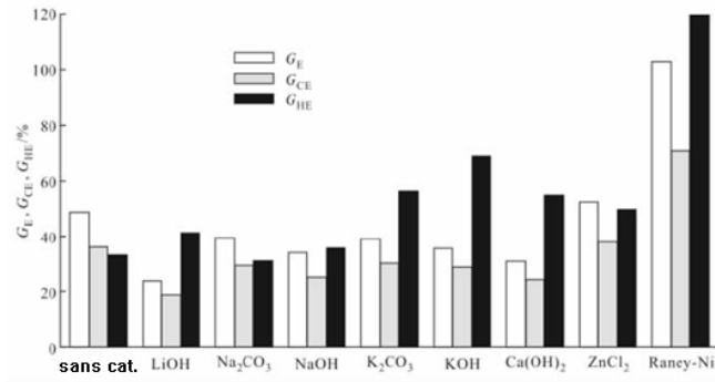
Figure 1-17 : Comparaison des activités des différents catalyseurs lors de la gazéification des coques d’arachide (400°C, 22-24 MPa) [83].
