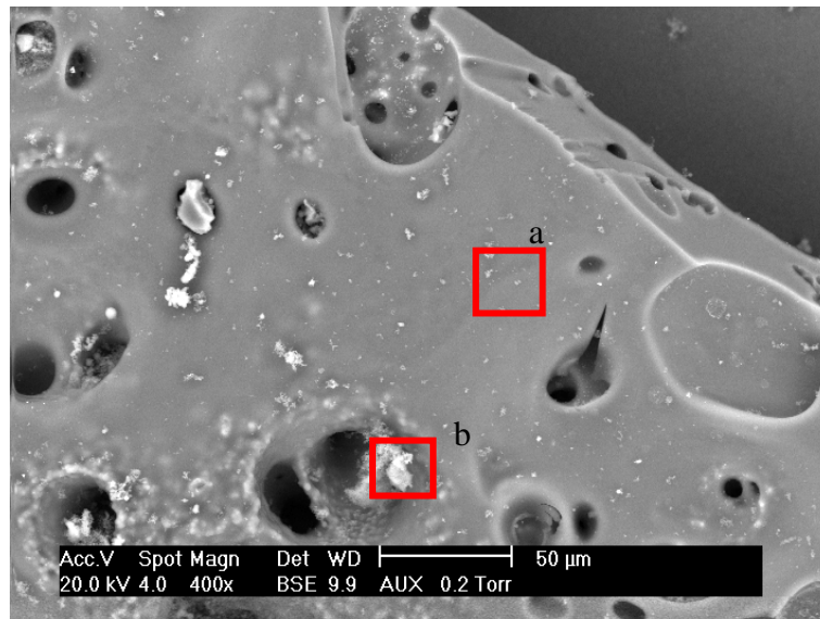
Figure 3-19 : Image du solide issu de la SCWG du glucose sans catalyseur (450°C, 25 MPa, 1 h, grand autoclave) analysé par MEBE (Echelle 50 µm).
