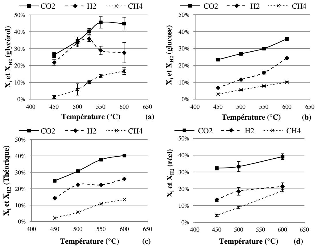
Figure 5-5 : Influence de la température sur X_i et X_{\text{H}_2} de différentes solutions traitées par le réacteur batch. (a): la solution de glycérol, (b): la solution de glucose; (c): la valeur moyenne théorique de a et b; (d) : la valeur expérimentale de la solution de mélange de glucose et glycérol. ([Glucose] = [glycérol] = 0,54 mol L -1 , 25 MPa, [K 2 CO 3 ] = 0,05 mol L -1 , 60 min.
