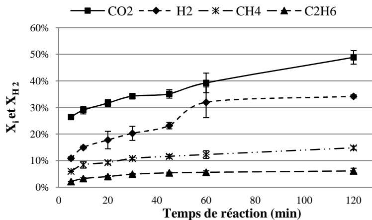
Figure 3-5 : Influence du temps de réaction sur le taux de conversion du carbone en gaz i ( X_i ) et le taux de conversion d'hydrogène en H 2 ( X_{H_2} ) (600°C, 25 MPa, 5-120 min, [glucose]=5% en masse, [K 2 CO 3 ]=1 % en masse).
