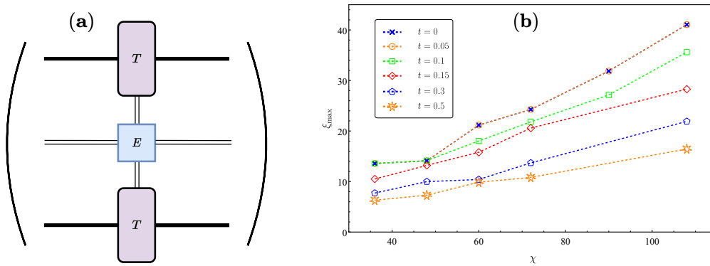
FIGURE B.16: (a) La matrice de transfert construite à l'aide du tenseur de bord T . (b) \xi_{\max} obtenu à partir du logarithme du rapport entre les valeurs propres principales et secondaires \frac{\lambda_2}{\lambda_1} de la matrice de transfert représentée.
