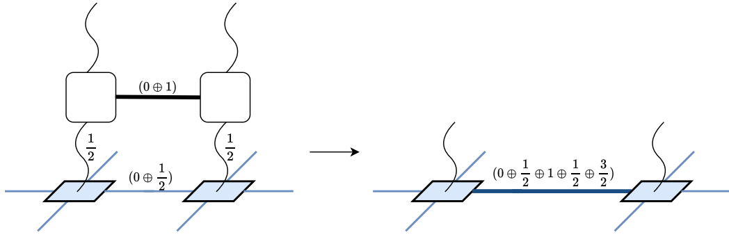
FIGURE B.11: L'espace virtuel résultant après l'application de la porte d'évolution temporelle. Le nouvel espace virtuel a une dimension D = 12 avec \mathcal{V} = (0 \oplus \frac{1}{2} \oplus 1 \oplus \frac{1}{2} \oplus \frac{3}{2}) . À l'aide des poids respectifs des différents spins, nous décidons d'utiliser les tenseurs D = 6 avec (\mathcal{V} = 0 \oplus \frac{1}{2} \oplus 1) pour capturer au mieux la dynamique de l'état NN-RVB.
