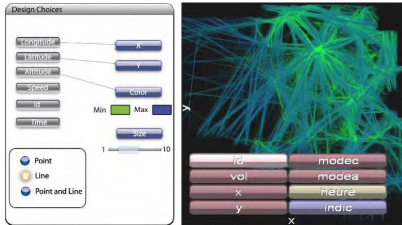
FIGURE 3.18 – FromDaDy : vue générale de l’interface [Hurter 09].
