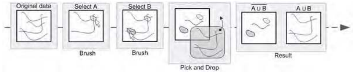
FIGURE 3.19 – FromDaDy met en œuvre des opérateurs booléens pour manipuler les vues.
