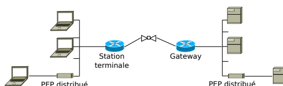
FIGURE 7.5 – Topologie du réseau employée pour nos expérimentations avec satellite
