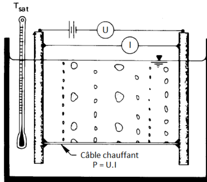
Figure I.6 – Expérience de Nukiyama. Illustration issue du livre de Lienhard [93]
