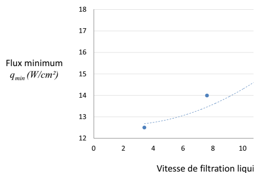
Figure IV.15 – Influence du débit sur la valeur du flux minimum q_{min}
