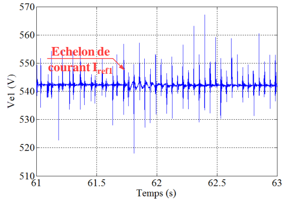
(b) Evolution de la tension V_{e1} après l'application d'un échelon du courant I_{ref1}
