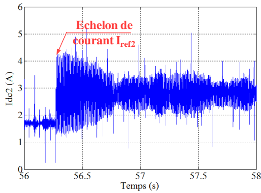
(a) Evolution du courant I_{dc2} après l'application d'un échelon du courant I_{ref2}
