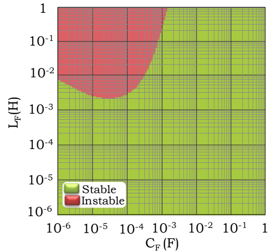
Fig. 98 Abaque de stabilité
