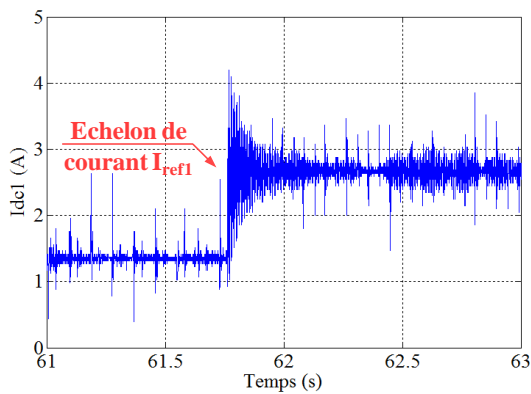
(a) Evolution du courant I_{dc1} après l'application d'un échelon du courant I_{ref1}
