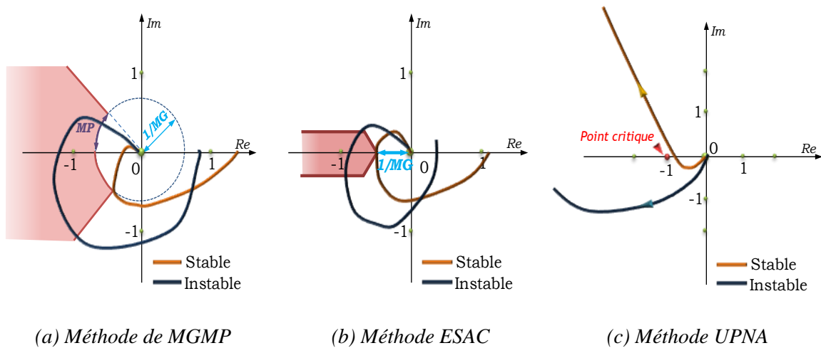
Fig.20 Critère de Middlebrook
