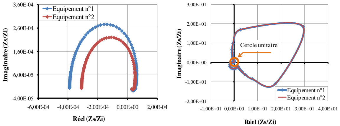
(a) Diagramme de Nyquist correspondant au 1 er point d'étude Fig. 112(a)
