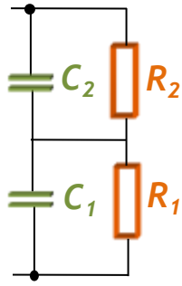
Fig.45 Circuit du condensateur d'entrée
