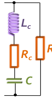
Fig.46 Circuit de la cellule équivalente du condensateur d'entrée
