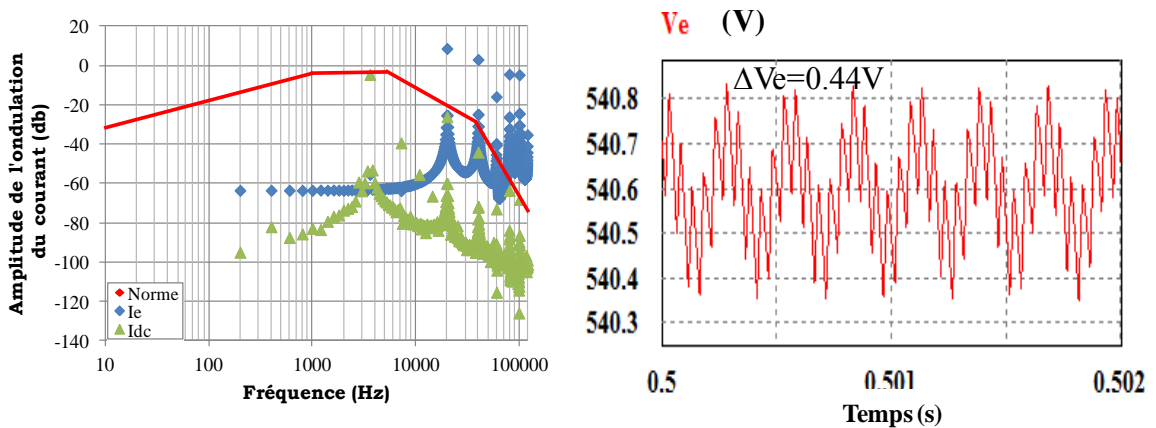
Fig. 94 Résultats de simulation de l'ensemble du système : F_{gen} = 600Hz
