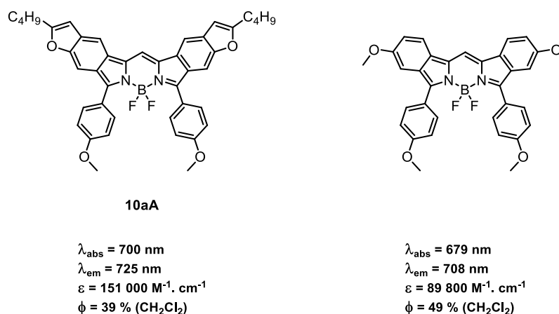
Figure 2-32 Comparisons des propriétés spectroscopiques de 10aA et du BODIPY tétraméthoxy
