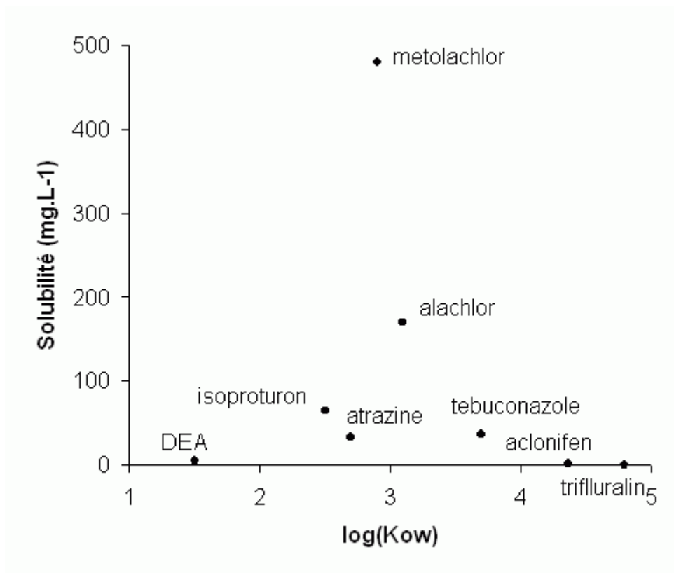
Figure 14. Répartition des 8 pesticides étudiés sur le bassin versant de la Save (dont le metolachlor, l’acлонifen et la trifluralin qui ont été modélisés) en fonction de leur solubilité ( \text{mg.L}^{-1} ) et de leur lipophilie quantifiée par le coefficient de distribution octanol/eau \log(K_{ow}) (d’après Tomlin, 2009).
