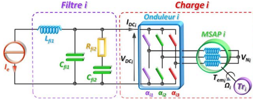
FIG. 2.28 – Sous-Ensemble du réseau HVDC
