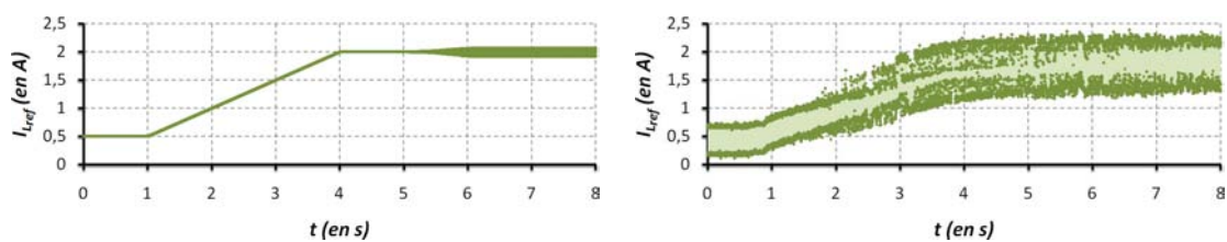
(a.) Résultat obtenu en simulation
