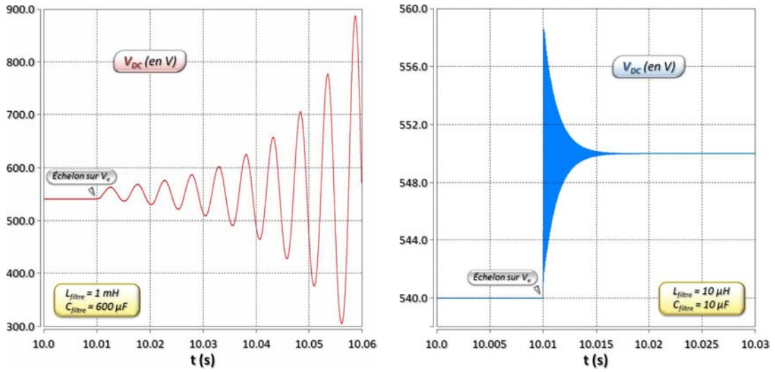
(a.) Dimensionnement du concepteur ( L_{filtre} = 1\text{ mH} , C_{filtre} = 600\text{ }\mu\text{F} )
