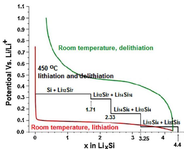
Figure 1.17. Courbe électrochimique obtenue lors de la première lithiation et de la délithiation du silicium cristallin (respectivement en rouge et en vert) à température ambiante et à 450°C (en noir). Extrait de Wu et al. 90
