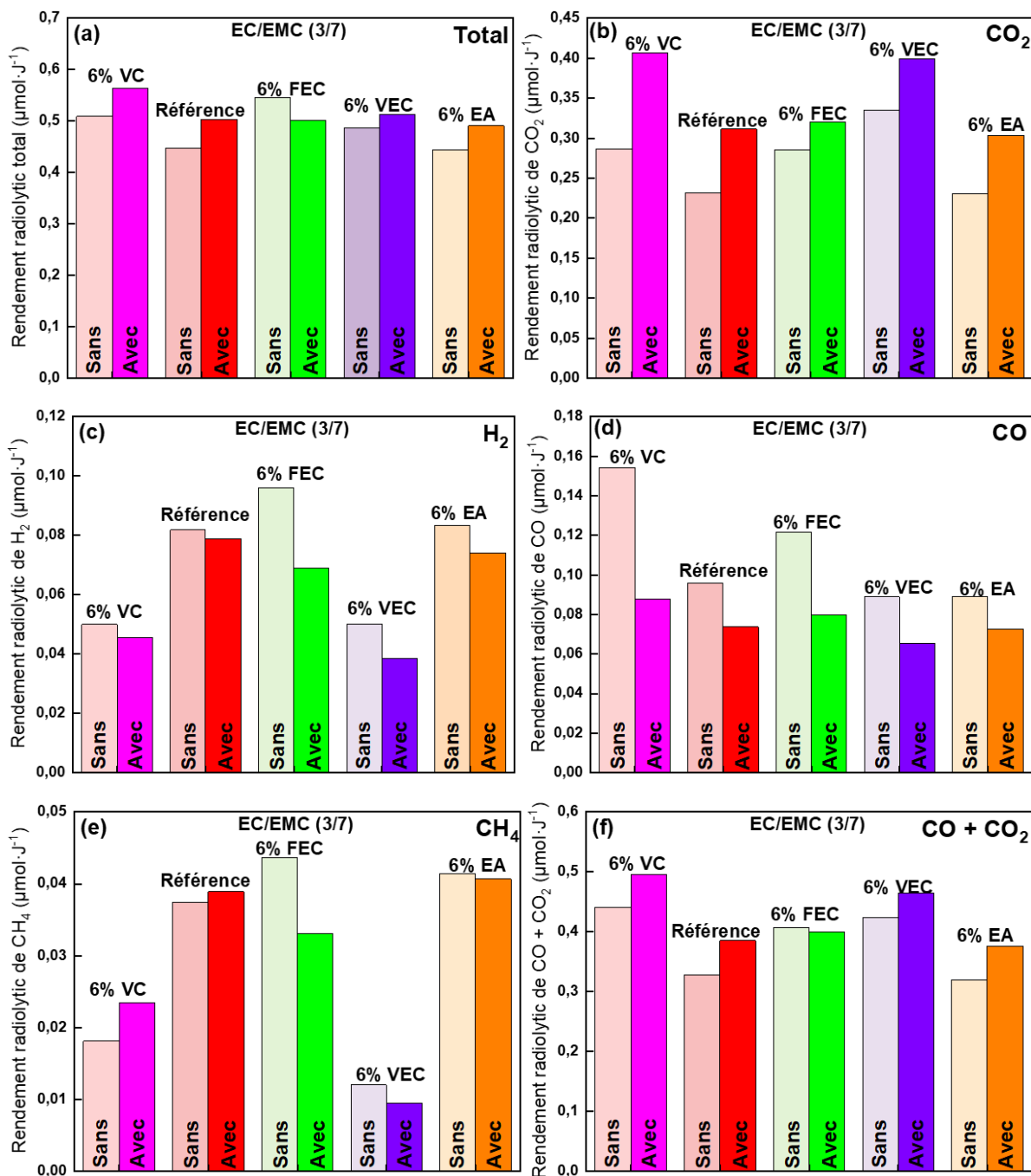
Figure 3.8. Evolution des rendements radiolytiques (a) du total des quatre gaz, (b) de \text{CO}_2 , (c) de \text{H}_2 , (d) \text{CO} , (e) de \text{CH}_4 et (f) de \text{CO} + \text{CO}_2 après irradiation d'EC/EMC (3/7) sans ou avec \text{LiPF}_6 (1 M) en présence de différents additifs.
