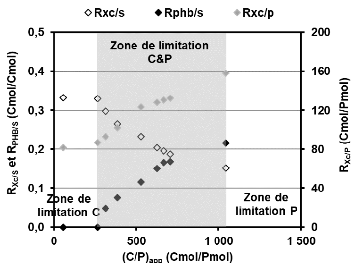
Figure 17. Rendements observés en cellules catalytiques ( X_c ) et PHB par rapport au substrat ( R_{(Xc/S)} et R_{(PHB/S)} , respectivement) et de X_c par rapport au phosphore ( R_{(Xc/P)} ) en fonction du degré de limitation phosphore appliqué ((C/P)_{app}) pour une culture continue conduite à D = 0,045 \text{ h}^{-1} ; la zone de DLN est représentée en gris (Cavaillé et al., 2016).
