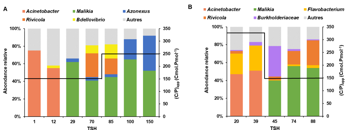
Figure 42. Dynamiques de sélection sur butyrate/propionate, respectivement durant la campagne B1 (A) et B2 (B) : abondance relative des populations bactériennes en fonction du nombre de TSH et du (C/P)_{app} . Les genres bactériens représentant moins de 4% de l'ADN 16S total ont été regroupés sous la dénomination « Autres ».
