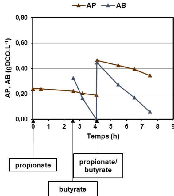
Figure 54. Evolution des concentrations en propionate (AP) et butyrate (AB) au cours du batch opéré avec une population microbienne préalablement sélectionnée sur un mélange acétate/butyrate (batch C1b).
