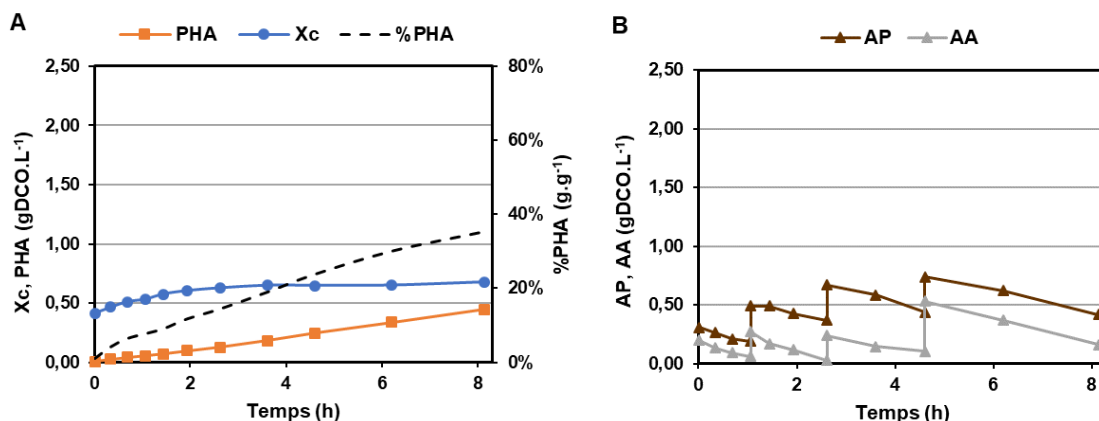
Figure 55. Evolution des concentrations en PHB, cellules catalytiques ( X_c ) et de la teneur en PHA ( A ), ainsi que celles en propionate (AP) et acétate (AA) ( B ) au cours du batch opéré avec consortia microbien sélectionné sur un mélange acétate/propionate à un (C/P)_{app} de 150 \text{ Cmol.Pmol}^{-1} (batch A2a).
