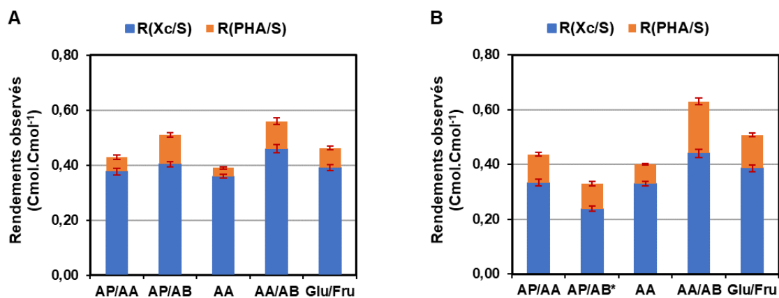
Figure 38. Rendements en biomasse catalytique (Xc) et PHA en fonction de la nature de la source de carbone pour des degrés de limitation en phosphore (C/P)_{app} de 250 (A) et 325 \text{Cmol.Pmol}^{-1} (B). La valeur des rendements observés à (C/P)_{app} = 325 \text{ Cmol.Pmol}^{-1} pour le substrat AP/AB est différenciée des autres car il s'agit du seul substrat pour lequel la valeur du degré de limitation a été appliquée directement, sans imposer de (C/P)_{app} inférieurs préalables.
