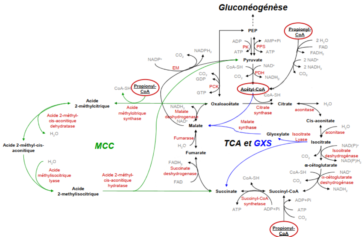
Figure 7. Voies d'entrée de l'acétate et du propionate dans le métabolisme central carboné (Grousseau, 2012).
