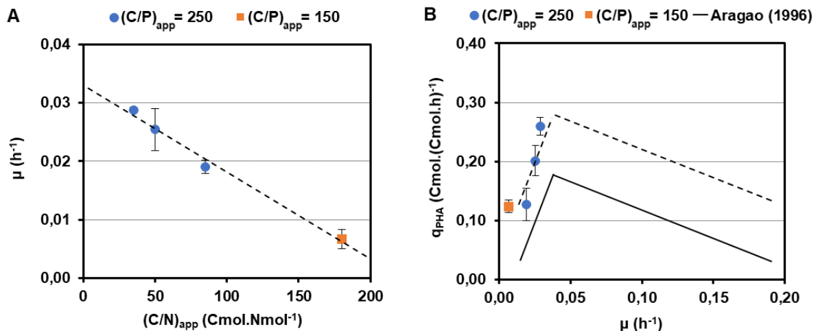
Figure 77. Evolution du taux de croissance spécifique ( \mu ) en fonction du degré de limitation (C/N)_{app} dans l'étage de production (A). Evolution de la vitesse spécifique de production de PHA en fonction du taux de croissance spécifique ( \mu ) dans l'étage de production (B). Le trait continu représente la relation établie par Aragao (1996) en conditions de limitation N. Le trait discontinu représente la projection pour les résultats obtenus, selon cette même relation.
