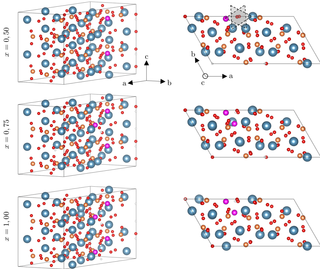
FIGURE 4.11 – Supers mailles a \times b \times c = 2 \times 1 \times 2 les plus stables pour différents taux de substitution x en cobalt. Les triangles de calcium/cobalt autour d'un canal d'hydroxydes sont indiqués. Code couleur : calcium (bleu), cobalt (rose), phosphore (orange), oxygène (rouge) et hydrogène (blanc).
