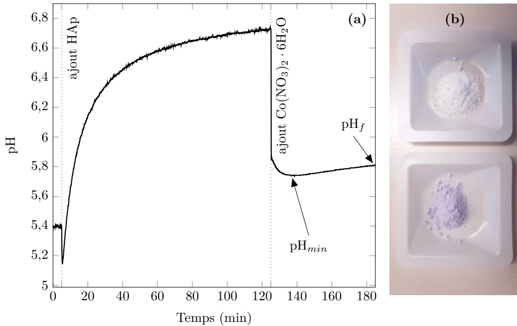
FIGURE 3.5 – Profil de pH caractéristique du protocole de dépôt du cobalt (1,00 g d'échantillon d'HAp 2*, m_{sel} = 0,200 g et t = 1 h), sans basification préalable de la solution de dépôt (a). Changement de couleur d'une HAp avant (blanc) et après (mauve-rose) dépôt de cobalt en excès de solution (b).
