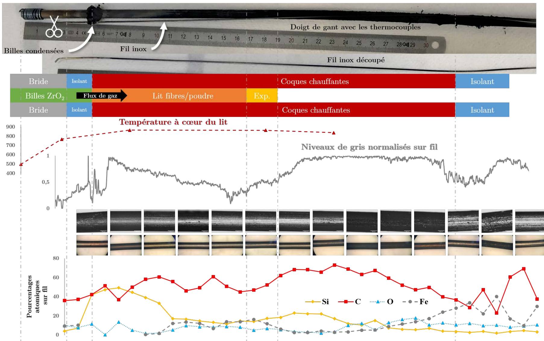
FIGURE 6.24 – Caractérisation du dépôt sur fil inox pendant une expérience de dépôt Si x C y ex-TES.
