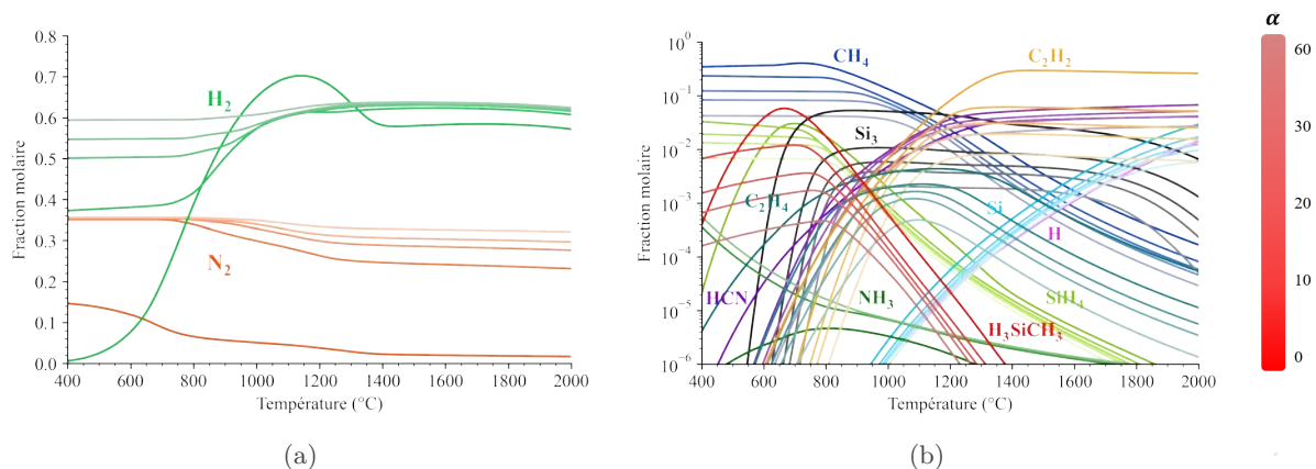
FIGURE 6.1 – Fractions molaires à l'équilibre homogène des espèces gazeuses a) H 2 et N 2 et b) CH 4 , C 2 H 2 , Si 3 , Si, H, HCN, SiH 4 et H 3 SiCH 3 pour \alpha = 0 ; 10; 20; 30 et 60.
