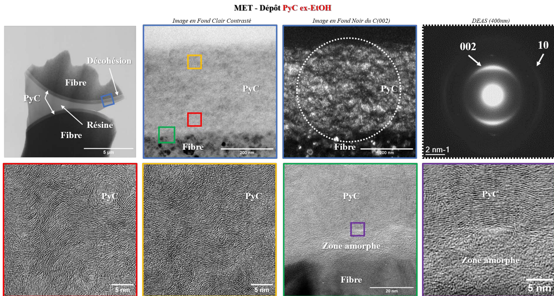
FIGURE 5.7 – Observations MET du dépôt PyC ex-EtOH épais.
