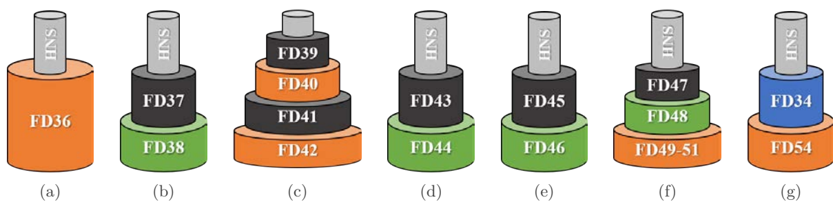
FIGURE 6.16 – Représentations schématiques des dépôts \text{PyC} , \text{Si}_x\text{C}_y , \text{Si}_y\text{N}_y et \text{BN} .
