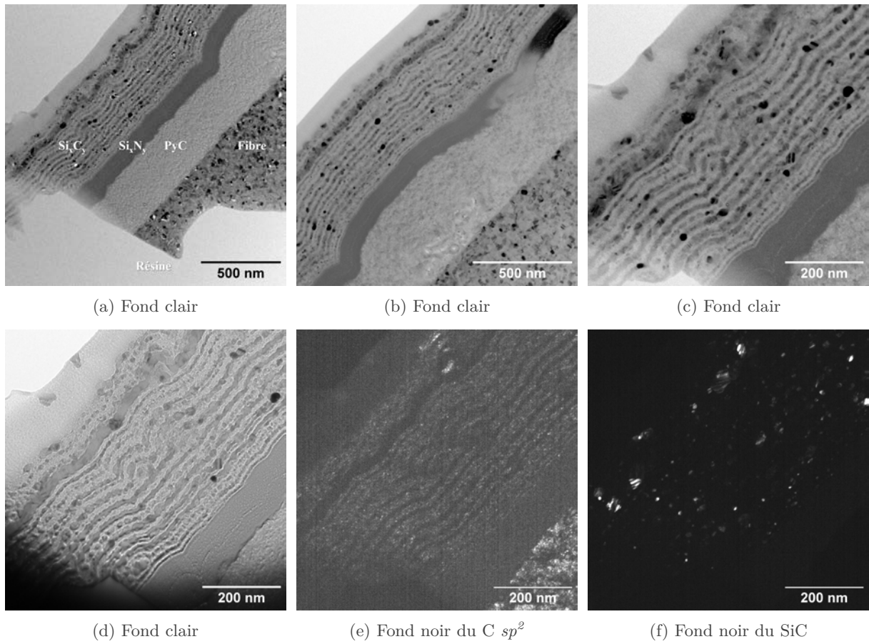
FIGURE 7.8 – Observations MET du dépôt FD47-51 (PyC/Si x N y /Si x C y ) après TTh sous azote 2h à 1450°C.
