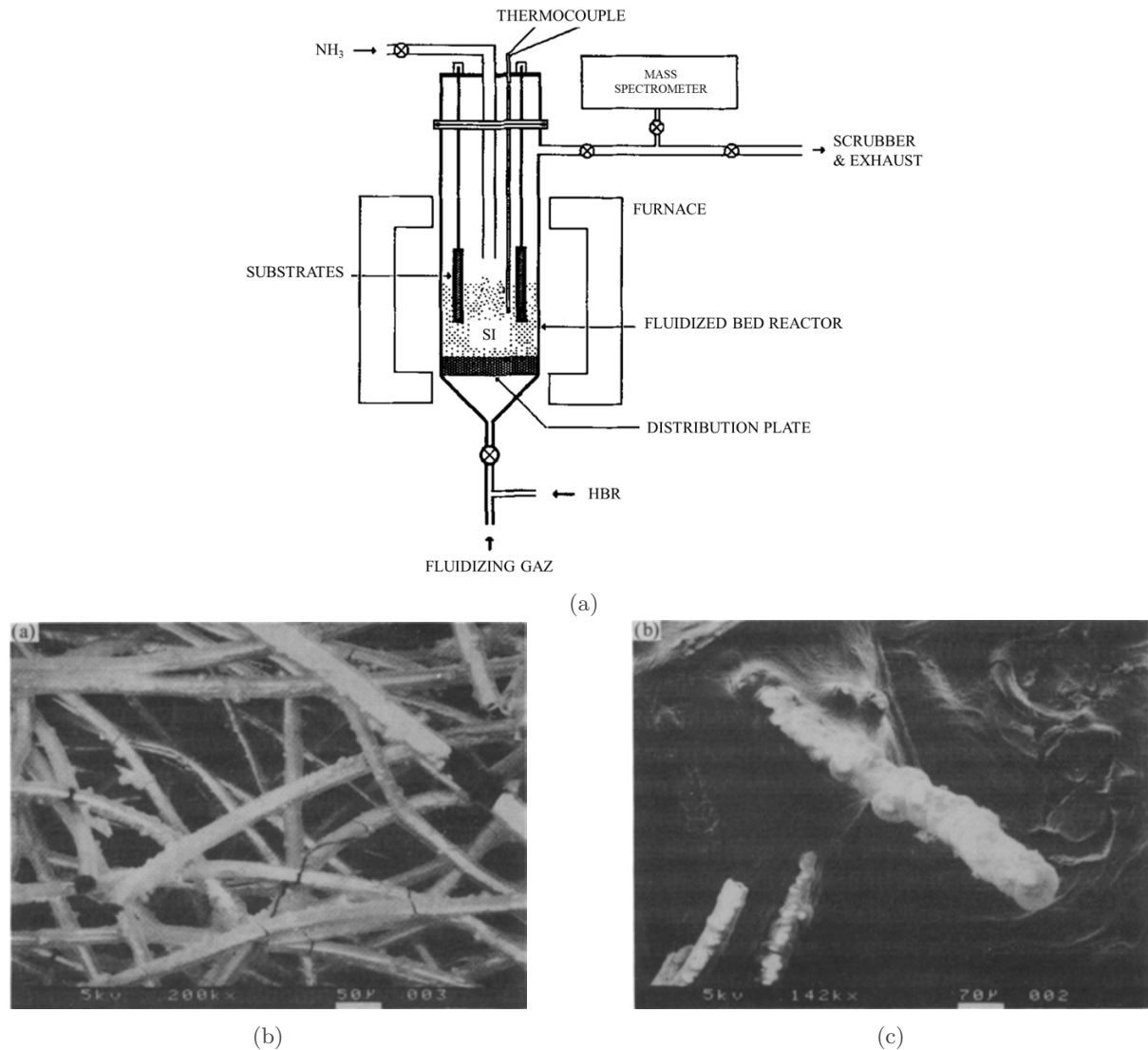
FIGURE 1.23 – a) Détail du réacteur CVD-LF à solide consommable. b) et c) Dépôt \text{Si}_3\text{N}_4 sur fibres de carbone [226].
