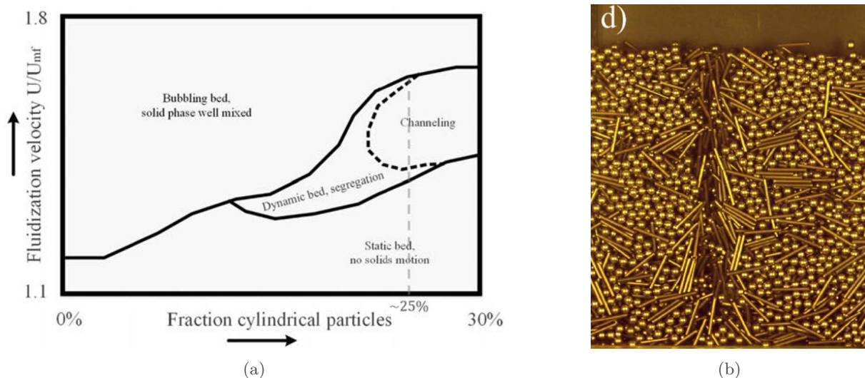
FIGURE 1.20 – a) Carte des régimes de fluidisation, montrant les effets qualitatifs de la vitesse superficielle du gaz et de la fraction de particules cylindriques sur le comportement en fluidisation et b) Images en contraste du lit fluidisé montrant le phénomène de renardage pour 30% mass. de particules cylindriques à U/U_{mf} = 1,5 . [209].
