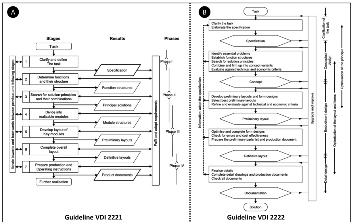
Figure-A III-6 Illustration des processus de conception systématique issus des VDI 2221 (A) et VDI 2222 (B) Tirée de Jänsch et Birkhofer (2006)
