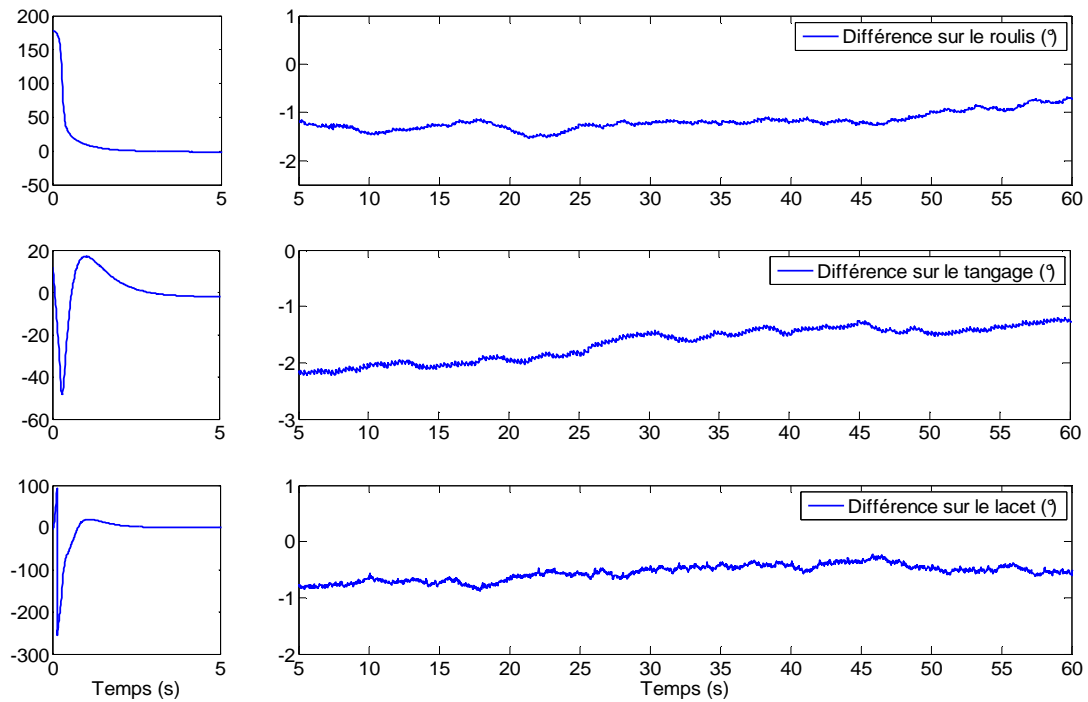
Fig. 4.4. Evolution temporelle de la différence entre les angles d'Euler estimés par l'observateur non linéaire additif et ceux calculés par la MTi-G lors d'une phase statique (avec un zoom entre 5 et 60 sec)
