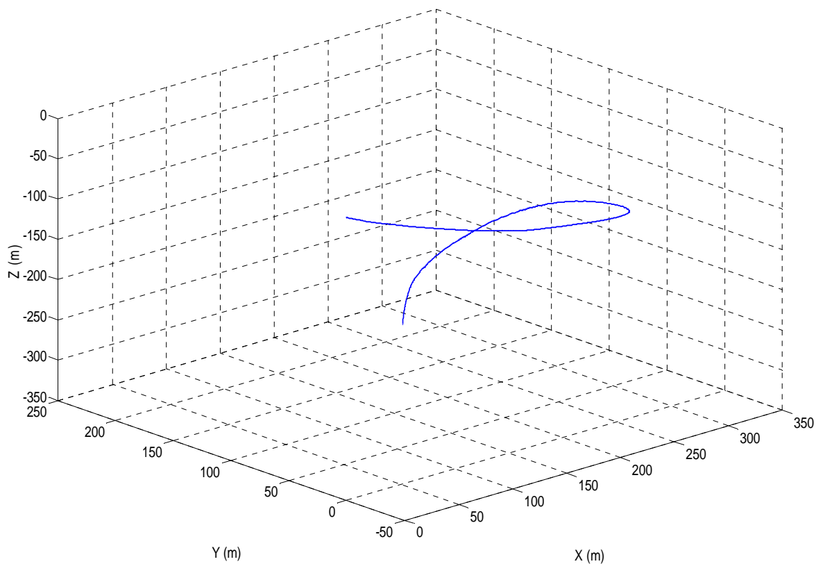
Fig. 5.6. Estimation de la position 3D au cours du déplacement en forme de rectangle au sein du CRESTIC (sans étape de recalage de la vitesse)
