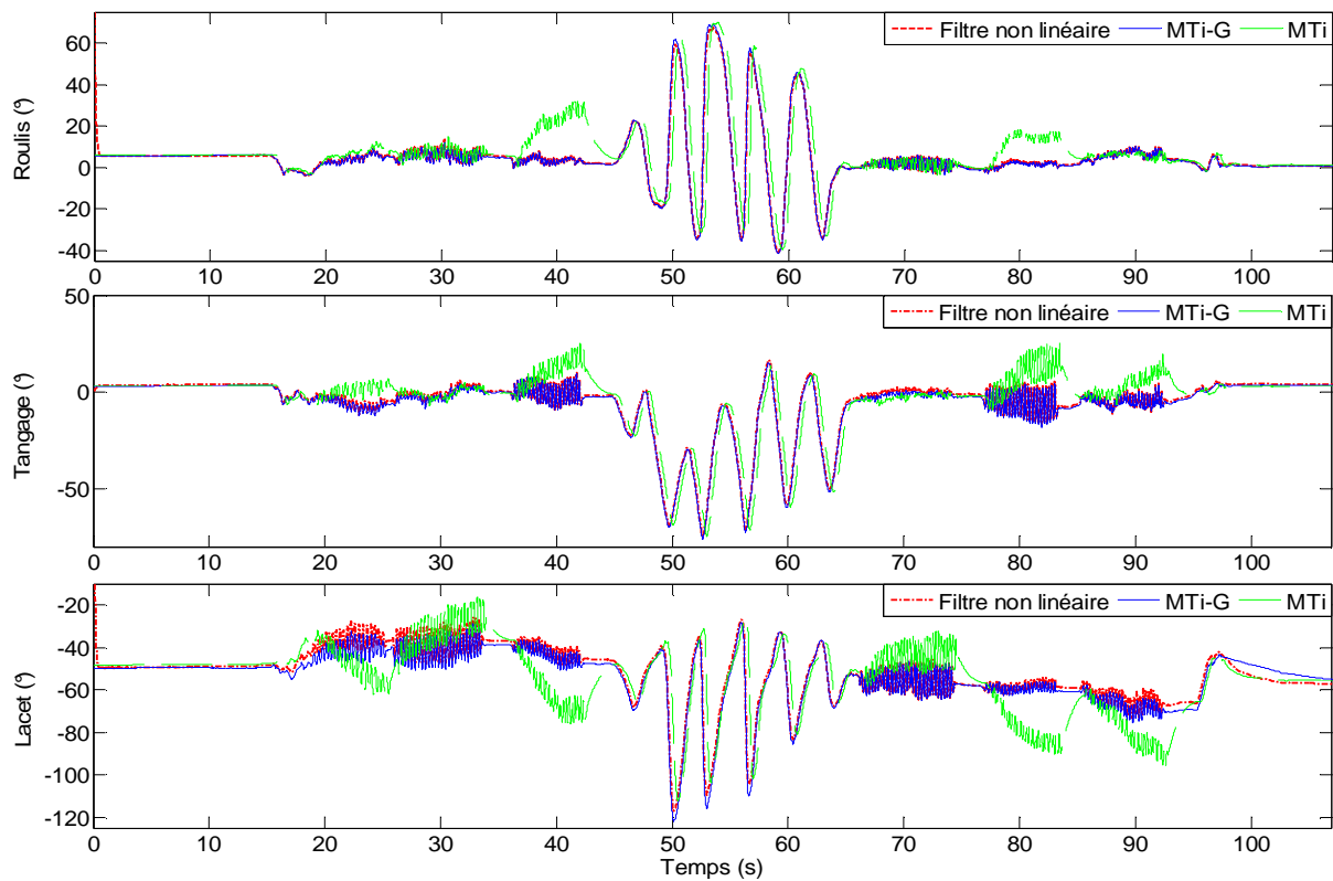
Fig. 4.35. Estimation des angles d'Euler avec le filtre complémentaire, la MTi et la MTi-G au cours du mouvement réalisé par le système complet
