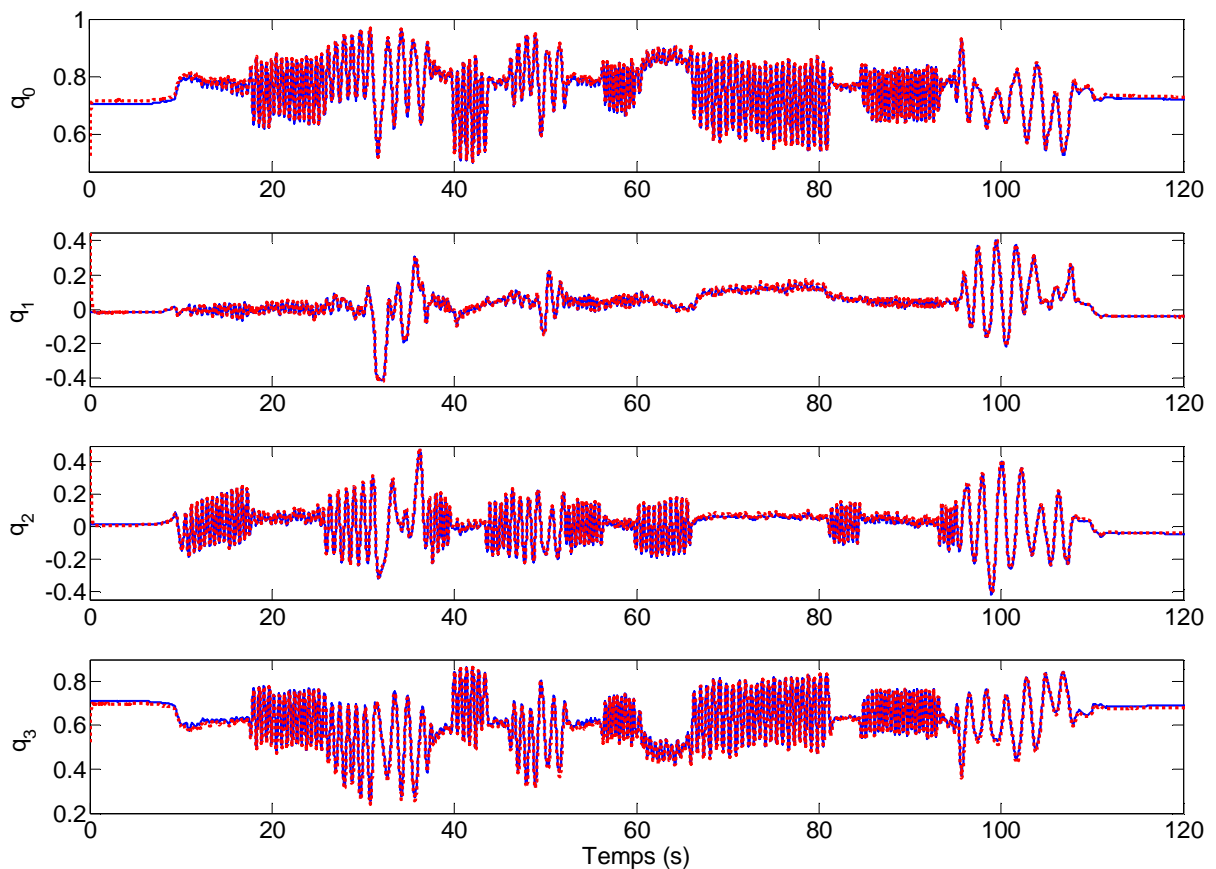
Fig. 4.13. Estimation des composantes du quaternion d'attitude au cours du mouvement réalisé par la main : q (quaternion calculé par la MTi-G (—)), \hat{q} (quaternion estimé par le filtre complémentaire (- -))
