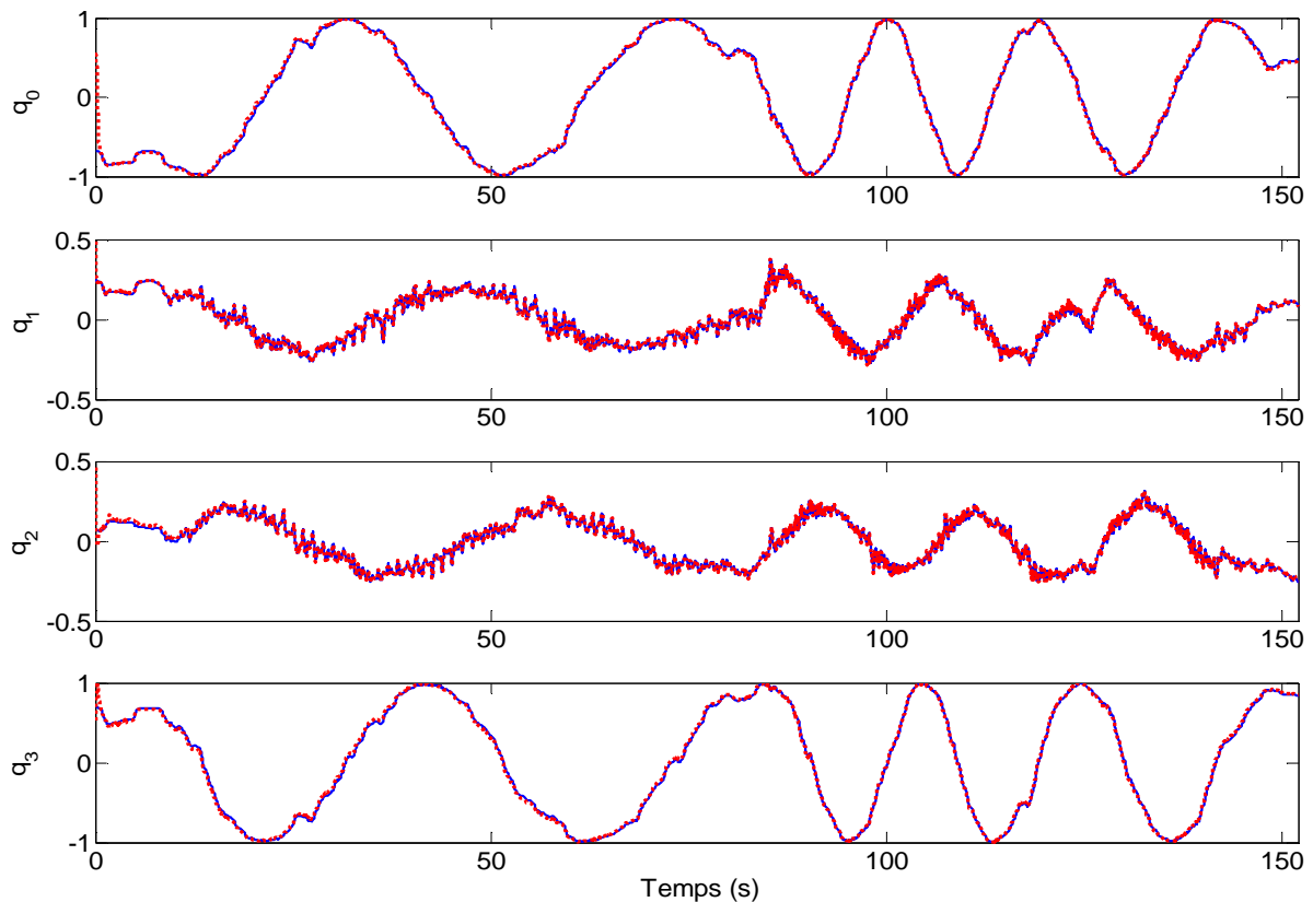
Fig. 4.28. Estimation des composantes du quaternion d'attitude au cours du mouvement réalisé par le cheval : q (quaternion calculé par la MTi-G (—)), \hat{q} (quaternion estimé par le filtre complémentaire (- -))
