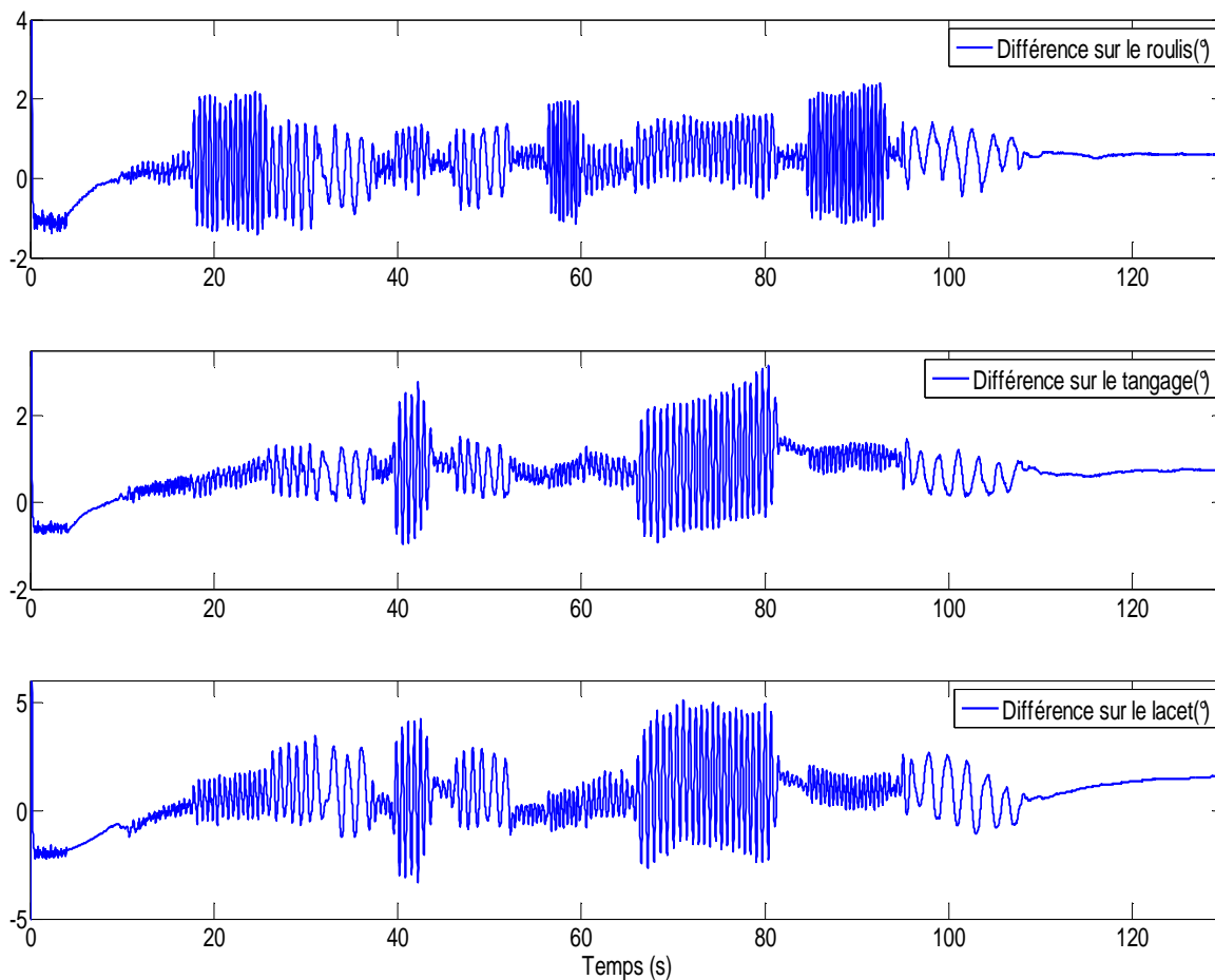
Fig. D.2. Evolution temporelle de la différence entre les angles d'Euler estimés par l'observateur à modes glissants et ceux calculés par la MTi-G au cours du mouvement réalisé par la main
