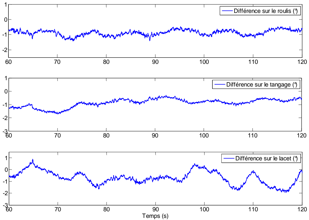
Fig. 4.7. Evolution temporelle de la différence entre les angles d'Euler estimés par l'observateur non linéaire additif et ceux calculés par la MTi-G lors d'une phase dynamique
