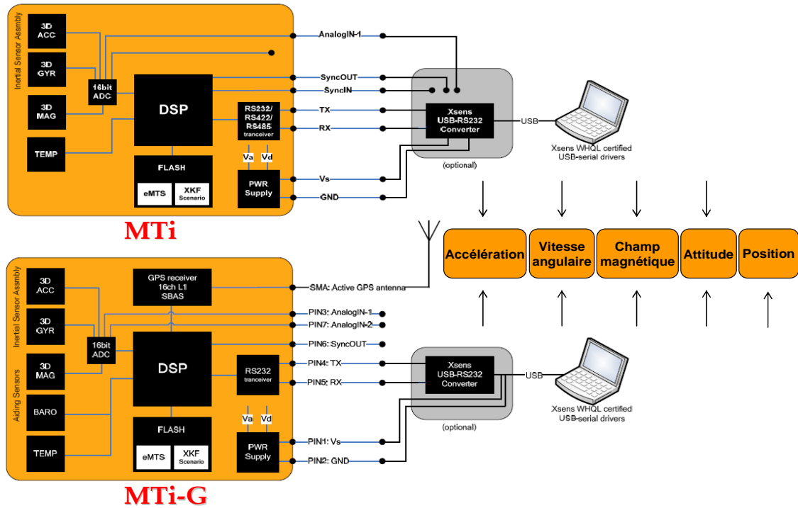
Fig. 4.2. Mécanismes de fonctionnement de la centrale d'attitude MTi et de la centrale inertielle MTi-G
