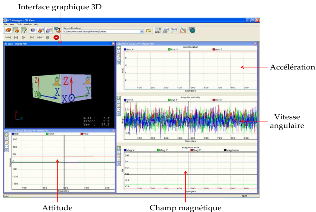
Fig. 4.3. Interface graphique du MT Manager v1.4.0
