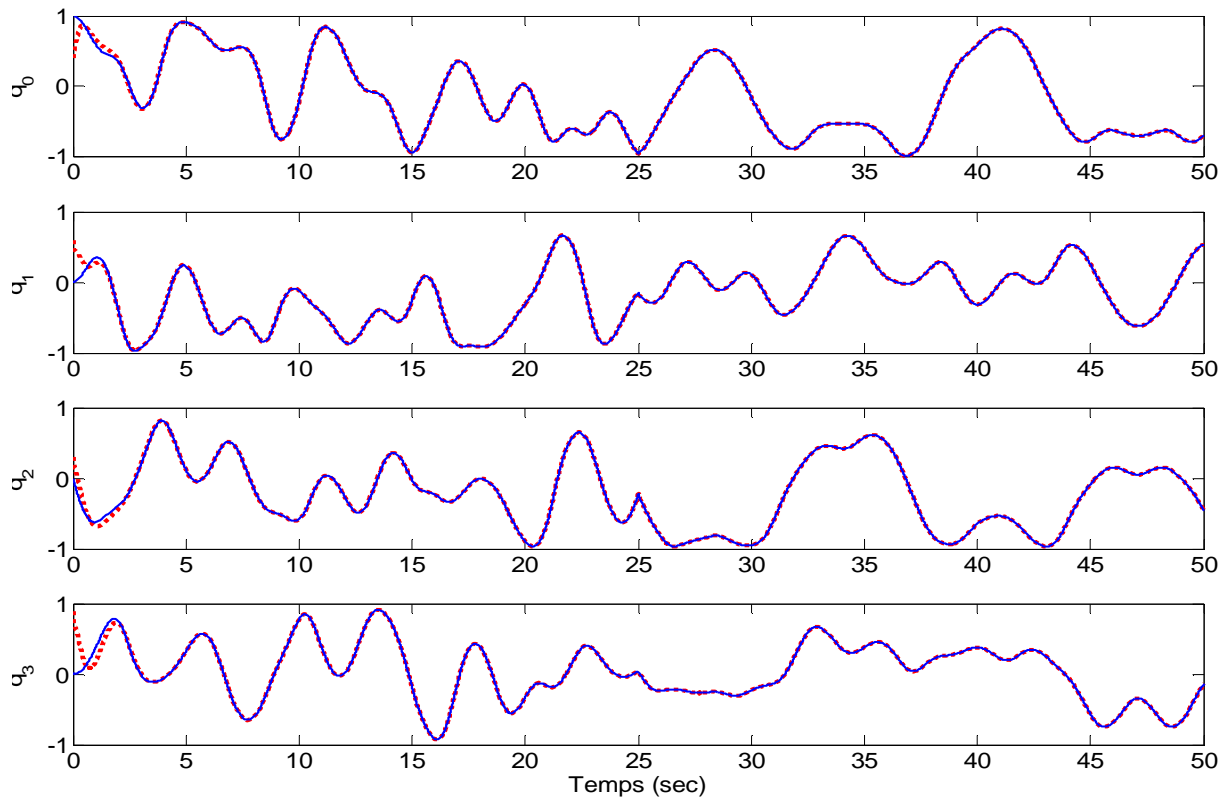
Fig. 3.3. Estimation des composantes du quaternion d'attitude par l'observateur non linéaire additif : q (modèle de référence (—)), \hat{q} (les états estimés (- -))
