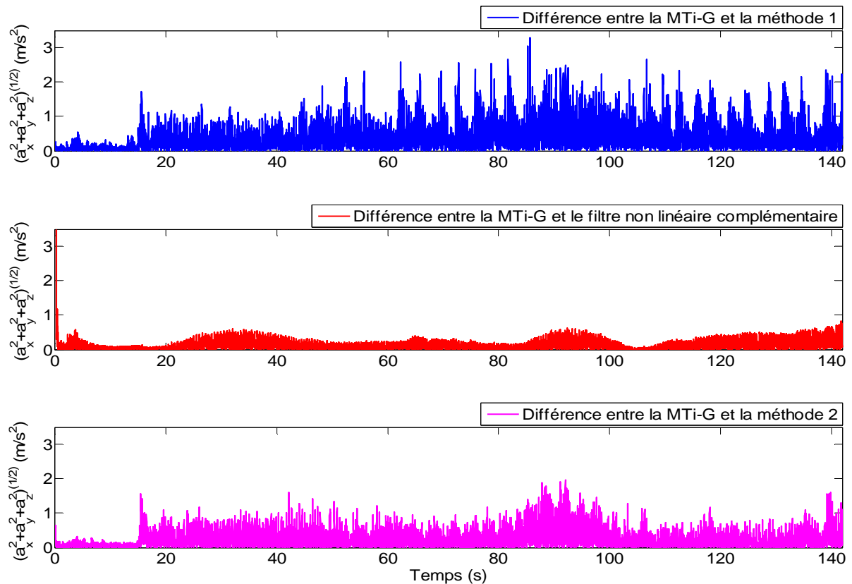
Fig. 4.38. Evolution de l'erreur d'estimation de la norme des accélérations propres du chien
