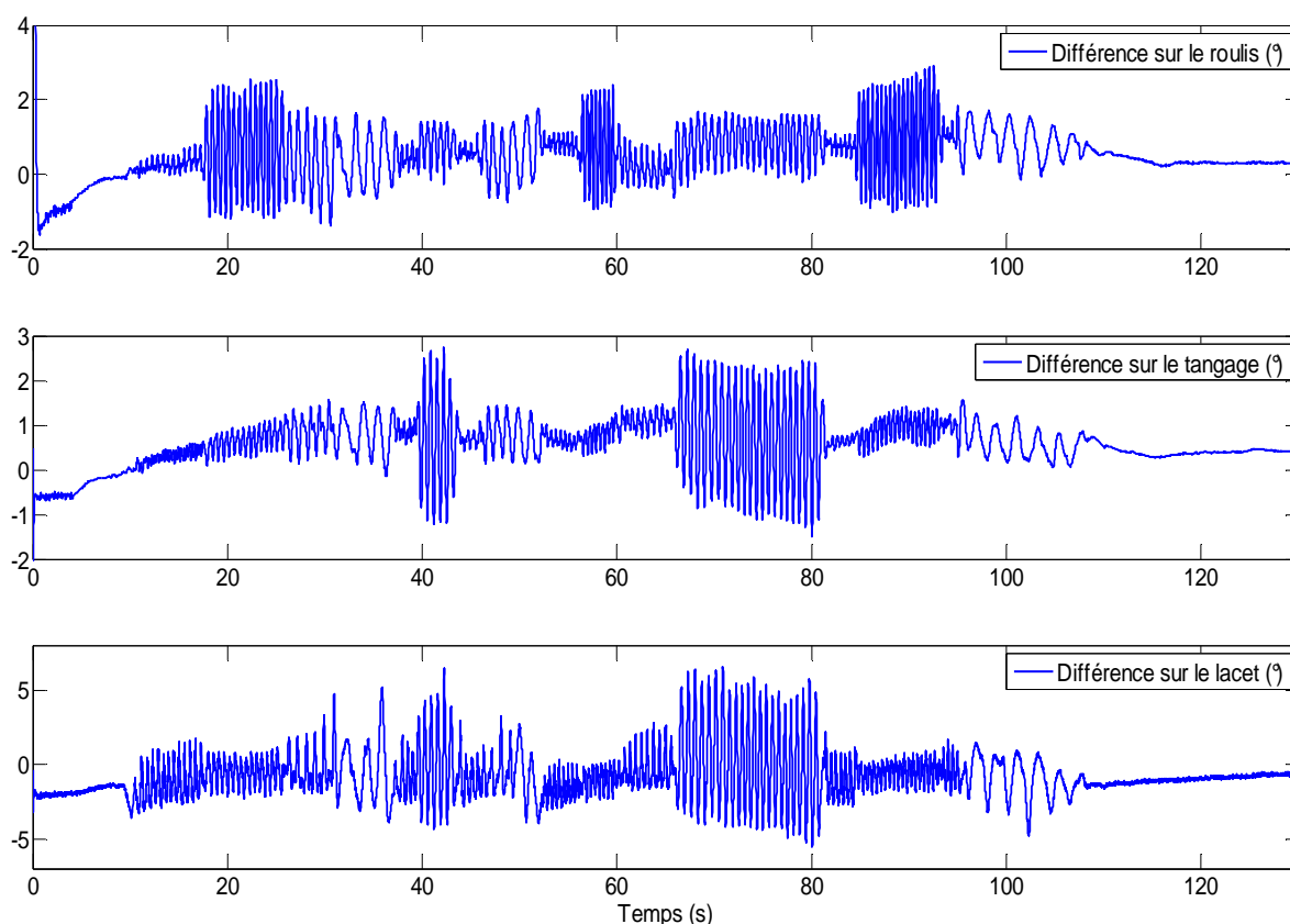
Fig. D.1. Evolution temporelle de la différence entre les angles d'Euler estimés par l'observateur non linéaire additif et ceux calculés par la MTi-G au cours du mouvement réalisé par la main
