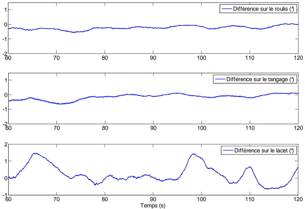
Fig. 4.8. Evolution temporelle de la différence entre les angles d'Euler estimés par l'observateur à modes glissants et ceux calculés par la MTi-G lors d'une phase dynamique
