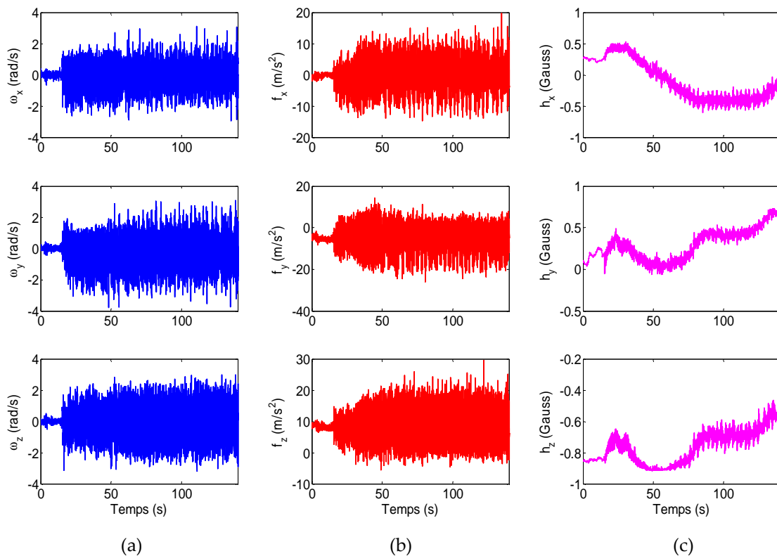
Fig. 4.19. Mesures réelles issues des capteurs de la MTi-G au cours du mouvement réalisé par le chien - (a) vitesse angulaire - (b) accélération totale - (c) champ magnétique terrestre
