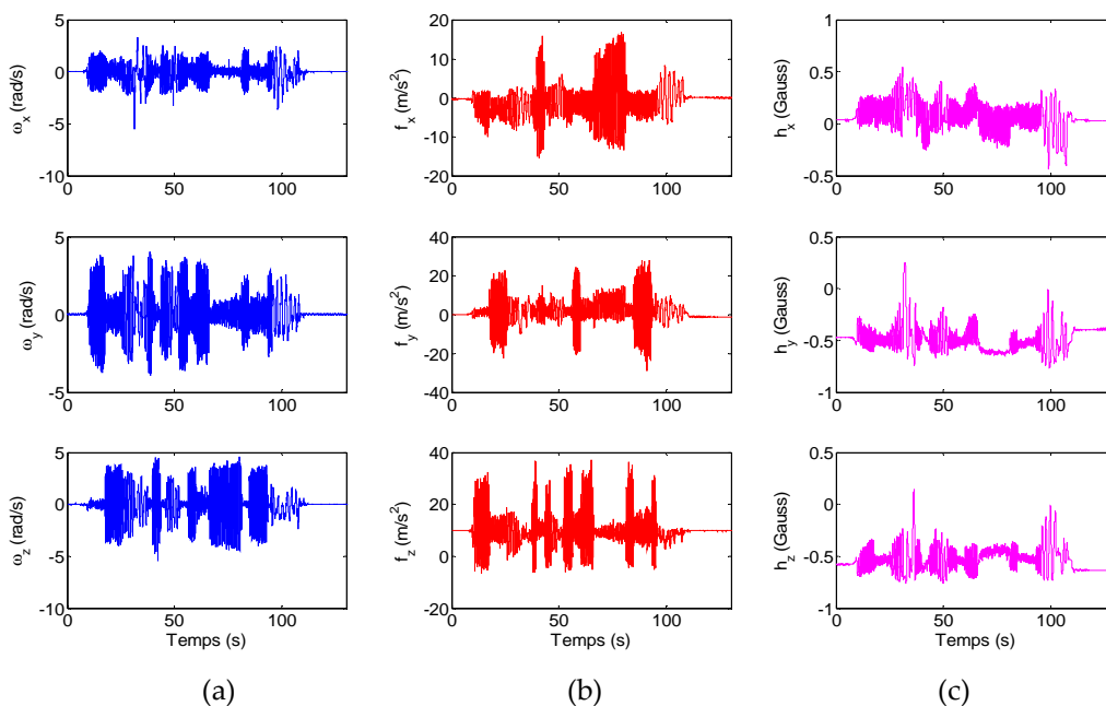
Fig. 4.12. Mesures réelles issues des capteurs au cours du mouvement de la main - (a) vitesse angulaire - (b) accélération totale - (c) champ magnétique terrestre
