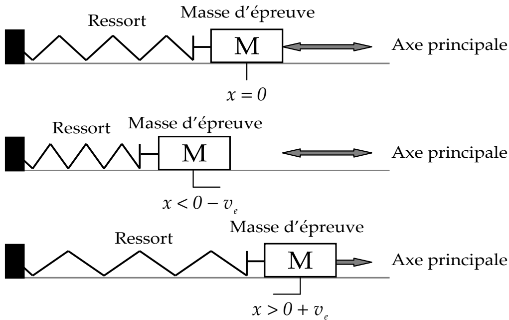
Fig. 1.7. Principe de fonctionnement d'un accéléromètre
