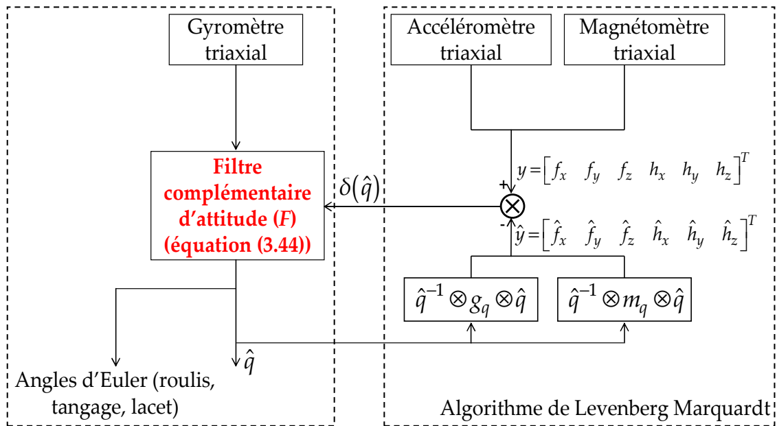
Fig. 3.10. Schéma bloc du filtre complémentaire de l'attitude
