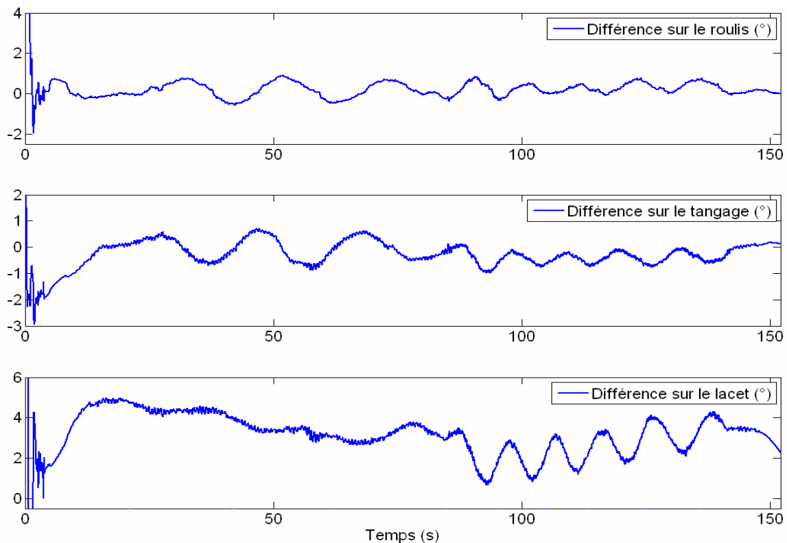
Fig. 4.31. Evolution temporelle de la différence entre les angles d'Euler estimés par le filtre complémentaire et ceux calculés par la MTi-G au cours du mouvement réalisé par le cheval
