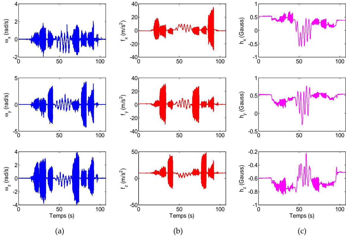
Fig. 4.34. Mesures réelles issues des capteurs de la MTi au cours du mouvement du système complet - (a) vitesse angulaire - (b) force spécifique - (c) champ magnétique terrestre
