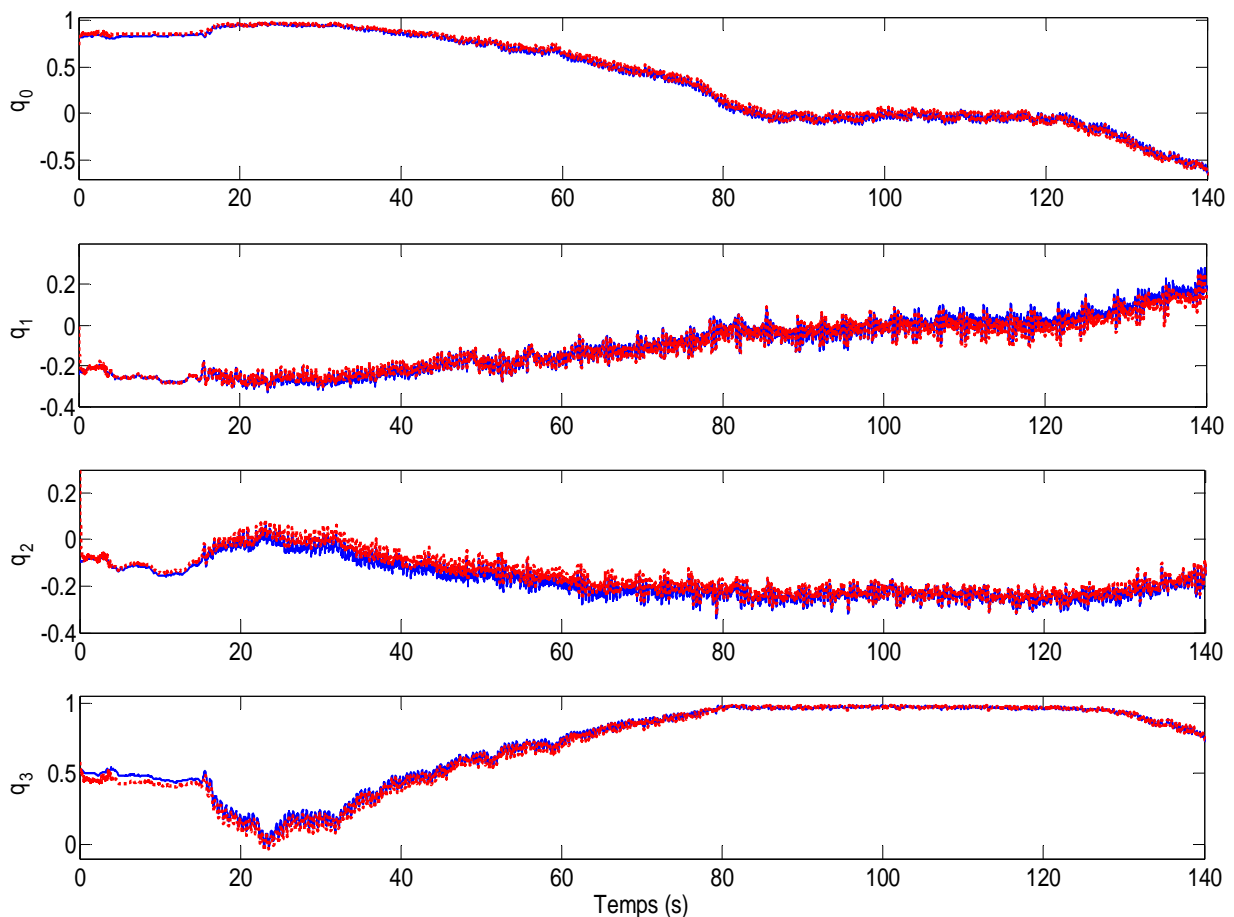
Fig. 4.20. Estimation des composantes du quaternion d'attitude au cours du mouvement réalisé par le chien : q (quaternion calculé par la MTi-G en ligne solide (—)), \hat{q} (quaternion estimé par le filtre complémentaire (- -))
