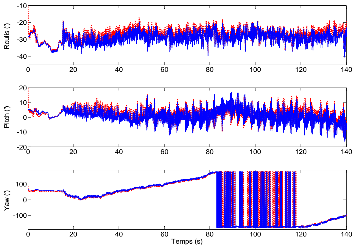
Fig. 4.22. Estimation des angles d'Euler au cours du mouvement réalisé par le chien : (\phi, \theta, \psi) : angles d'Euler calculés par la MTi-G (—), (\hat{\phi}, \hat{\theta}, \hat{\psi}) : angles d'Euler estimés par le filtre complémentaire (---)
