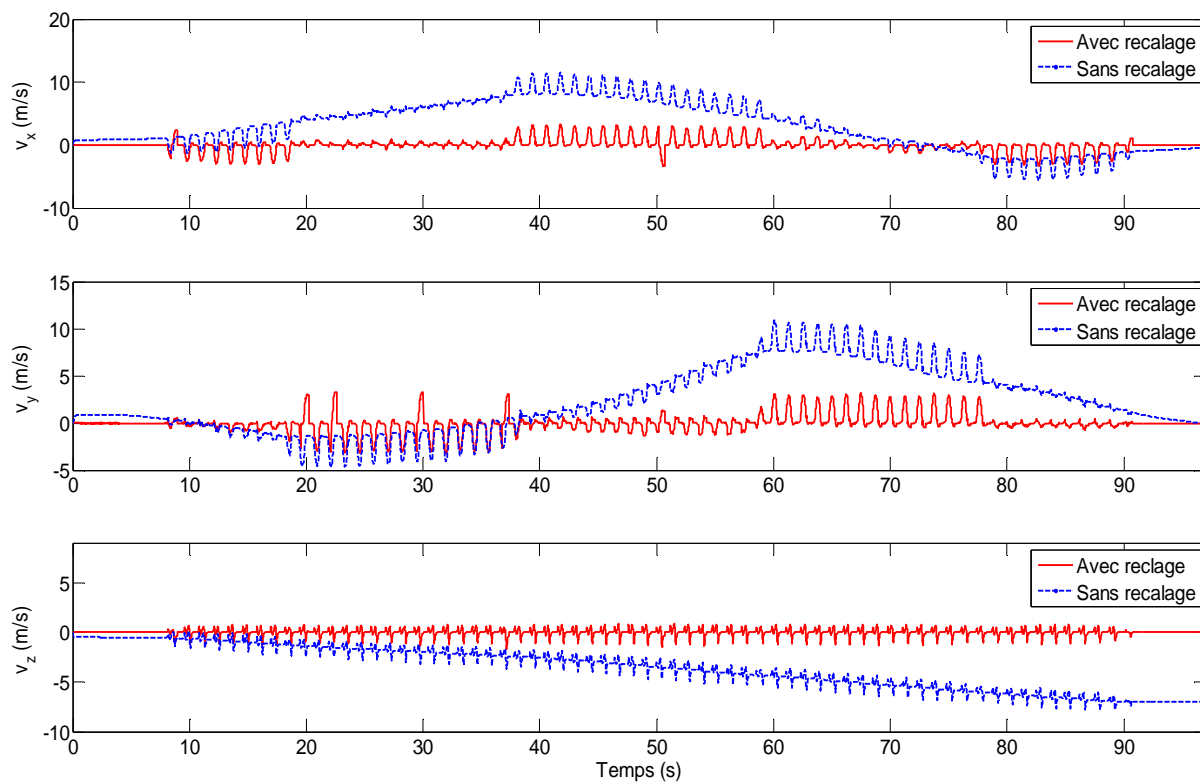
Fig. 5.5. Estimation de la vitesse linéaire \hat{v} avec et sans étape de recalage (remise à zéro)
