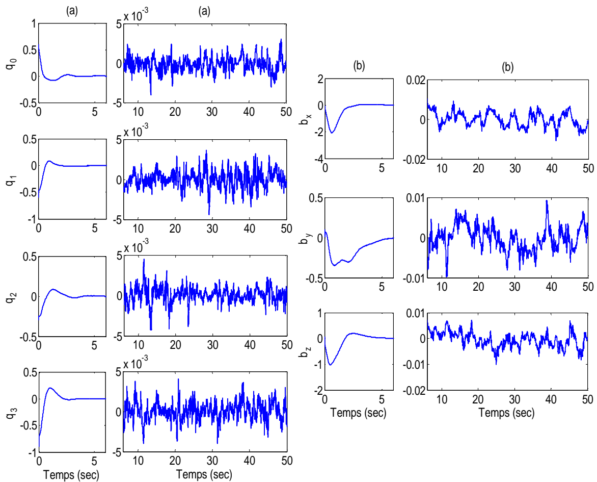
Fig. 3.5. (a) Erreurs d'estimation sur les composantes du quaternion obtenues avec l'observateur non linéaire additif (avec un zoom entre 6 et 50 sec) - (b) Erreurs d'estimation sur les composantes du biais obtenues avec l'observateur non linéaire additif (avec un zoom entre 6 et 50 sec)
