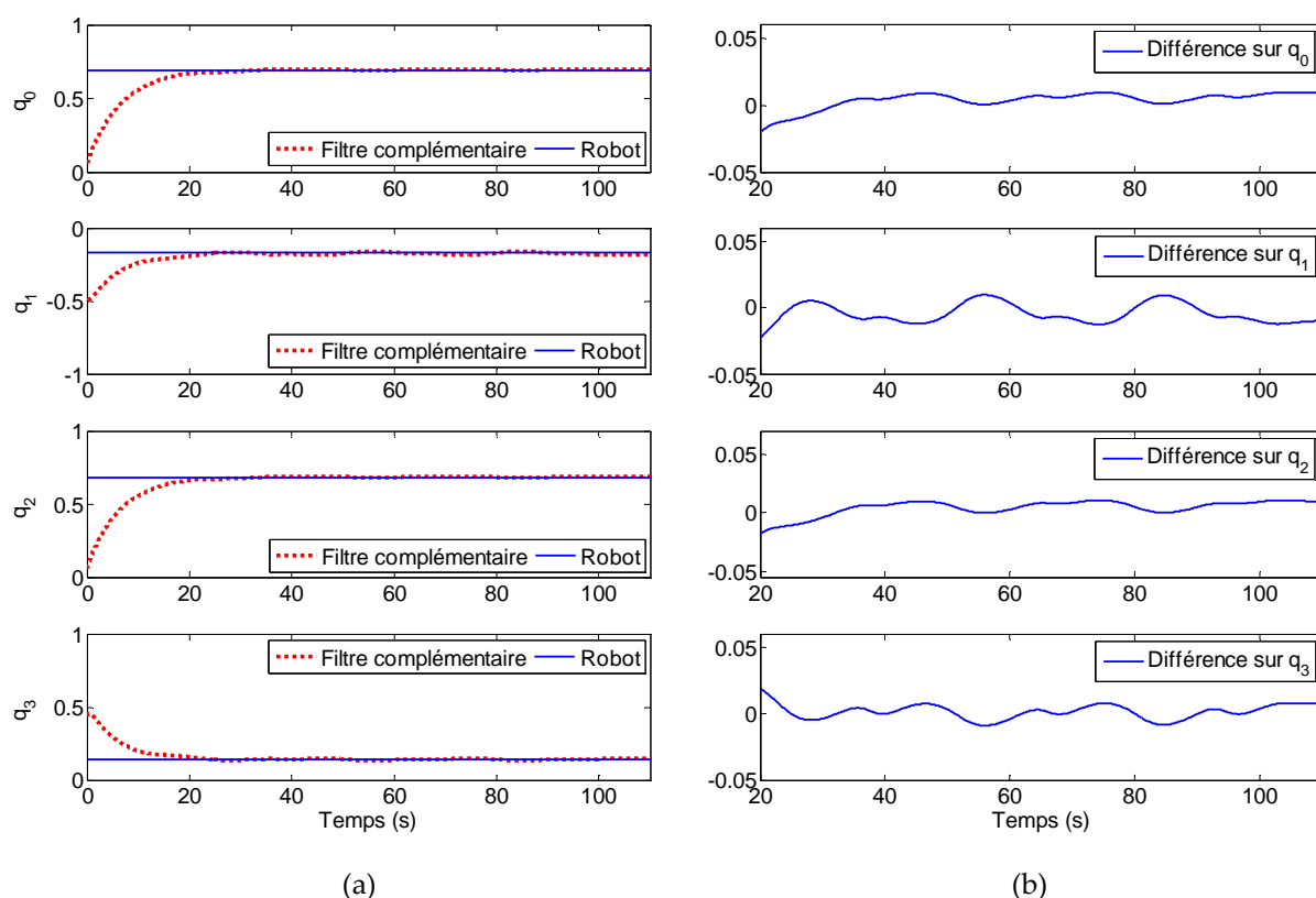
Fig. E.2. (a) Estimation des composantes du quaternion d'attitude au cours du mouvement réalisé par la tête du robot : q (quaternion calculé par le robot (—)), \hat{q} (quaternion estimé par le filtre complémentaire (- -)) - (b) Erreur entre le quaternion estimé par le filtre complémentaire et celui calculé par le robot
