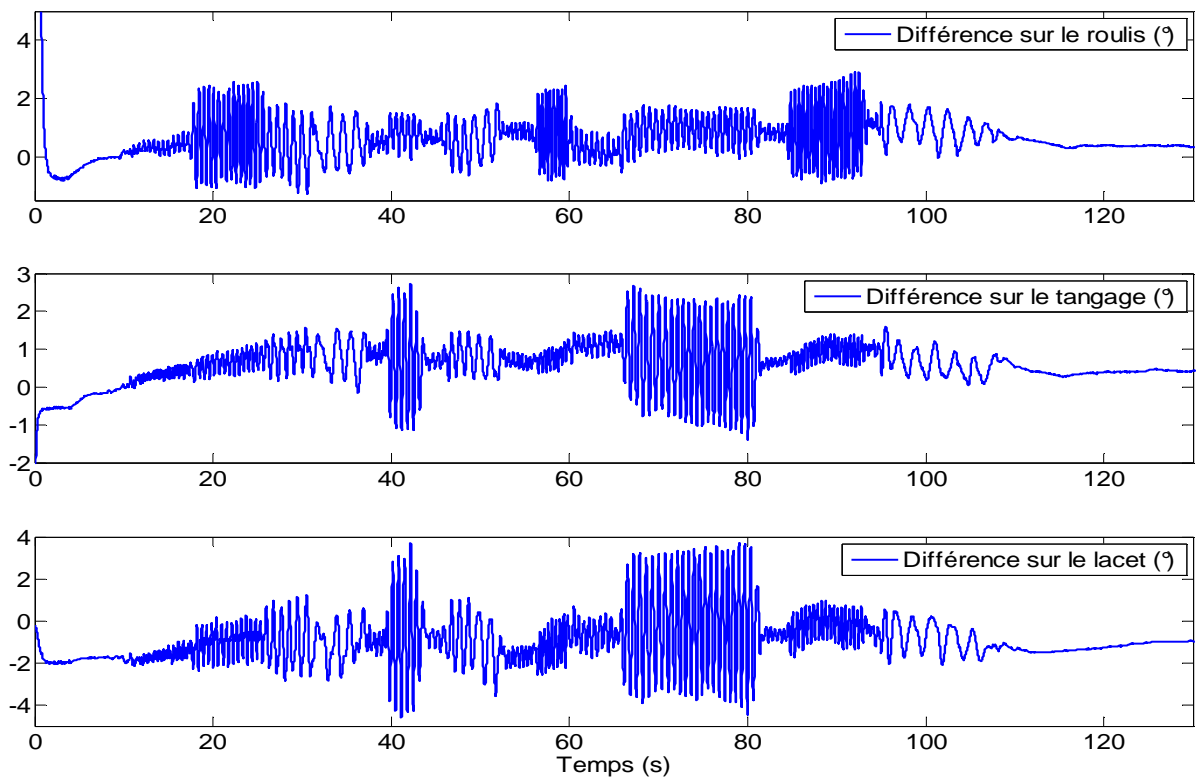
Fig. 4.16. Evolution temporelle de la différence entre les angles d'Euler estimés par le filtre complémentaire et ceux calculés par la MTi-G au cours du mouvement réalisé par la main
