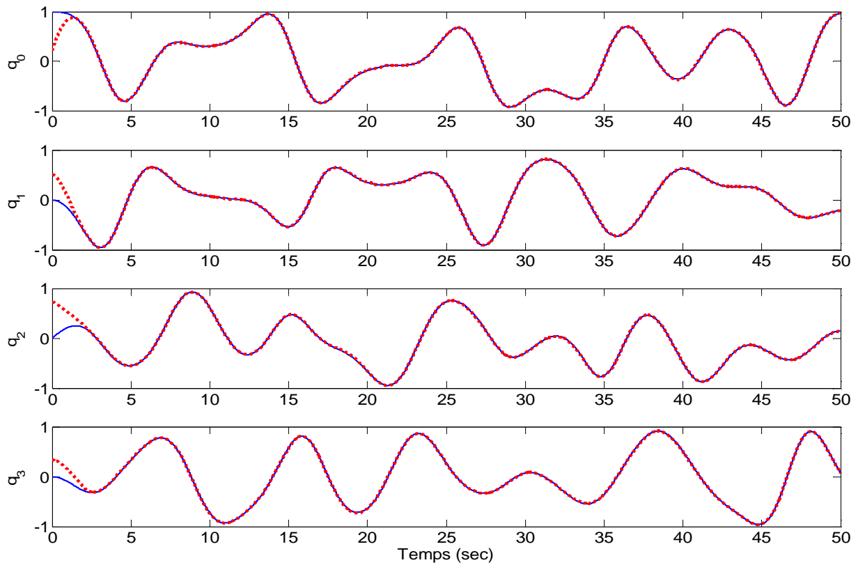
Fig. 3.8. Estimation des composantes du quaternion d'attitude par l'observateur à modes glissants: q (modèle de référence (—)), \hat{q} (les états estimés (- -))
