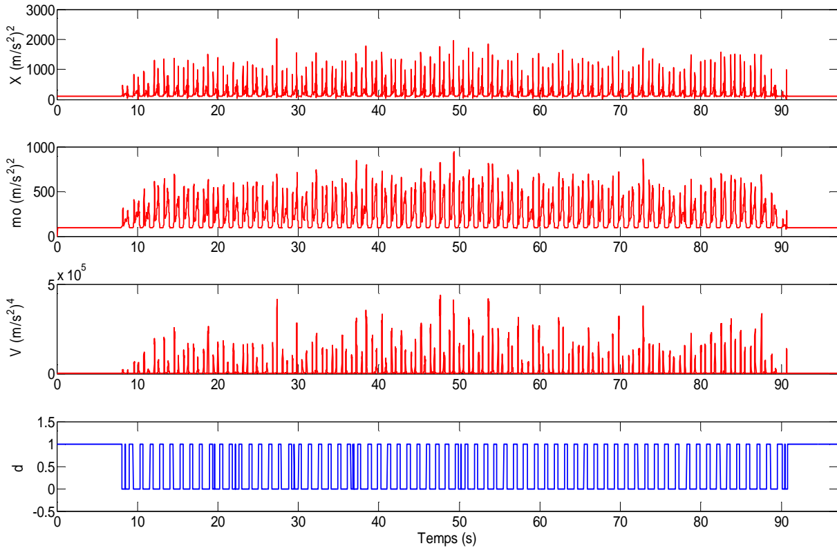
Fig. 5.4. La norme carrée de l'accélération totale \chi_i , la moyenne mo_j , la variance V_e(j) et les instants de détection du pas (détecteur)
