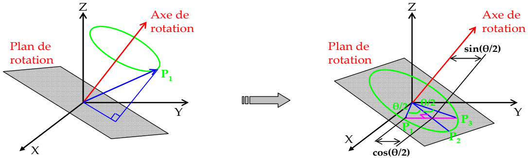
Fig. 1.4. Représentation graphique d'un quaternion unitaire
