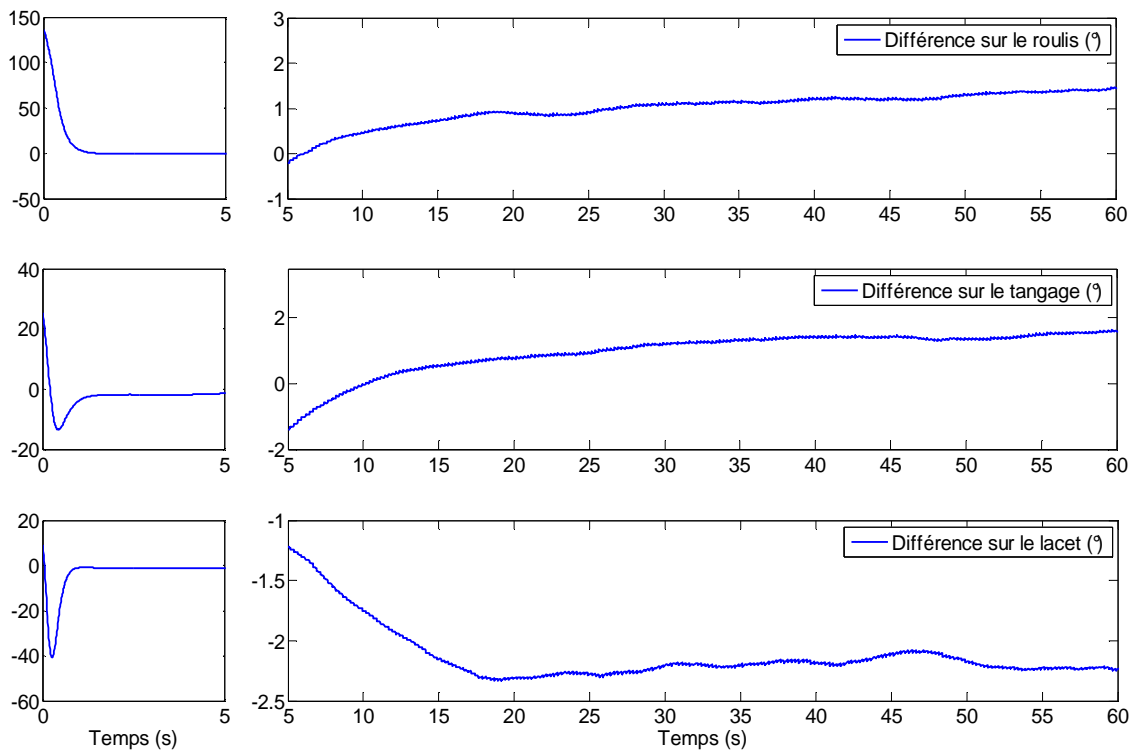
Fig. 4.6. Evolution temporelle de la différence entre les angles d'Euler estimés par le filtre complémentaire et ceux calculés par la MTi-G lors d'une phase statique (avec un zoom entre 5 et 60 sec)
