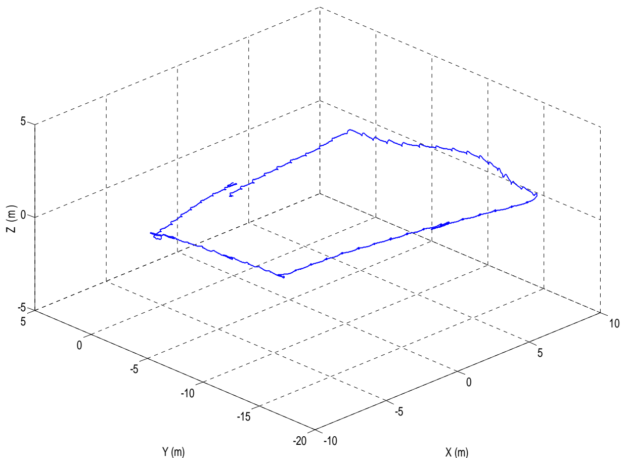
Fig. 5.7. Estimation de la position 3D au cours du déplacement en forme de rectangle au sein du CReSTIC (avec étape de recalage de la vitesse)
