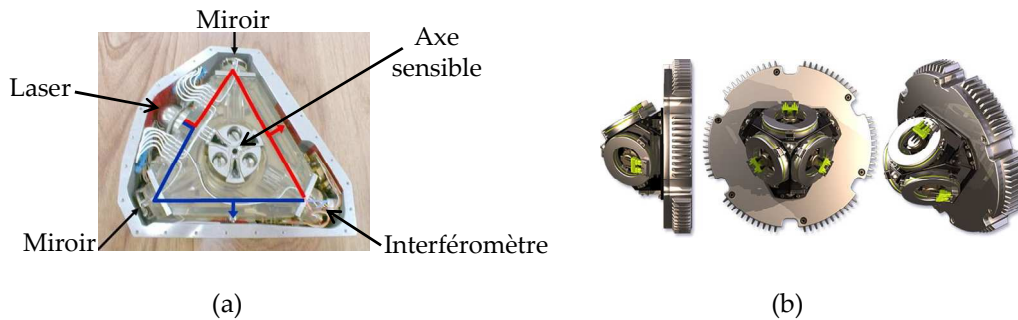
Fig. 1.14. Gyromètre - (a) laser - (b) à fibre optique
