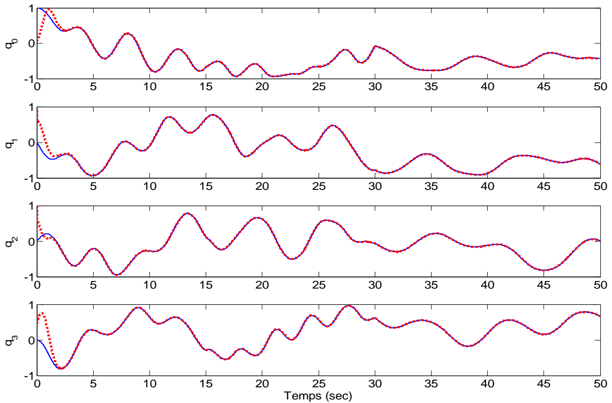
Fig. 3.13. Estimation des composantes du quaternion d'attitude par le filtre complémentaire : q (modèle de référence (—)), \hat{q} (les états estimés (- -))
