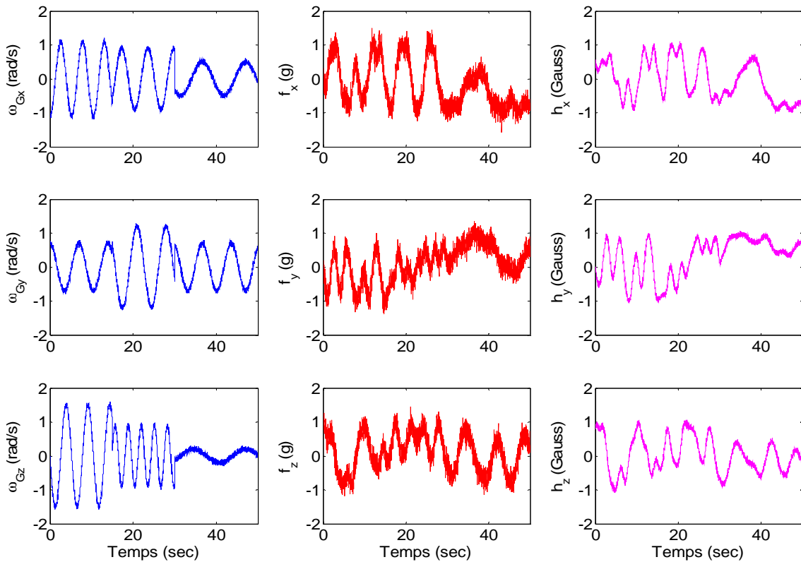
Fig. 3.12. Mesures simulées issues des capteurs - (a) vitesse angulaire - (b) accélération totale - (c) champ magnétique terrestre
