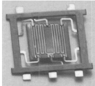
Fig. 1.12. Magnétomètre à effet magnétorésistif
