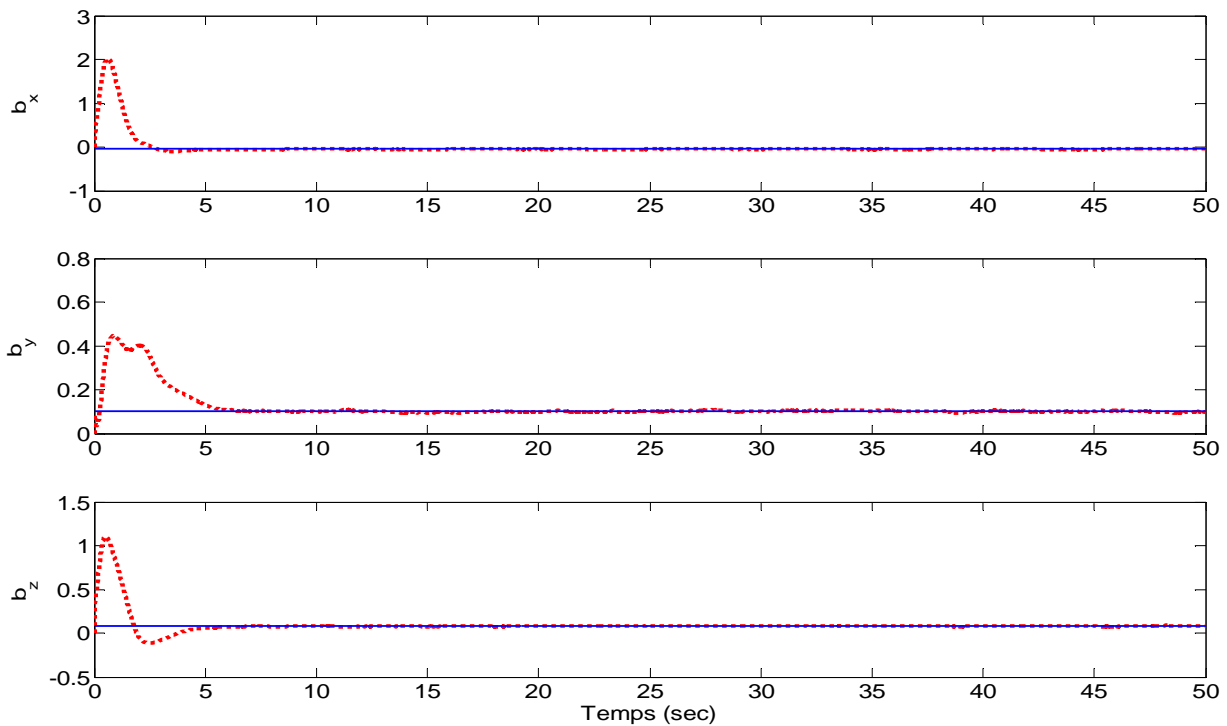
Fig. 3.4. Estimation des composantes du biais dans le gyromètre par l'observateur non linéaire additif : b (modèle de référence (—)), \hat{b} (les états estimés (- -))
