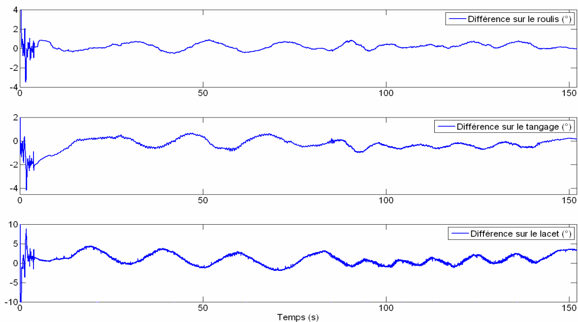
Fig. D.5. Evolution temporelle de la différence entre les angles d'Euler estimés par l'observateur non linéaire additif et ceux calculés par la MTi-G au cours du mouvement réalisé par le cheval
