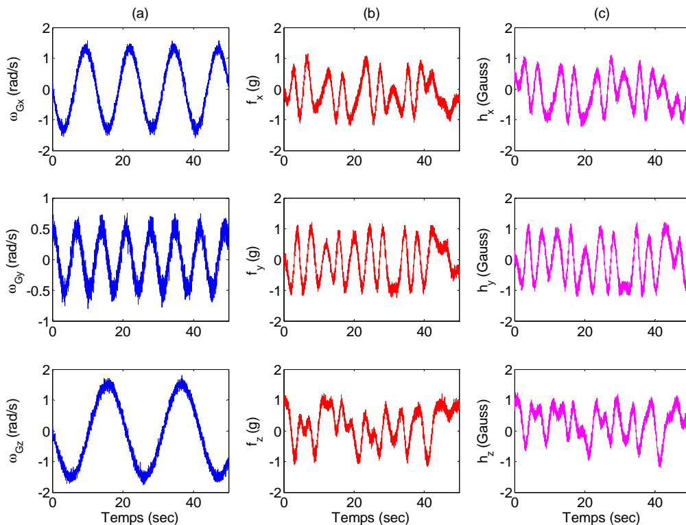
Fig. 3.7. Mesures simulées issues des capteurs - (a) vitesse angulaire - (b) accélération totale - (c) champ magnétique terrestre
