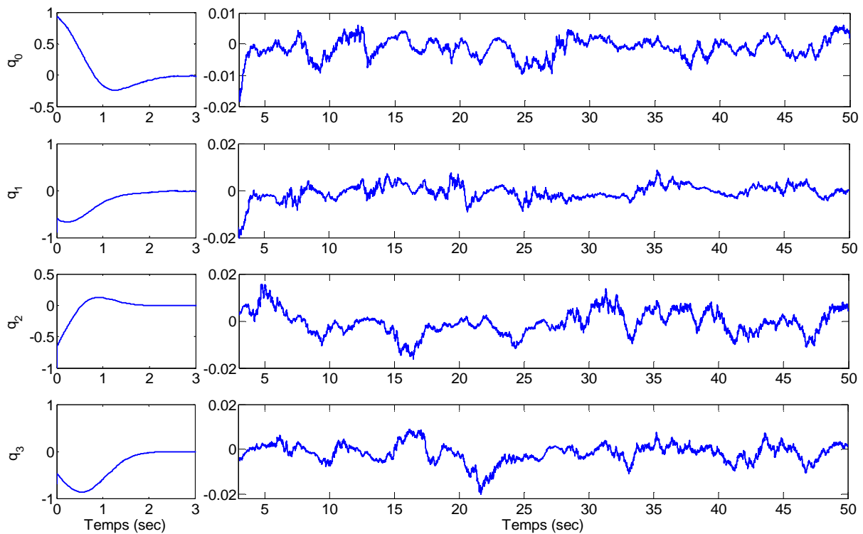
Fig. 3.14. Erreurs d'estimation sur les quatre composantes du quaternion obtenues avec le filtre complémentaire (avec un zoom entre 3 et 50 sec)
