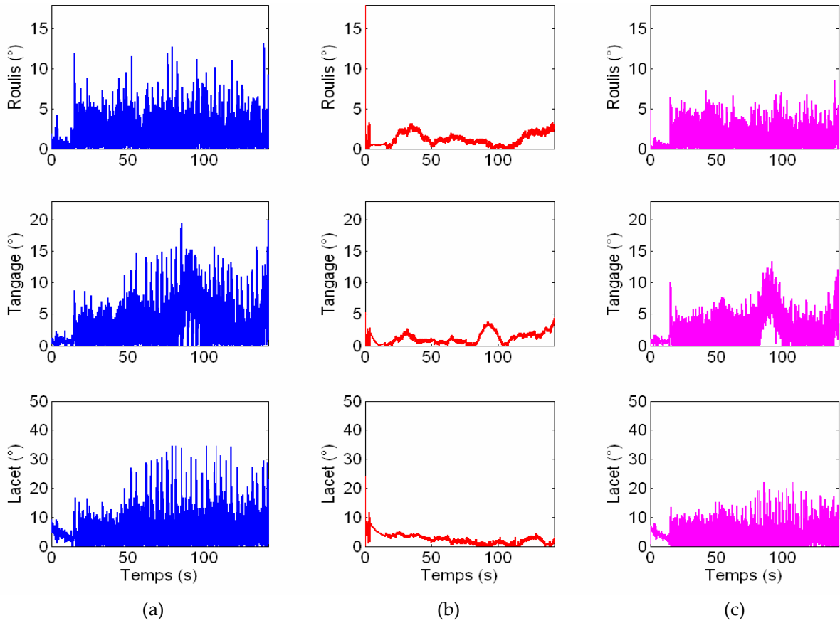
Fig. 4.37. Evolution de l'erreur d'estimation des angles d'Euler au cours du mouvement réalisé par le chien - (a) différence entre la MTi-G et la méthode_1 - (b) différence entre la MTi-G et le filtre complémentaire - (c) différence entre la MTi-G et la méthode_2
