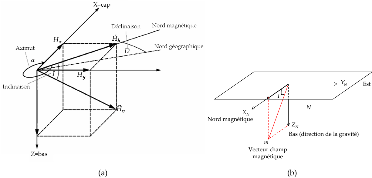
Fig. 1.11. (a) Représentation réelle du vecteur magnétique terrestre - (b) Représentation approchée du champ magnétique terrestre dans le système de coordonnées NED N(X_N, Y_N, Z_N)
