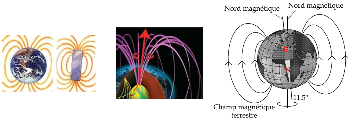
Fig. 1.10. Représentation des lignes du champ magnétique terrestre
