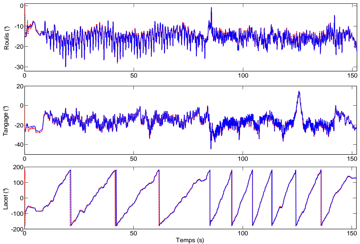
Fig. 4.30. Estimation des angles d'Euler au cours du mouvement réalisé par le cheval : (\phi, \theta, \psi) : angles d'Euler calculés par la MTi-G (—), (\hat{\phi}, \hat{\theta}, \hat{\psi}) : angles d'Euler estimés par le filtre complémentaire (- -)
