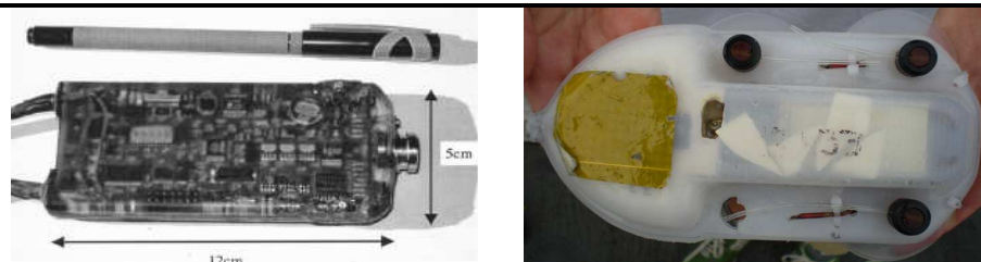
Fig. B.4. Le bio-logger DTAG
