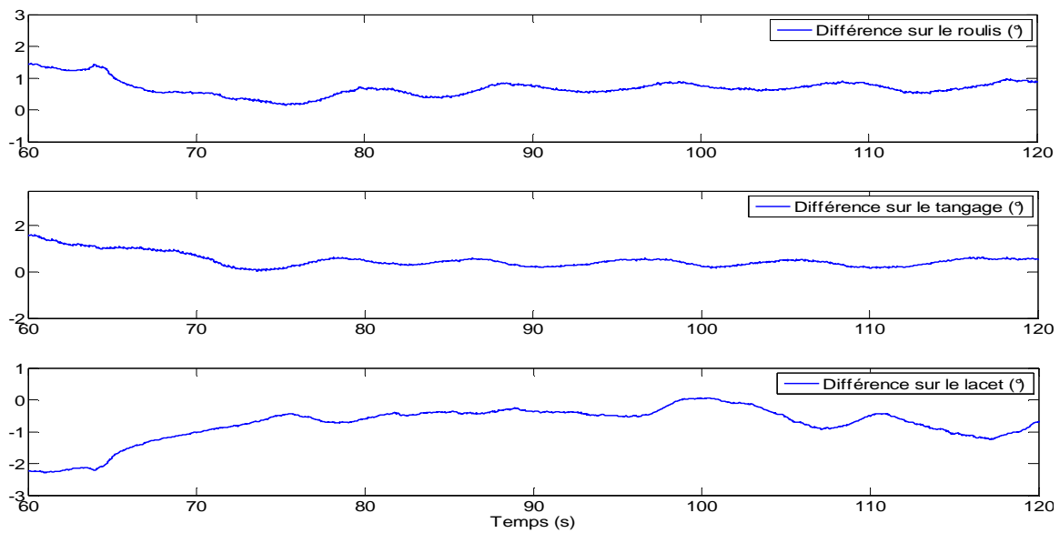
Fig. 4.9. Evolution temporelle de la différence entre les angles d'Euler estimés par le filtre complémentaire et ceux calculés par la MTi-G lors d'une phase dynamique
