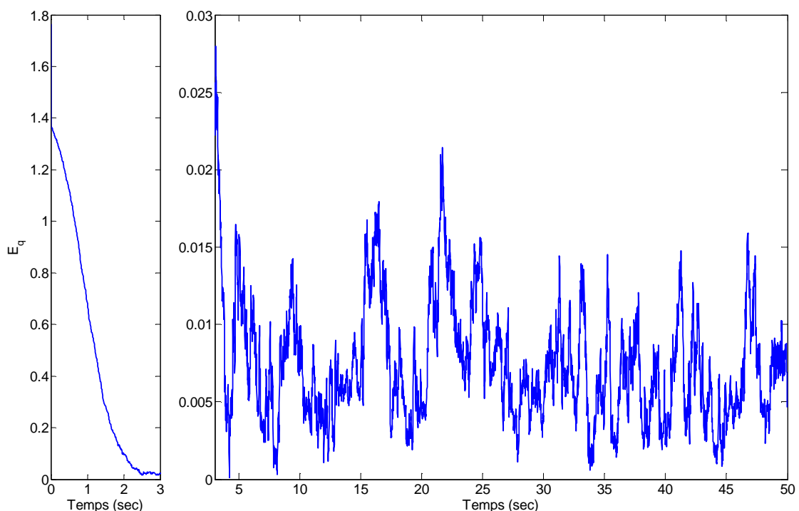
Fig. 3.15. Erreur d'estimation E_q = \|(q^{-1} \otimes \hat{q}) - 1\| sur le quaternion obtenue avec le filtre complémentaire (avec un zoom entre 3 et 50 sec)
