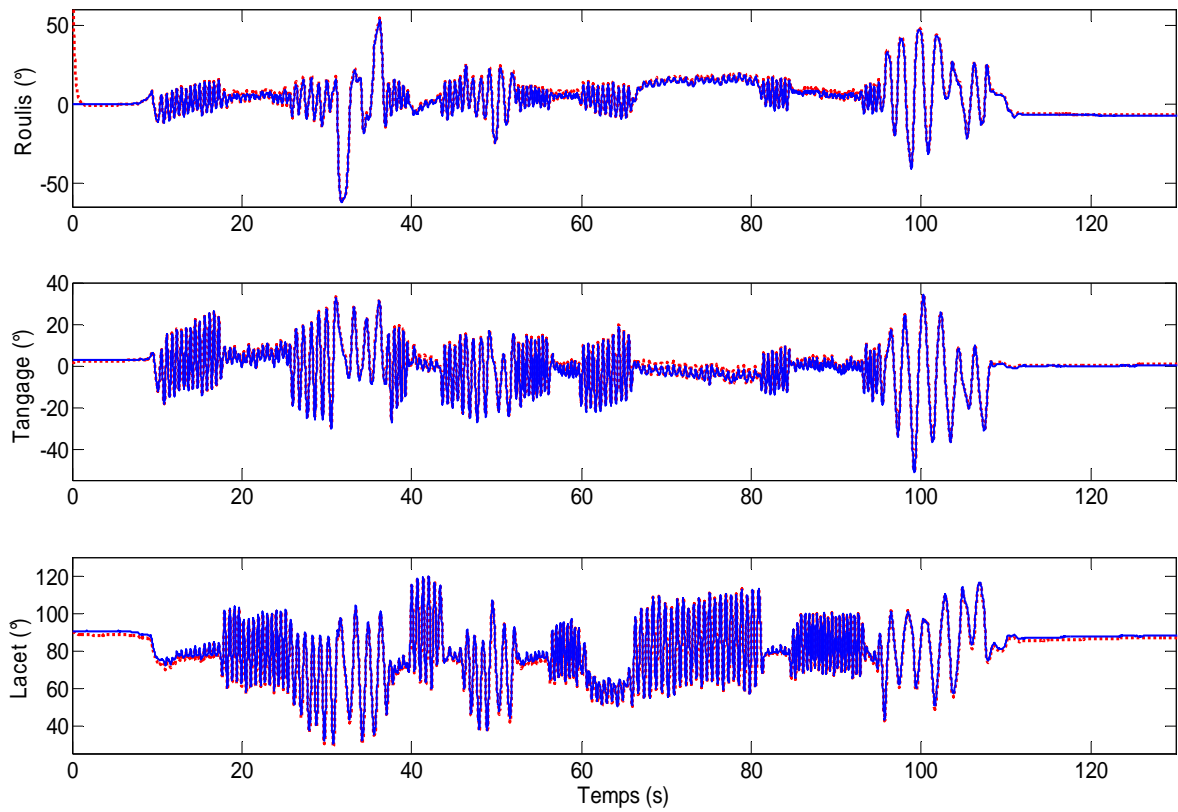
Fig. 4.15. Estimation des angles d'Euler au cours du mouvement réalisé par la main : (\phi, \theta, \psi) : angles d'Euler calculés par la MTi-G (—), (\hat{\phi}, \hat{\theta}, \hat{\psi}) : angles d'Euler estimés par le filtre complémentaire (- -)
