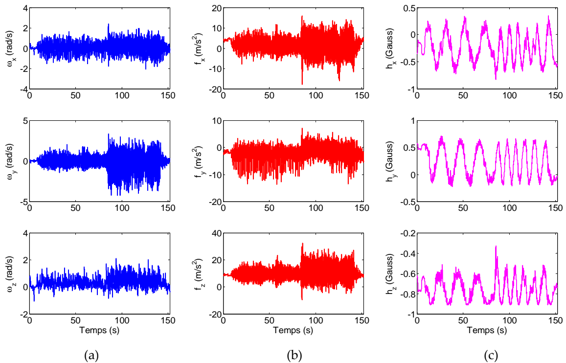
Fig. 4.27. Mesures réelles issues des capteurs de la MTi-G au cours du mouvement réalisé par le cheval - (a) vitesse angulaire - (b) force spécifique - (c) champ magnétique terrestre
