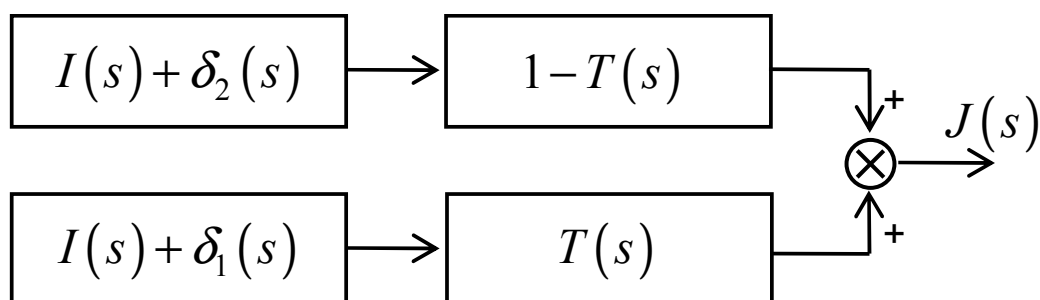
Fig. C.1. Structure usuelle d'un filtre complémentaire
