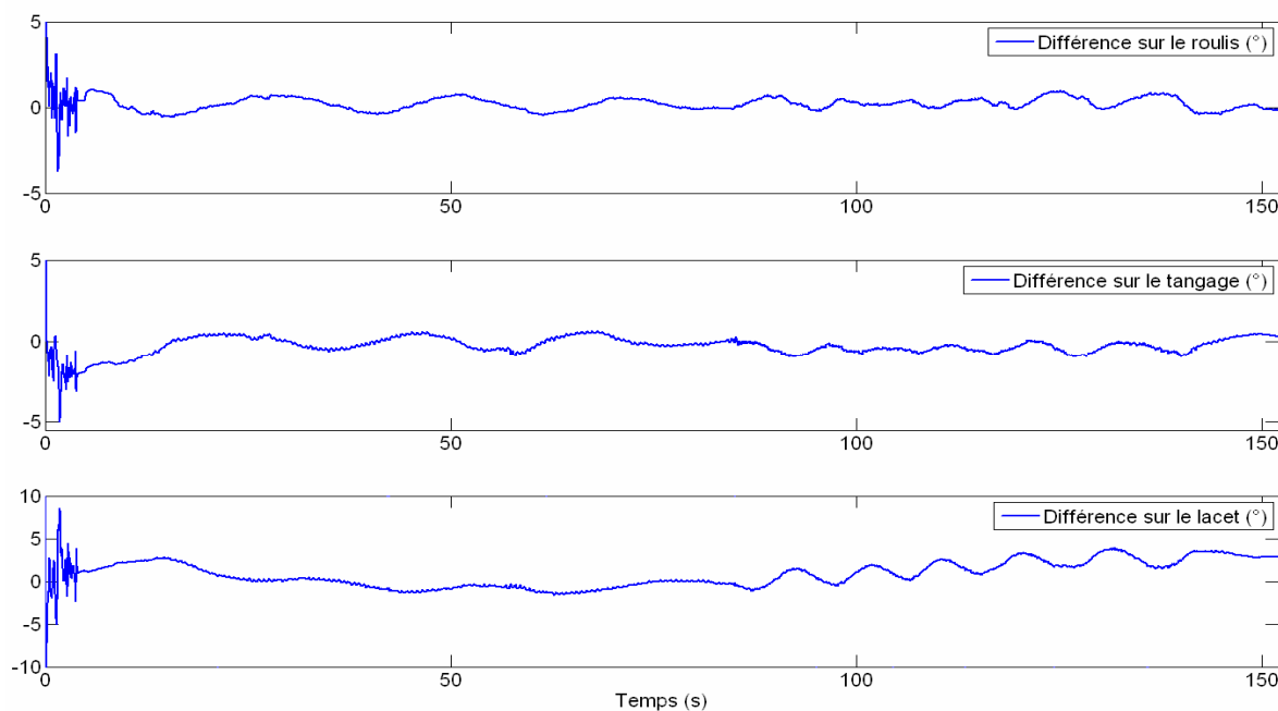
Fig. D.6. Evolution temporelle de la différence entre les angles d'Euler estimés par l'observateur à modes glissants et ceux calculés par la MTi-G au cours du mouvement réalisé par le cheval
