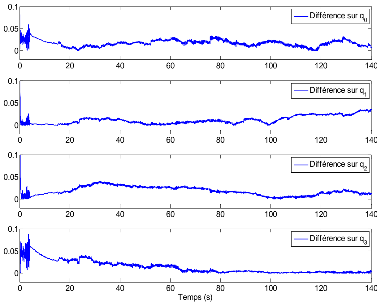
Fig. 4.21. Evolution temporelle de la différence entre le quaternion estimé par le filtre complémentaire et celui calculé par la MTi-G au cours du mouvement réalisé par le chien
