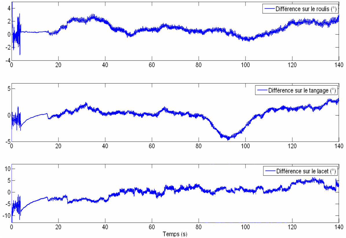
Fig. D.3. Evolution temporelle de la différence entre les angles d'Euler estimés par l'observateur non linéaire additif et ceux calculés par la MTi-G au cours du mouvement réalisé par le chien
