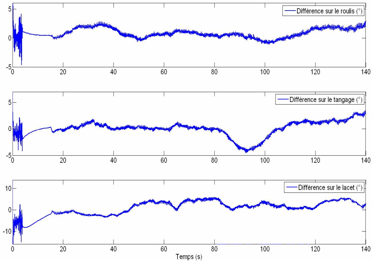
Fig. D.4. Evolution temporelle de la différence entre les angles d'Euler estimés par l'observateur à modes glissants et ceux calculés par la MTi-G au cours du mouvement réalisé par le chien
