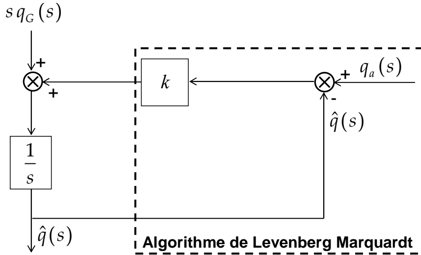
Fig. 3.11. Structure linéarisée du filtre complémentaire ramenée dans le domaine de Laplace
