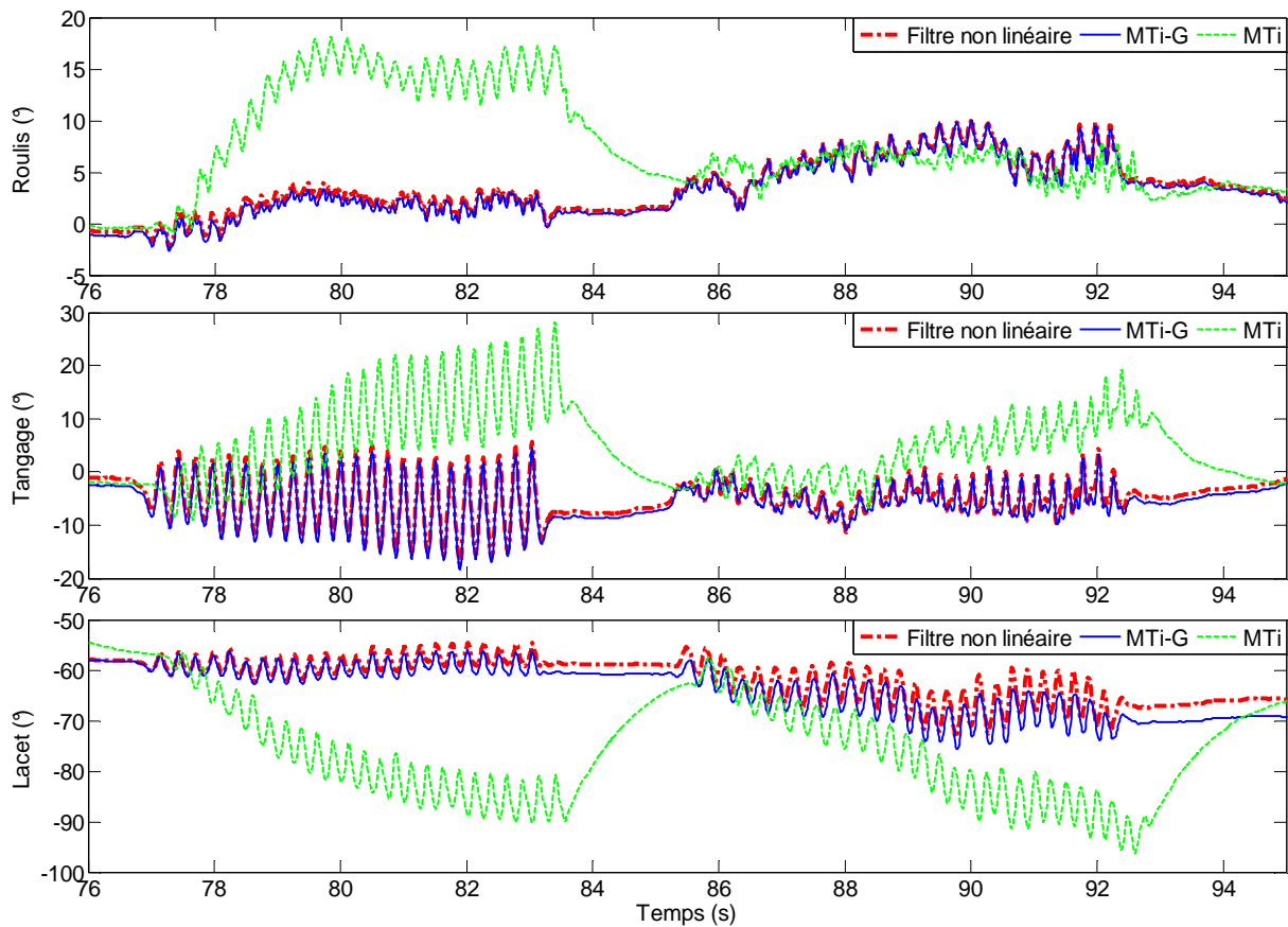
Fig. 4.36. Un zoom de l'intervalle [76 ; 95 sec] de la figure 4.35
