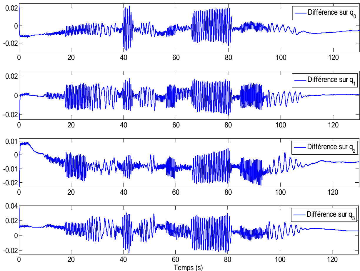
Fig. 4.14. Evolution temporelle de la différence entre le quaternion estimé par le filtre complémentaire et celui calculé par la MTi-G au cours du mouvement réalisé par la main
