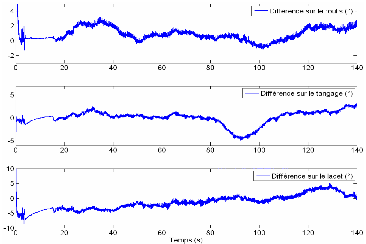
Fig. 4.23. Evolution temporelle de la différence entre les angles d'Euler estimés par le filtre complémentaire et ceux calculés par la MTi-G au cours du mouvement du chien
