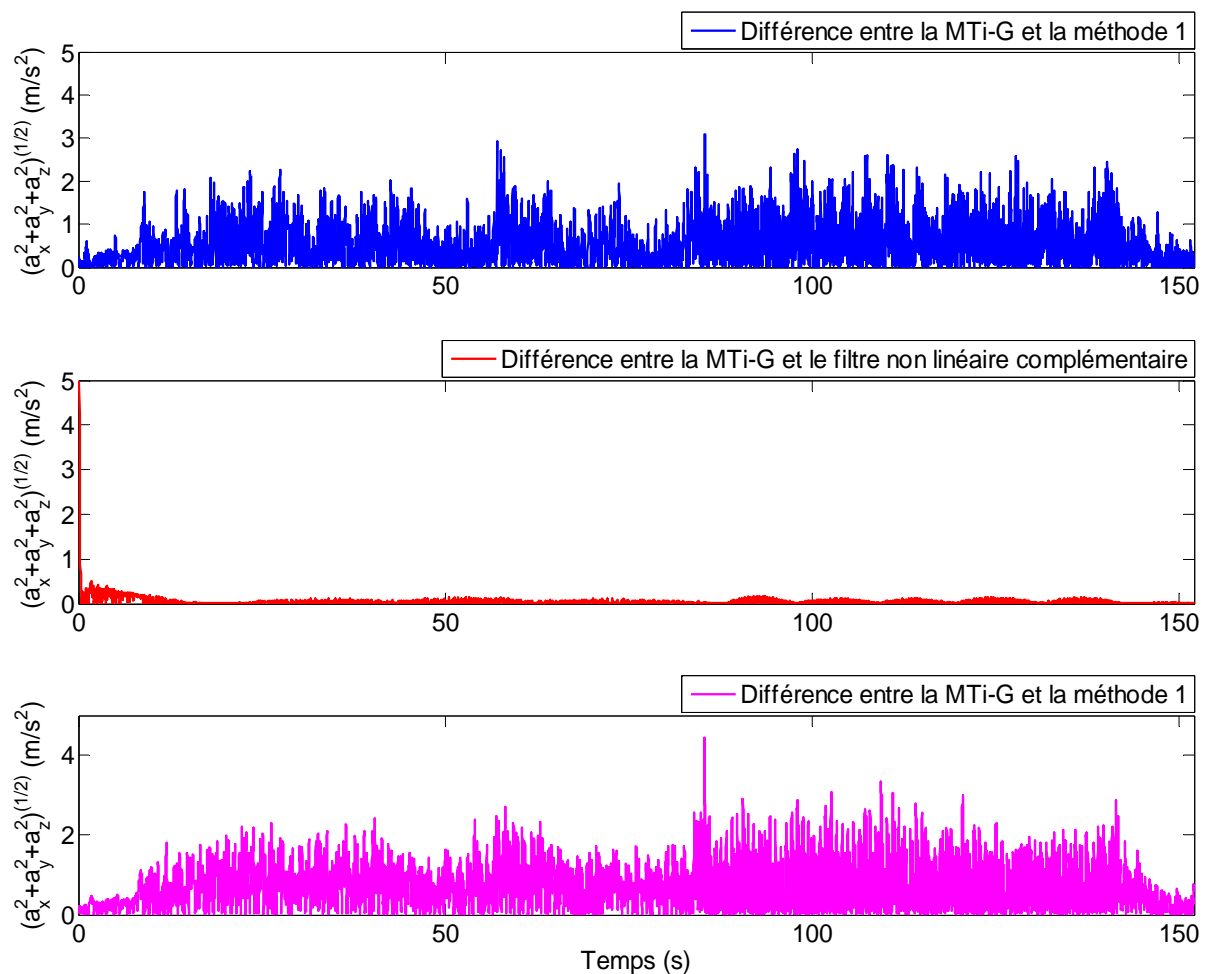
Fig. 4.40. Evolution de l'erreur d'estimation de la norme des accélérations propres du cheval
