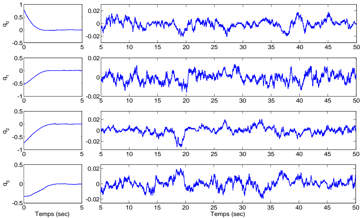
Fig. 3.9. Erreurs d'estimation sur les composantes du quaternion obtenues avec l'observateur à modes glissants (avec un zoom entre 5 et 50 sec)
