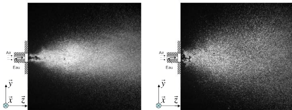
(g) (Sw3) - Strioscopie diphasique : R_{ac} = 0.2 (h) (Sw3) - Strioscopie diphasique : R_{ac} = 0.5
