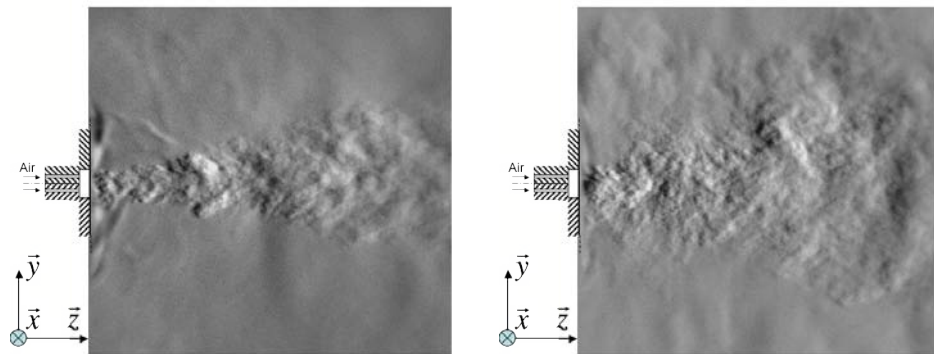
(e) (Sw3) - Strioscopie monophasique : R_{ac} = 0.2 (f) (Sw3) - Strioscopie monophasique : R_{ac} = 0.5
