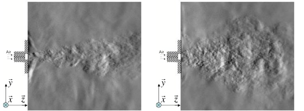
(a) (Sw2) - Strioscopie monophasique : R_{ac} = 0.2 : (b) (Sw2) - Strioscopie monophasique : R_{ac} = 0.5
