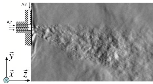
(b) (Dev55) - Strioscopie monophasique : R_{ac} = 0.4
