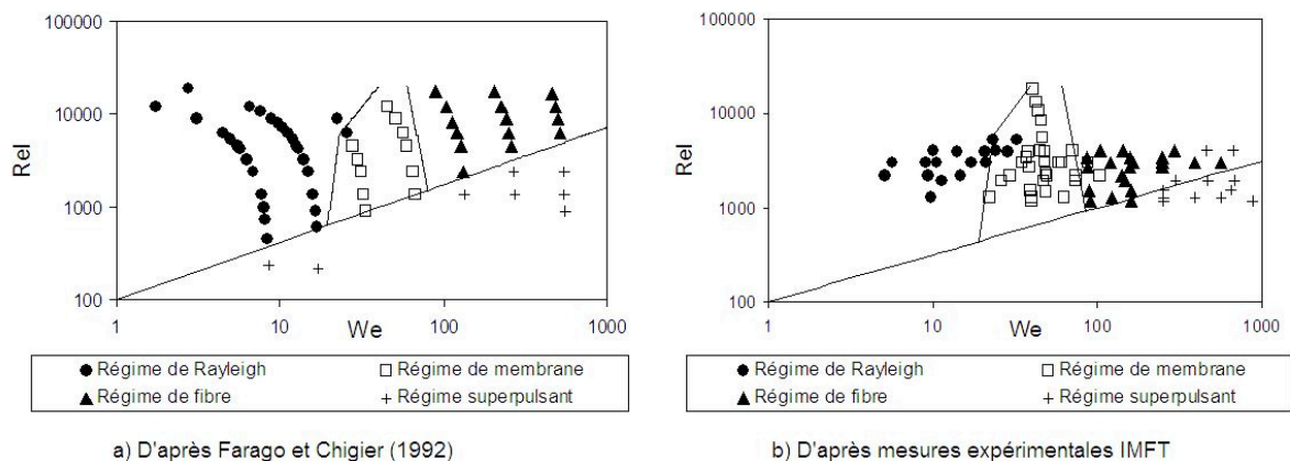
FIGURE 2.4 – Cartographies des régimes d'atomisation en fonction de We et Re_l . Comparaison des résultats de cette thèse (droite) avec Farago et Chigier [26].
