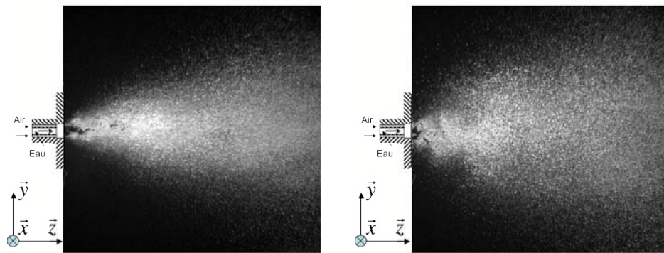
(c) (Sw2) - Strioscopie diphasique : R_{ac} = 0.2 (d) (Sw2) - Strioscopie diphasique : R_{ac} = 0.5
