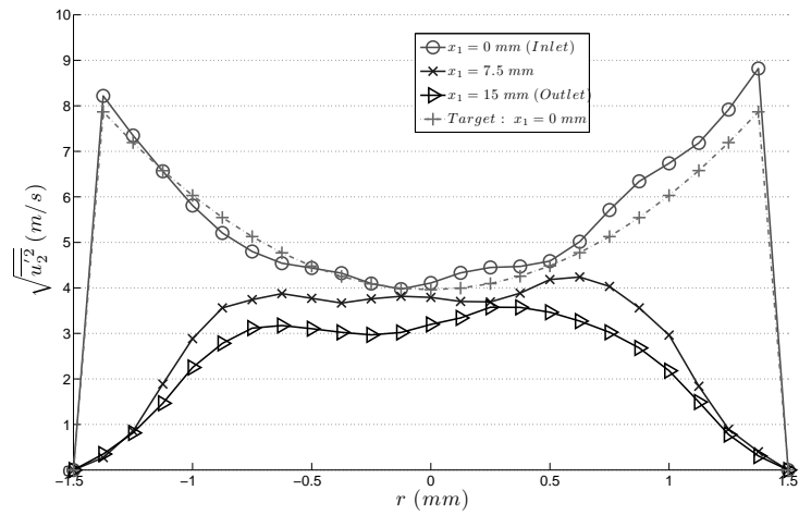
(b) \sqrt{u_2'^2}
