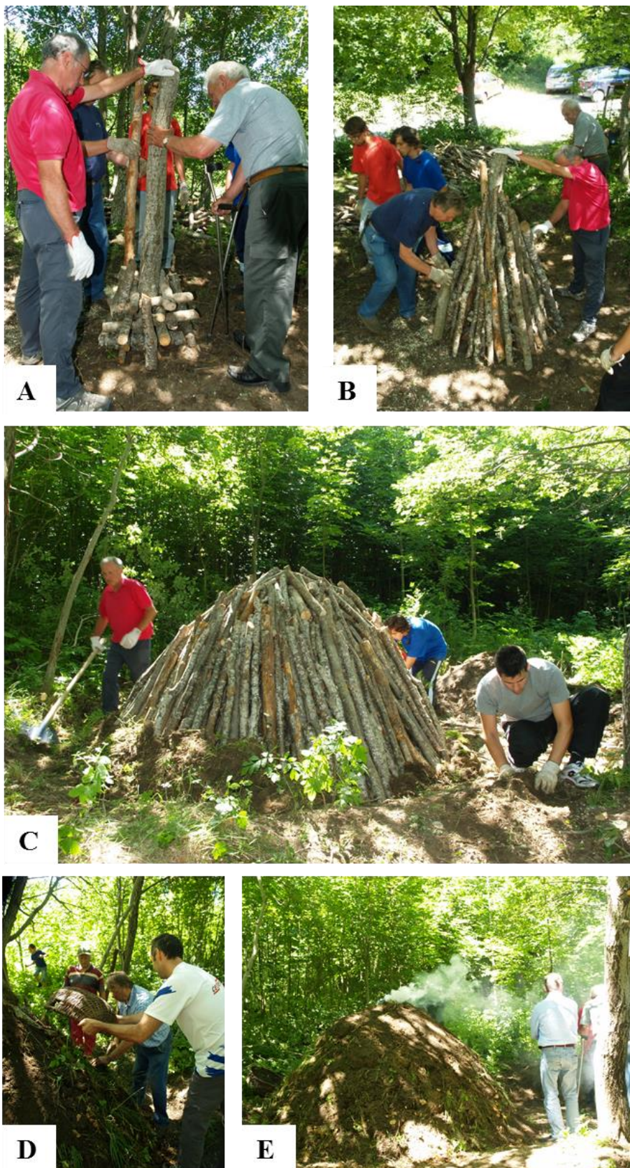
Figura 24. Alcune fasi della ricostruzione storica della carbonaia realizzata nel 2010 dal carbonaio Orlando su iniziativa del CAI di Sassuolo. A: costruzione della “rocchetta” e del camino centrale; B: posa dei primi pezzi; C: catasta di legna a forma di cupola completata; D: impermeabilizzazione o copertura della carbonaia; E: accensione della carbonaia. (Foto D. Maccaferri - gentilmente fornite dal Sig. Claudio Fregni).
