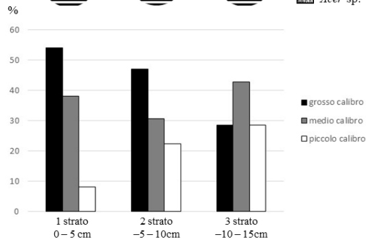
Figura 64. Risultati ottenuti dallo studio della piazzola da carbonaia “Carbo MC-2” localizzata sul versante nord-ovest del Monte Cimone.
