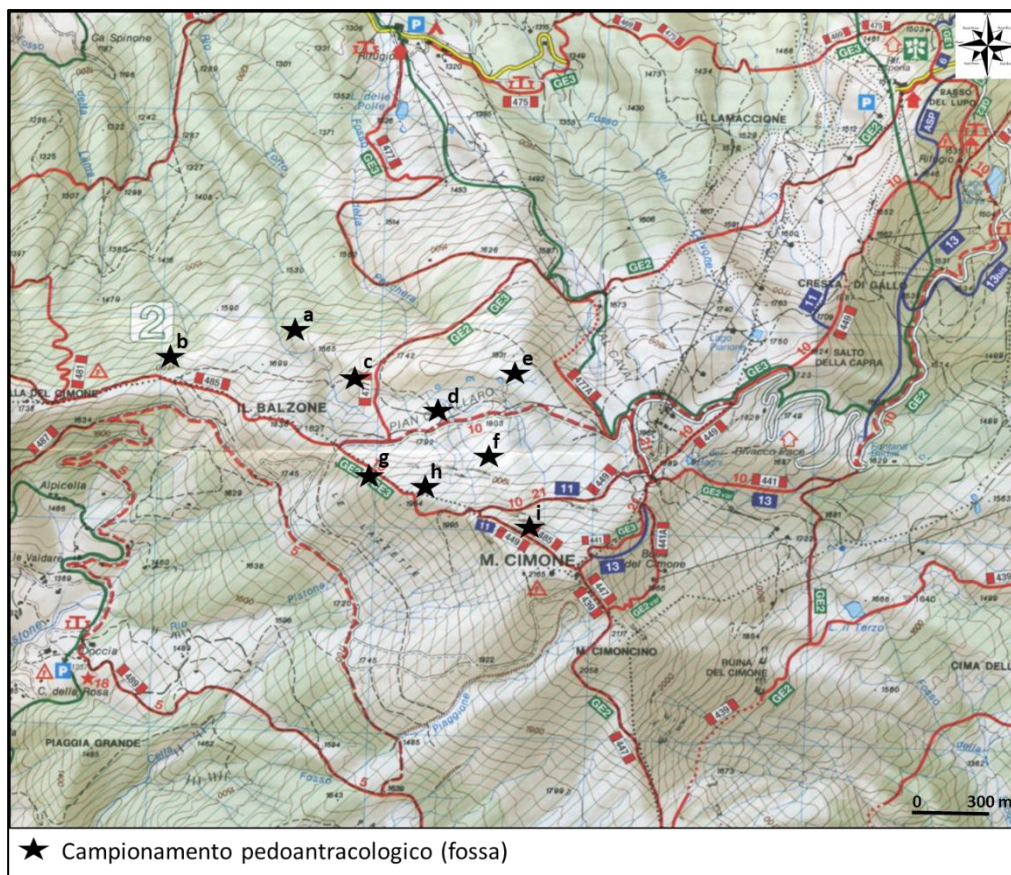
Figura 33. Localizzazione dei 9 punti di campionamento pedoantracologico effettuati nel versante nord-ovest del Monte Cimone.
