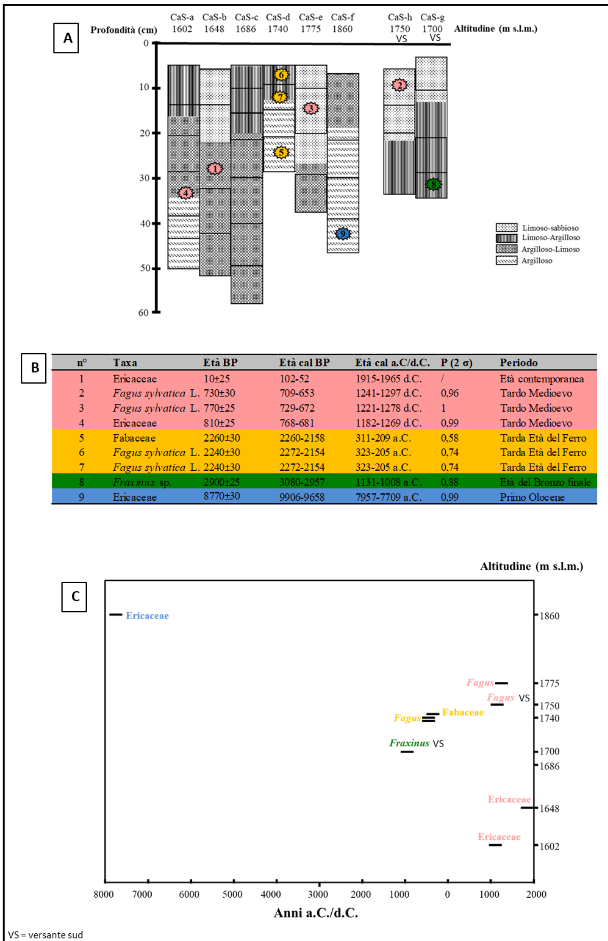
Figura 59. Datazioni ^{14}\text{C} effettuate nell'area del Corno alle Scale, evidenziate sulla base del periodo storico di appartenenza. A: Posizione dei carboni datati lungo il profilo del suolo; B: Tabella riassuntiva delle datazioni; C: Datazioni rappresentate in base all'altitudine delle fosse dei carboni datati.
