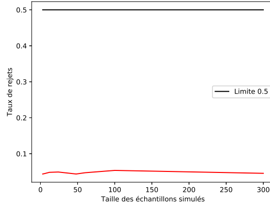
FIGURE 2.3 – Taux de rejets du test d’ajustement selon AD en fonction de la taille des échantillons simulés selon la loi de Rayleigh.
