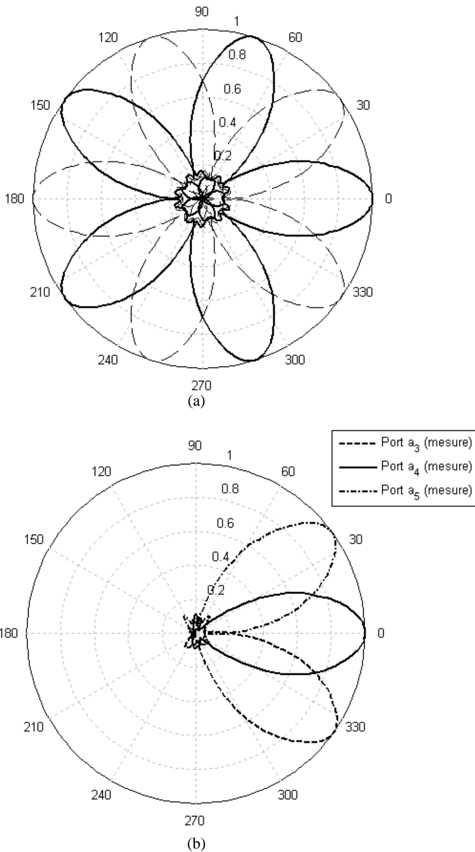
Figure 109 : Diagrammes de rayonnement en amplitude normalisés : (a) simulation et (b) mesure dans le cas du réseau circulaire à 20 patches
