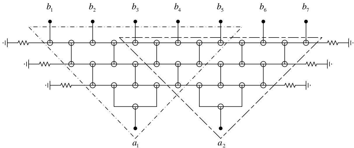
Figure 99 : Réseau d'alimentation périodique à pertes intrinsèques réduites
