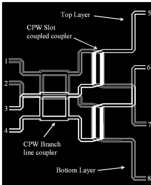
Figure 35 : Matrice de Butler 4×4 en technologie CPW deux couches [54]
