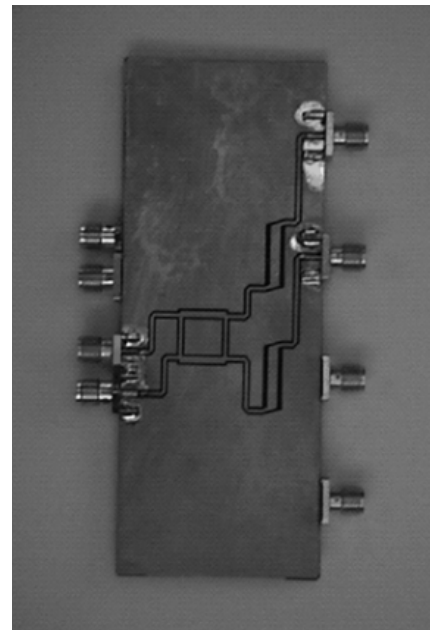
Figure 35 : Matrice de Butler 4×4 en technologie CPW deux couches [54]
