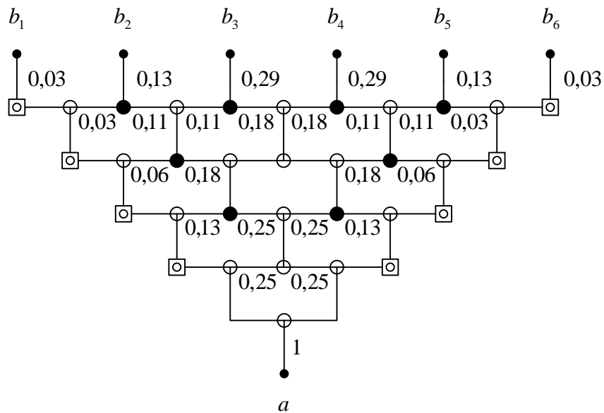
Figure 86 : Réseau d'alimentation périodique monofaisceau large bande
