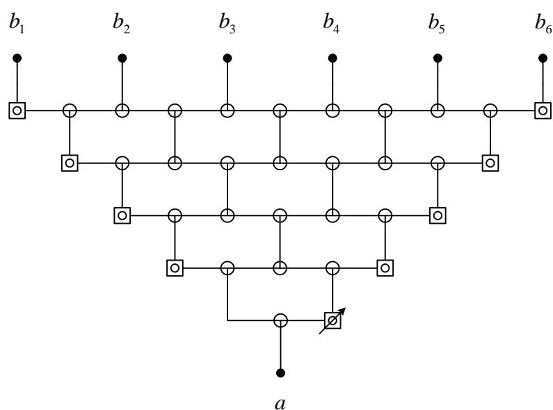
Figure 91 : Matrice périodique monofaisceau à balayage électronique
