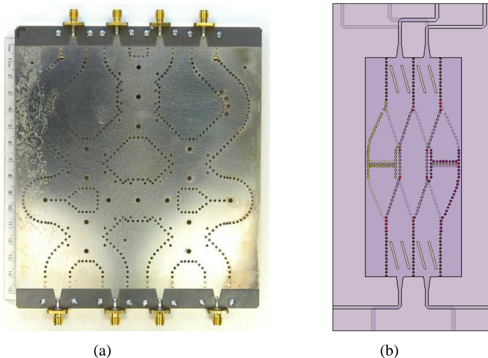
Figure 45 : Matrice de Butler 4x4 en technologie GIS (a) planaire [64] et (b) sur deux couches [63]
