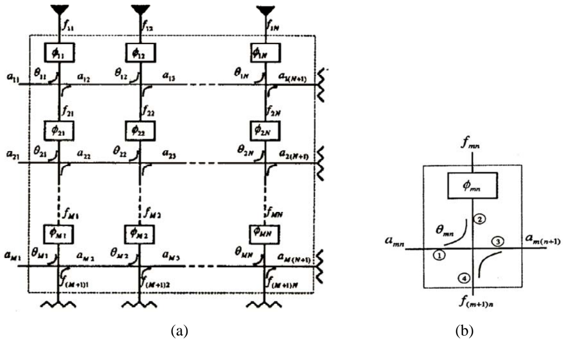
Figure 21 : (a) Schéma fonctionnel de la matrice de Blass à M entrées et N sorties et (b) détail d'un nœud de la matrice [36]
