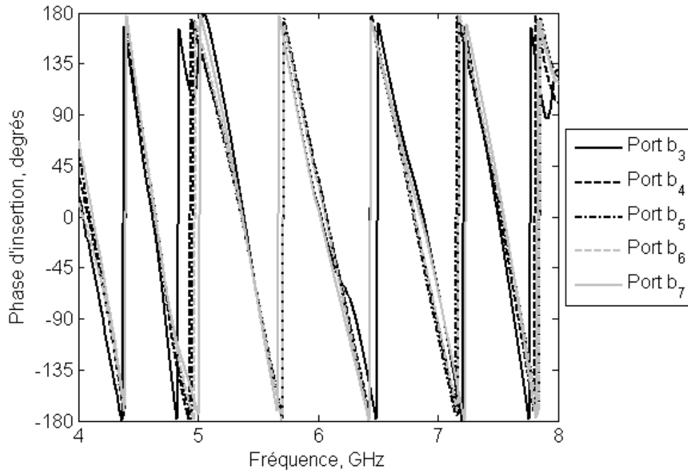
Figure 156 : Phases d'insertion associées à l'entrée 3 du réseau périodique 3 vers 7 à quatre couches
