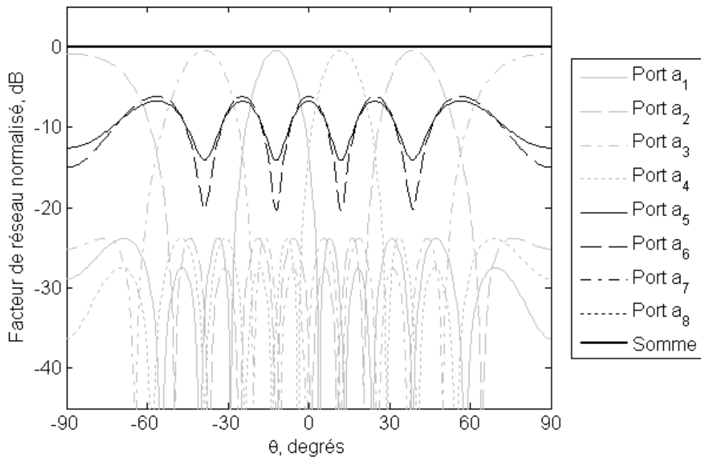
Figure 61 : Facteurs de réseau normalisés obtenus avec les ports chargés de la matrice de Nolen 4x8 à loi d'amplitude non-uniforme
