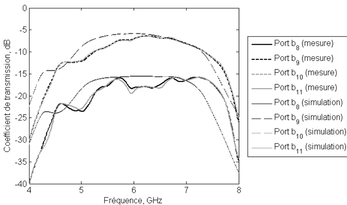
Figure 167 : Coefficients de transmission associés à l'entrée 5 du réseau périodique refermé 7 vers 14 à trois couches
