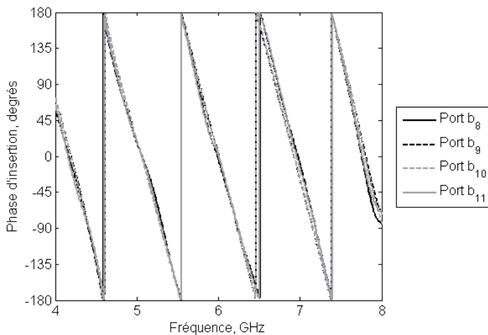
Figure 170 : Phases d'insertion associées à l'entrée 5 du réseau périodique refermé 7 vers 14 à trois couches
