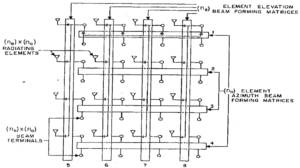
Figure 69 : Matrices de Butler pour réseaux rayonnants plans carrés [12]
