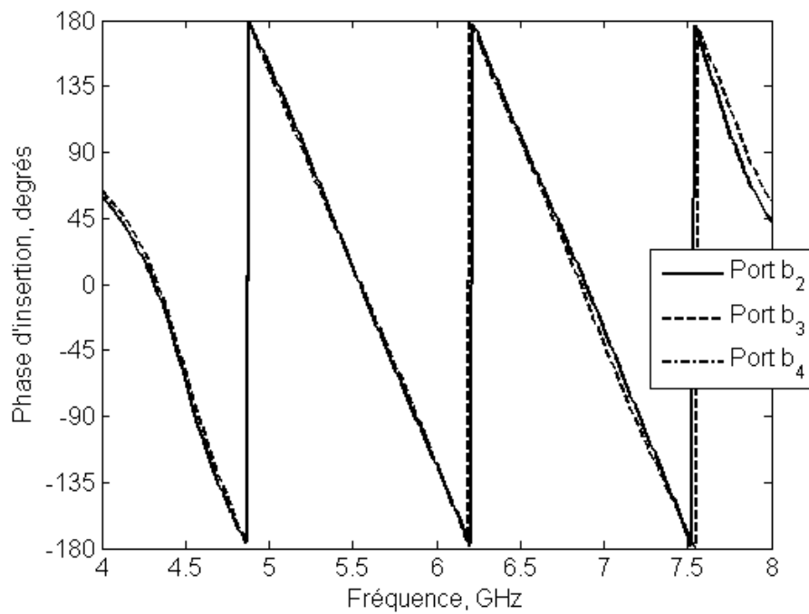
Figure 147 : Phases d'insertion associées à l'entrée 2 du réseau périodique 3 vers 5 à deux couches
