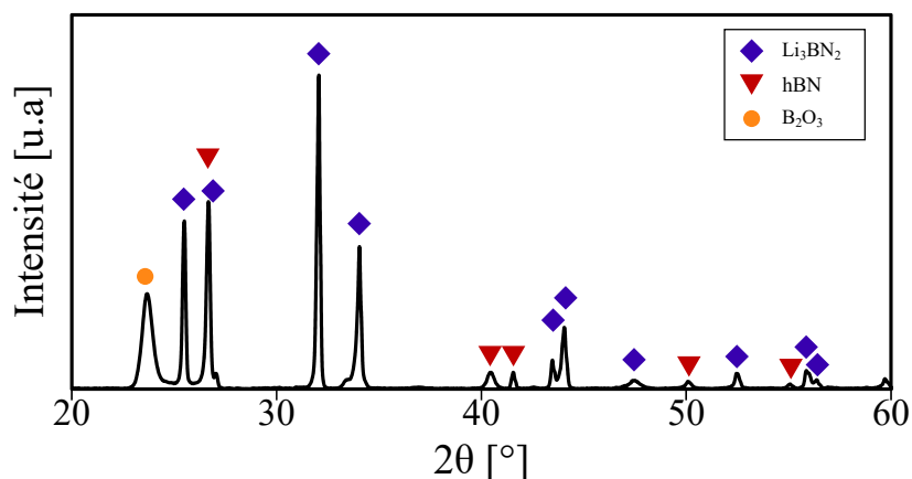
Figure 3.17 – Diffractogramme de DRX du produit de \text{Li}_3\text{BN}_2 après traitement thermique à pression atmosphérique pendant 4h à 1200\text{ }^\circ\text{C} .
