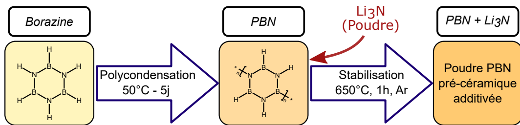
Figure 1.16 – Procédé de préparation du précurseur précéramique pour la synthèse de hBN
