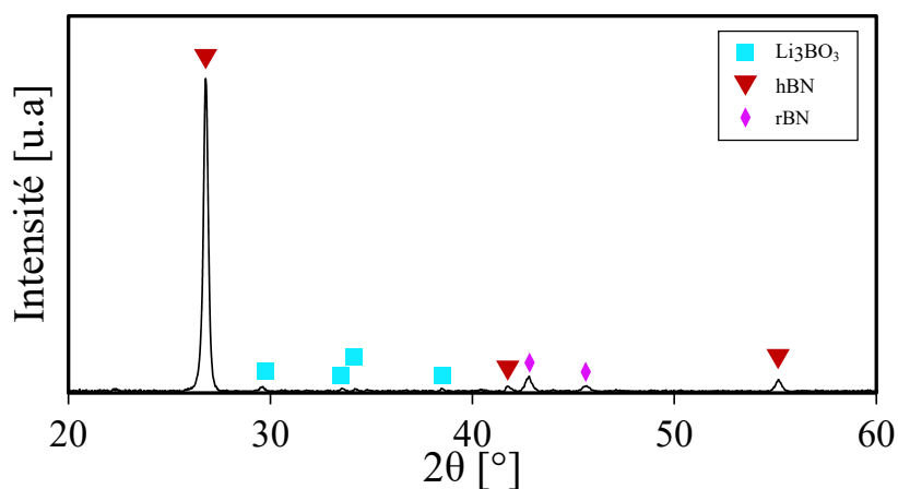
Figure 3.18 – Diffractogramme de DRX du produit de \text{Li}_3\text{BN}_2 après traitement thermique à pression atmosphérique pendant 4h à 1300\text{ }^\circ\text{C} .
