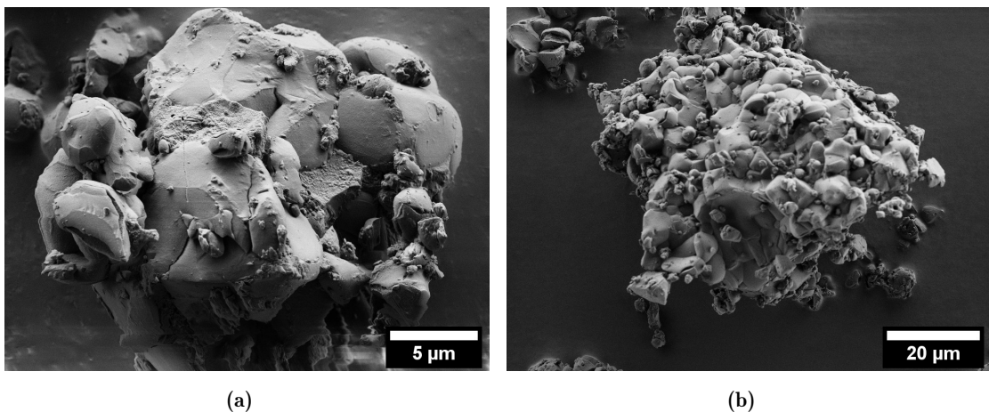
Figure 3.2 – Images MEB de grains représentatifs du précurseur précéramique composé de 30 wt% PBN + 70 wt% \text{Li}_3\text{BN}_2 : (a) grain micrométrique ; (b) grain présentant une taille latérale de plusieurs dizaines de microns. Les deux composés sont indissociables.
