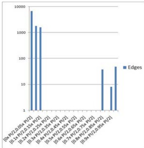
FIGURE 3.13 – Classement des angles entre facettes dans le maillage
