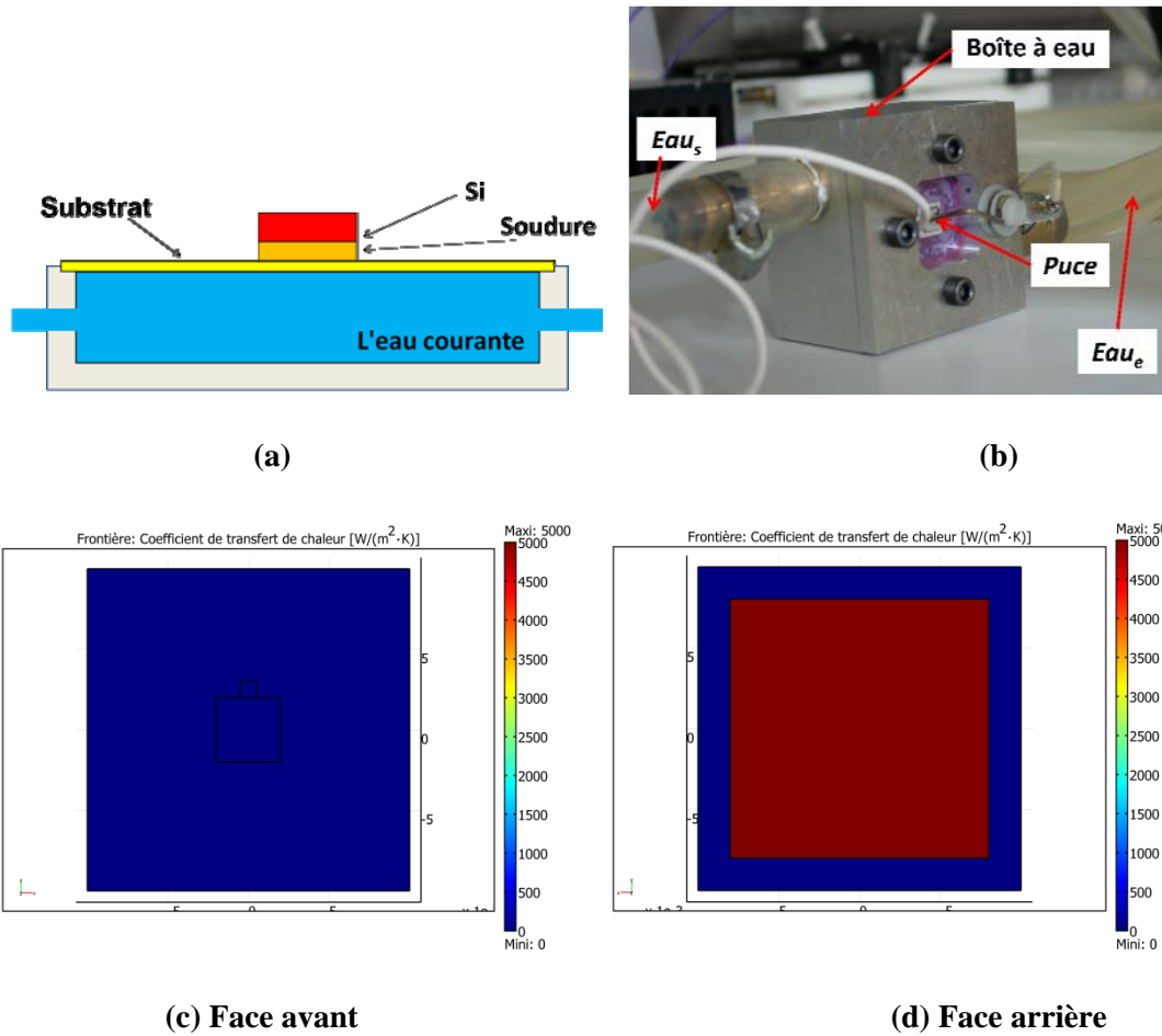
Figure II.9: Description du dispositif de mesure de l'échange convectif par lame d'eau (a),(b) : Description et mise en œuvre de la boîte à eau. (c) Coefficient h sur la face supérieure. (d) Coefficient h sur la face inférieure en contact avec l'eau
