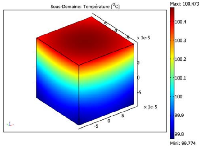
Figure II.24 Simulation d'un micropoteau 200\mu\text{m}^3 en cuivre chauffé par le haut refroidi dans de l'eau à 20^\circ\text{C} . Mise en évidence de la faible variation de température le long du poteau
