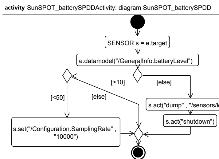
FIGURE 4.4 – PDD pour le "self-configuring" de paramètres internes d'un capteur
