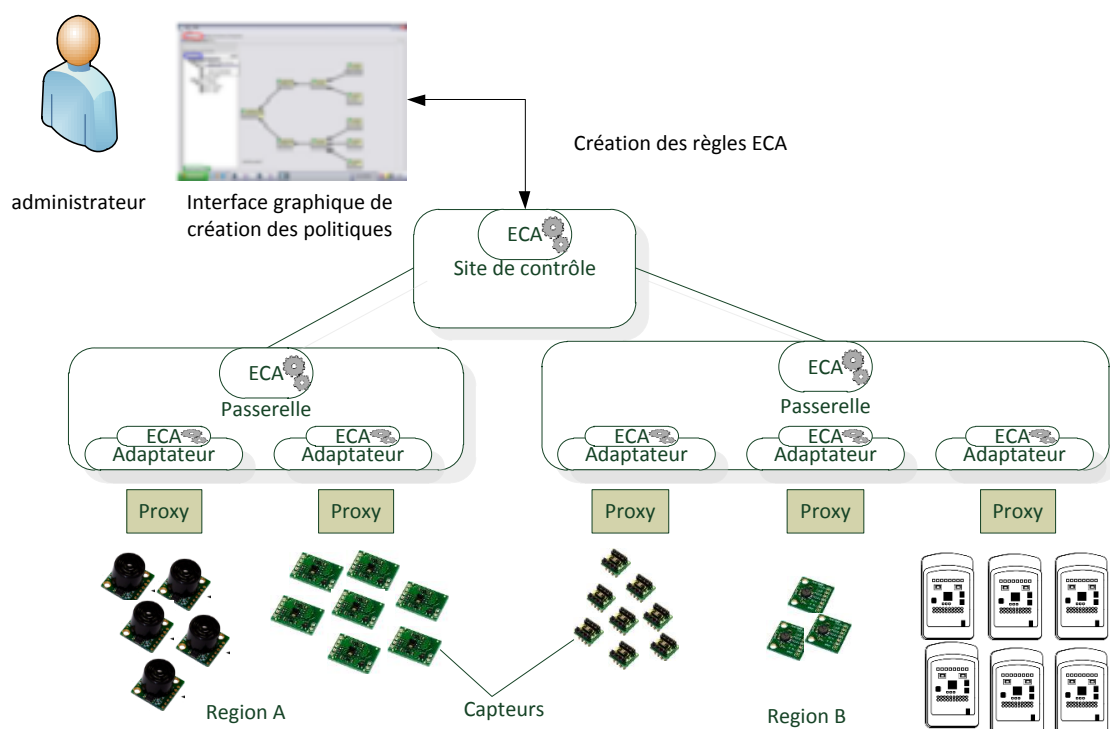
FIGURE 4.1 – Intégration de services ECA dans l'architecture hiérarchique de XSSstreamWare
