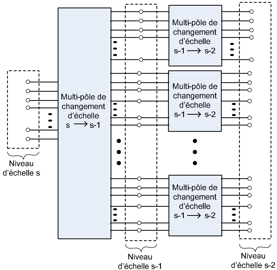
Figure III.4 : Multi-pôle de changement d'échelle permettant de relier le champ électromagnétique transverse, de l'échelle s à l'échelle s-1 [7].
