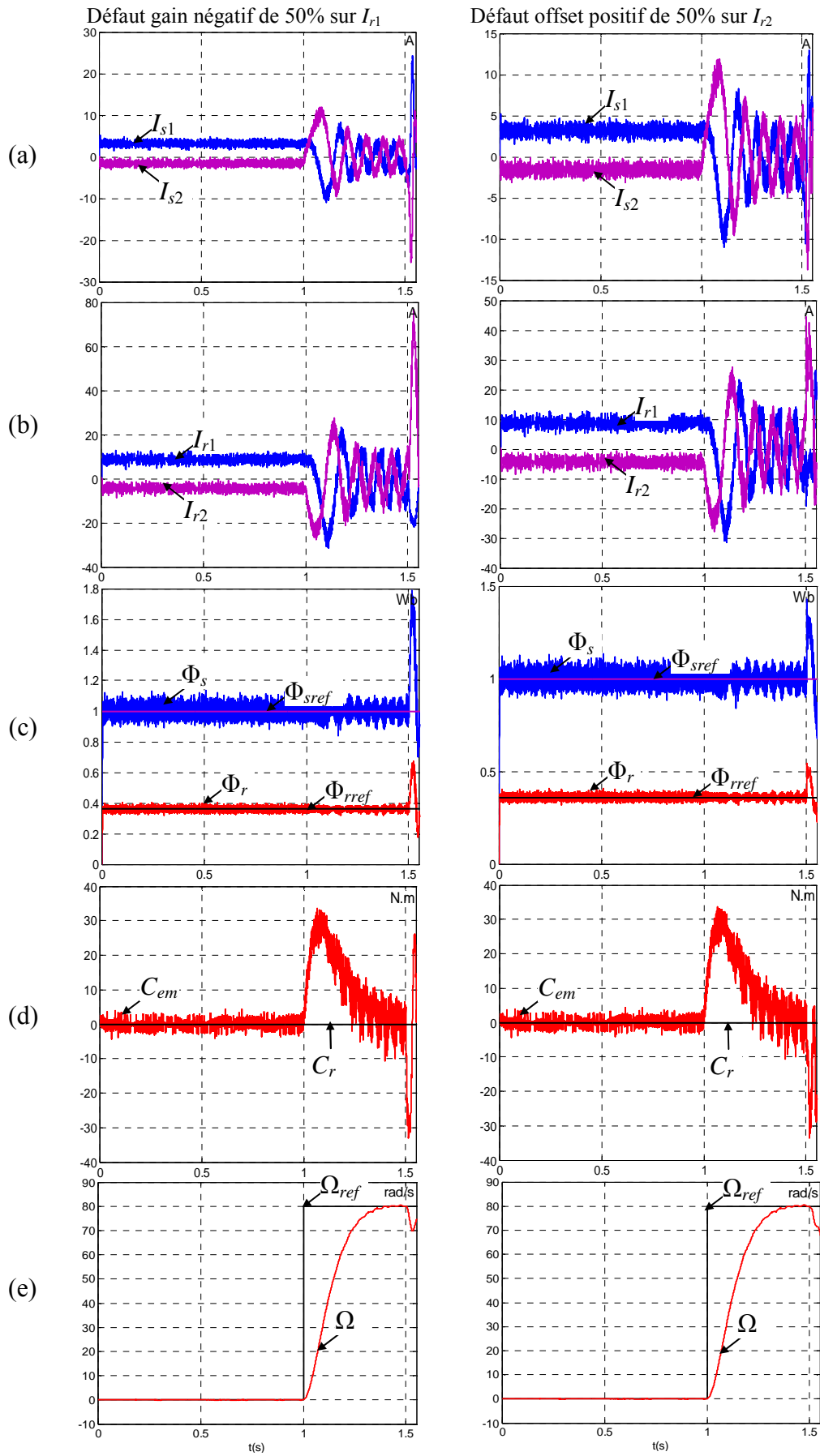
Figure2. 20. Effets de défaut capteurs courants rotoriques (phase1 et phase 2) gain et offset.
