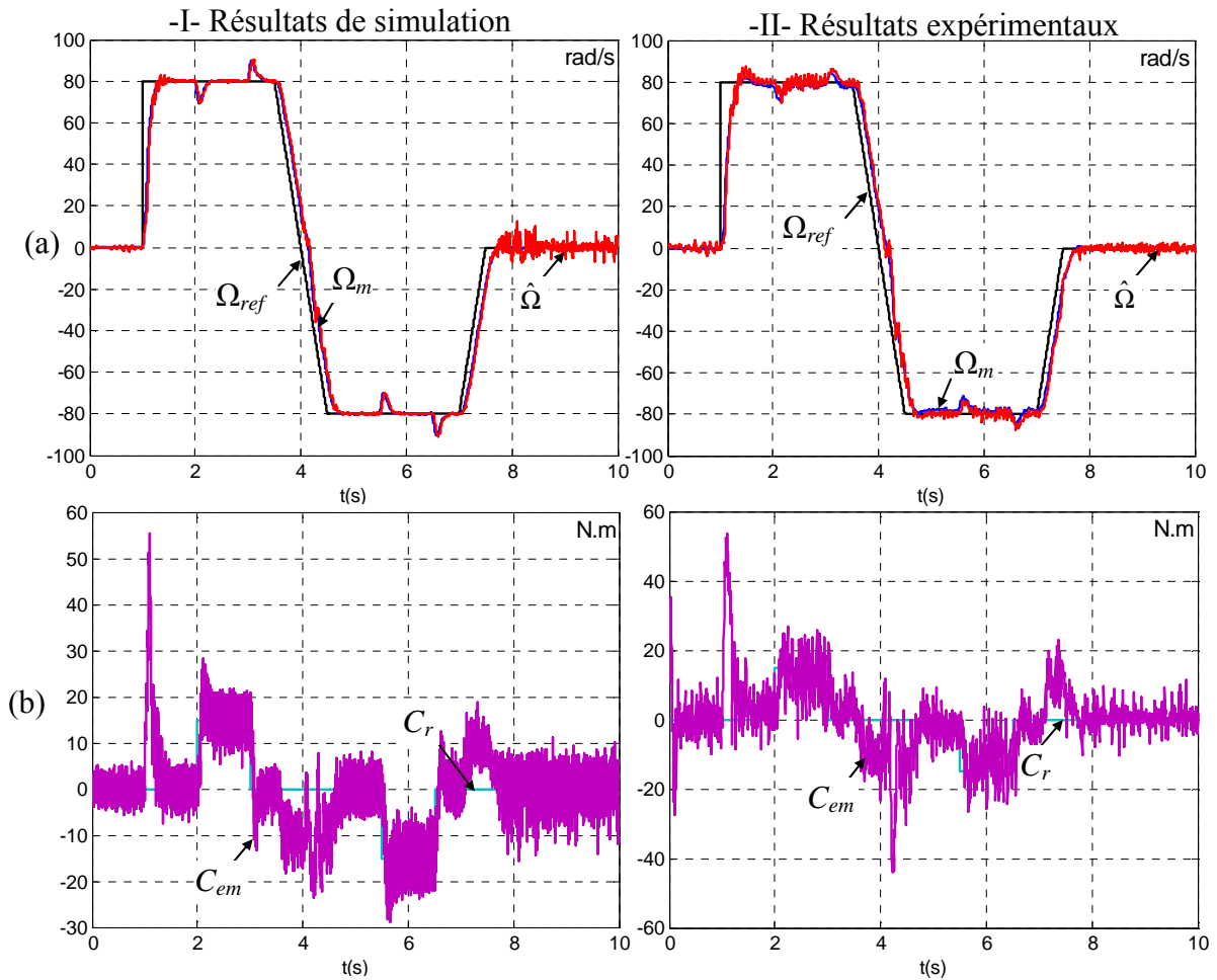
Figure 4. 12. Résultats obtenus par simulation et expérimentalement pour le fonctionnement en BF de l'estimateur (a) : cycle de la vitesse et (b) : allure du couple électromagnétique.
