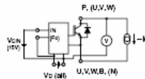
Fig. 2 V_{ce, (Vsw)} Test
