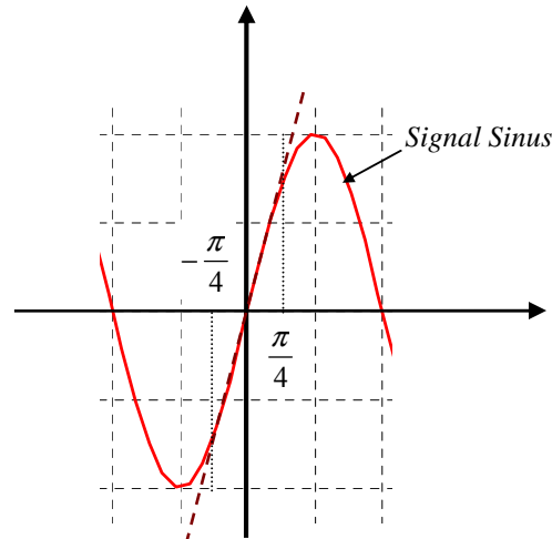
Figure 4. 5. Zone de linéarité du signal sinusoïdal.
