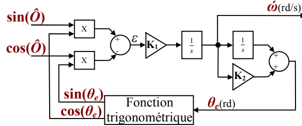
Figure 4. 4. Principe général de calcul de la vitesse utilisant l'algorithme de l'ATO.
