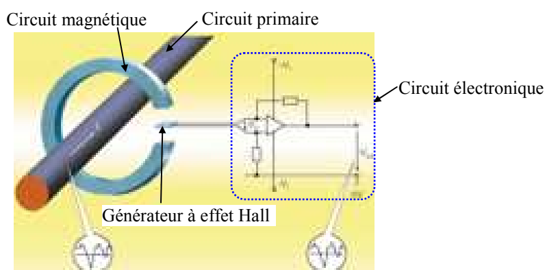
Figure 1. 9. Composition d'un capteur à effet Hall de courant en boucle ouverte [14]
