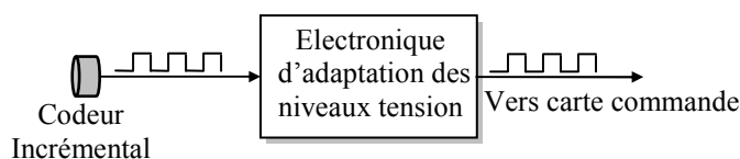
Figure 1. 16. Chaîne d'acquisition pour un codeur incrémental.
