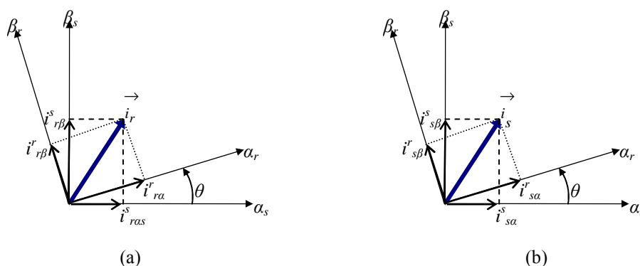
Figure 4. 1. Les différentes composantes des vecteurs courant (a) : rotorique ; (b) : statorique dans els repères \alpha_s\beta_s et \alpha_r\beta_r .
