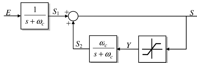
Figure 3. 5. Principe de l'intégrateur à utiliser.
