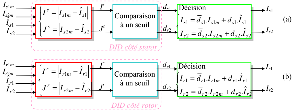
Figure 3. 3. Algorithme DID capteur courant détaillé (a) : côté stator ; (b) : côté rotor.
