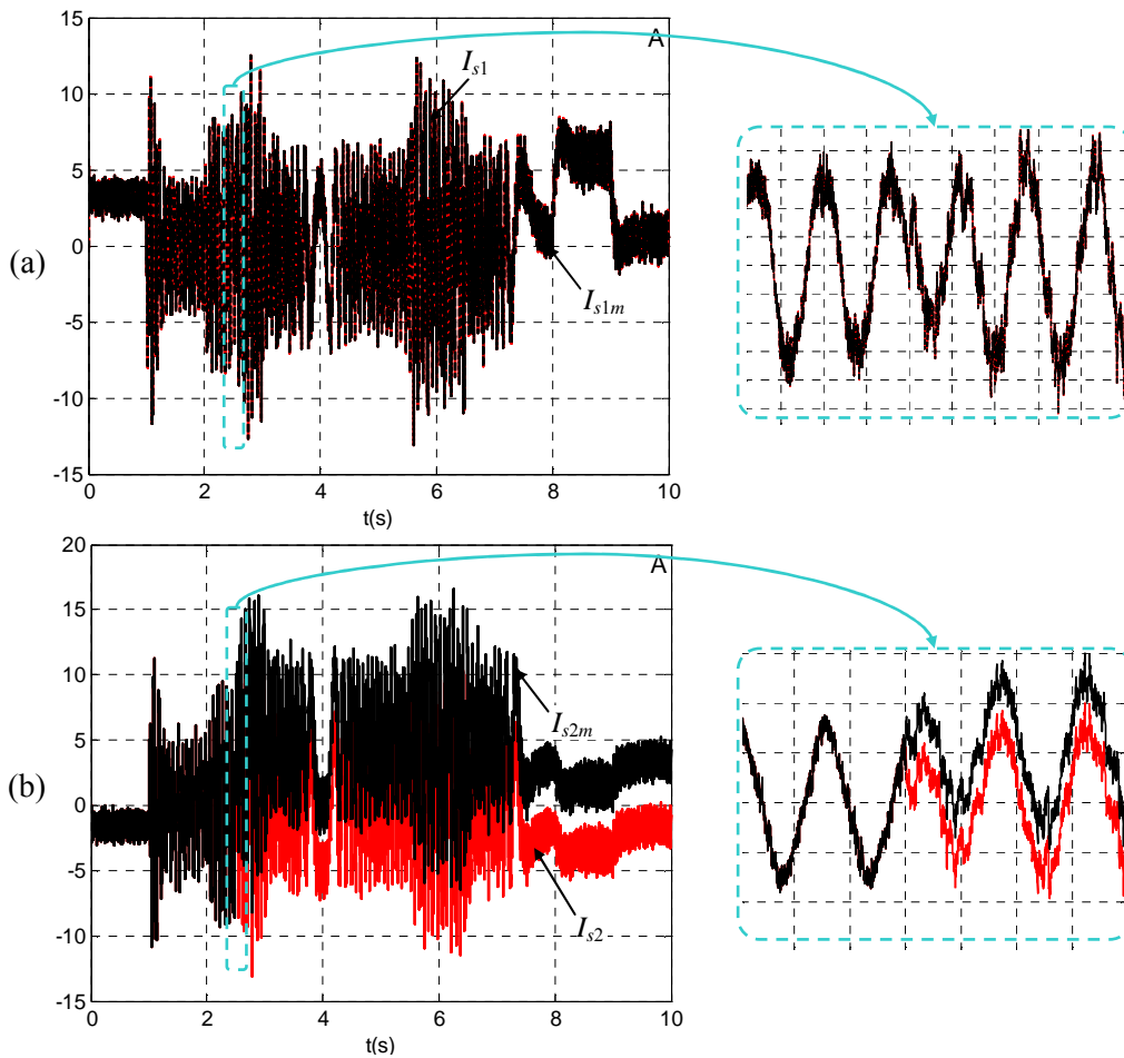
Figure 3. 23. Résultats de simulation obtenus avant et après un défaut capteur statorique de la deuxième phase (a) : allure des courants statoriques de la phase1 ; (b) : allure des courants statoriques de la phase 2.
