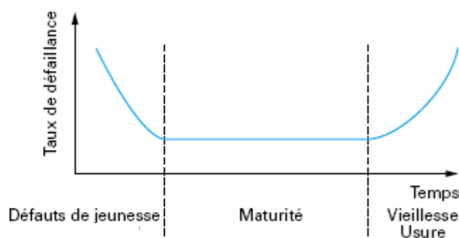
Figure 1. 1. Courbe du taux de défaillance d'un composant quelconque en fonction du temps : courbe en baignoire [2].
