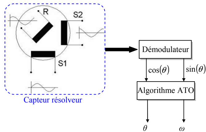
Figure 4. 2. Principe de calcul de la position en présence d'un capteur type résolveur.
