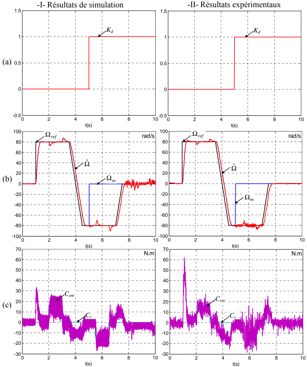
Figure 4. 21. Fonctionnement en supervision et application d'un défaut simulant la perte d'information à la sortie du capteur de vitesse à l'instant t=5.0s (a) : le marqueur permettant la détection et la reconfiguration, (b) : allures de la vitesse avant et après défaut, (c) : allure du couple électromagnétique avant et après défaut.
