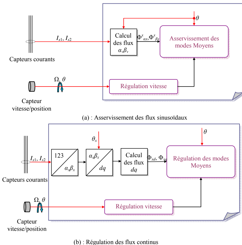
Figure 1. 6. Commande basée sur la régulation des modes moyens.
