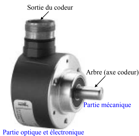
Figure 1. 14. Exemple d'un codeur incrémental commercialisé. [17].
