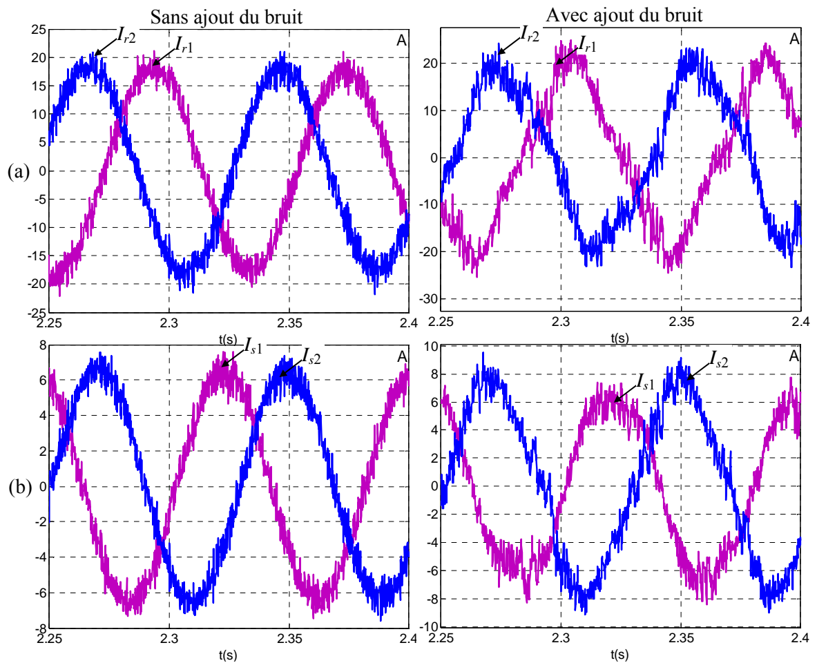
Figure2. 15. Allure des courants (a) : rotoriques et (b) : statoriques simulés avant et après ajout du bruit.
