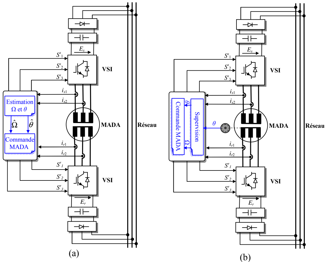
Figure 4. 9. Solutions proposées (a) : fonctionnement sans capteur de vitesse et (b) : fonctionnement en supervision.
