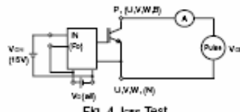
Fig. 4 I_{ces} Test
