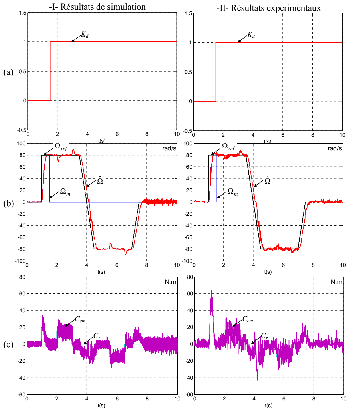
Figure 4. 20. Fonctionnement en supervision et application d'un défaut simulant la perte d'information à la sortie du capteur de vitesse à l'instant t = 1.5 s (a) : le marqueur permettant la détection et la reconfiguration, (b) : allures de la vitesse avant et après défaut, (c) : allure du couple électromagnétique avant et après défaut.
