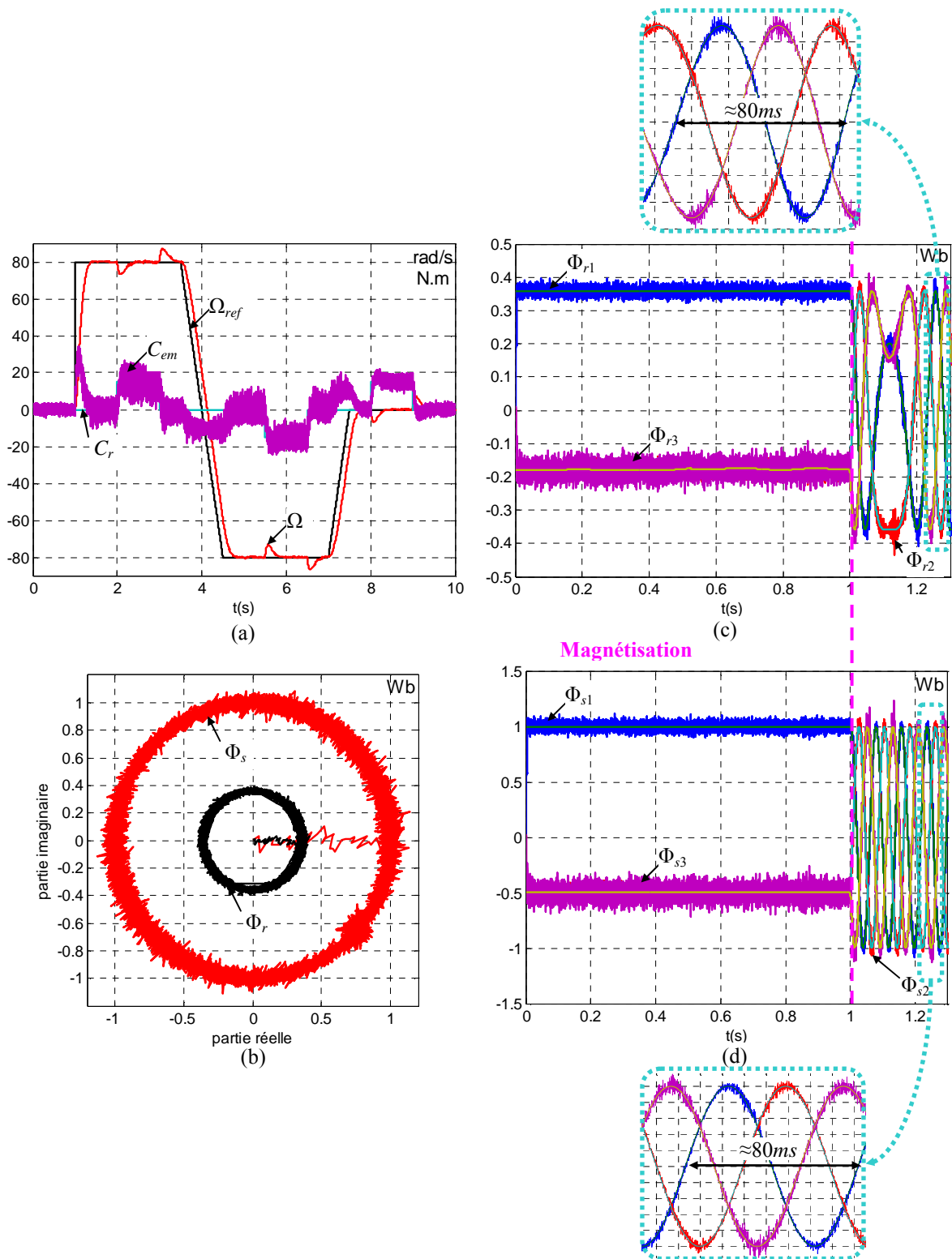
Figure2. 9. Résultats de simulation de la commande CDC
