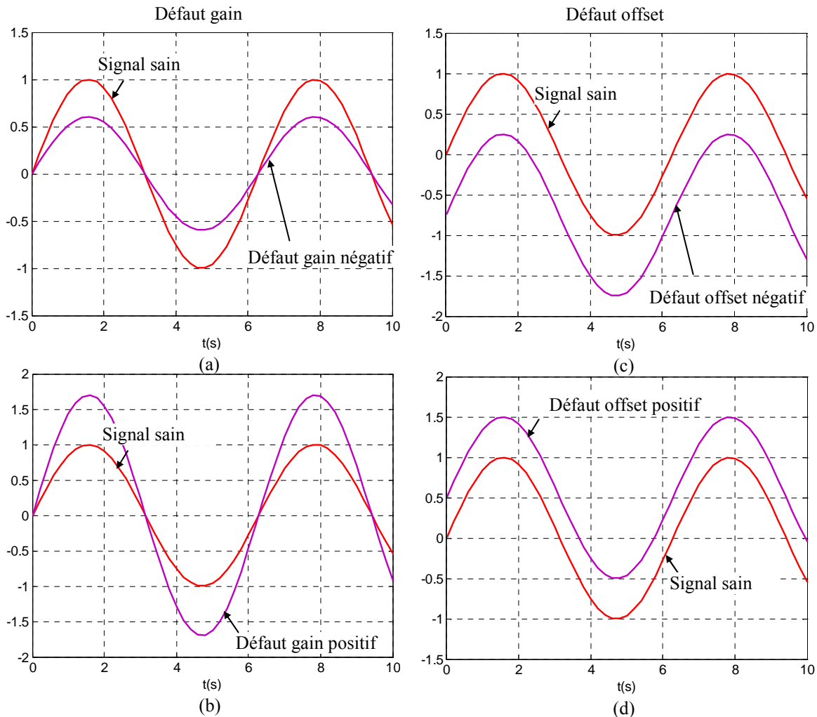
Figure 2.18. Allures de la sortie d'un capteur de courant dans le cas (a): d'un défaut de gain négatif; (b): d'un défaut de gain positif; (c): d'un défaut d'offset négatif; (d): d'un défaut d'offset positif.
