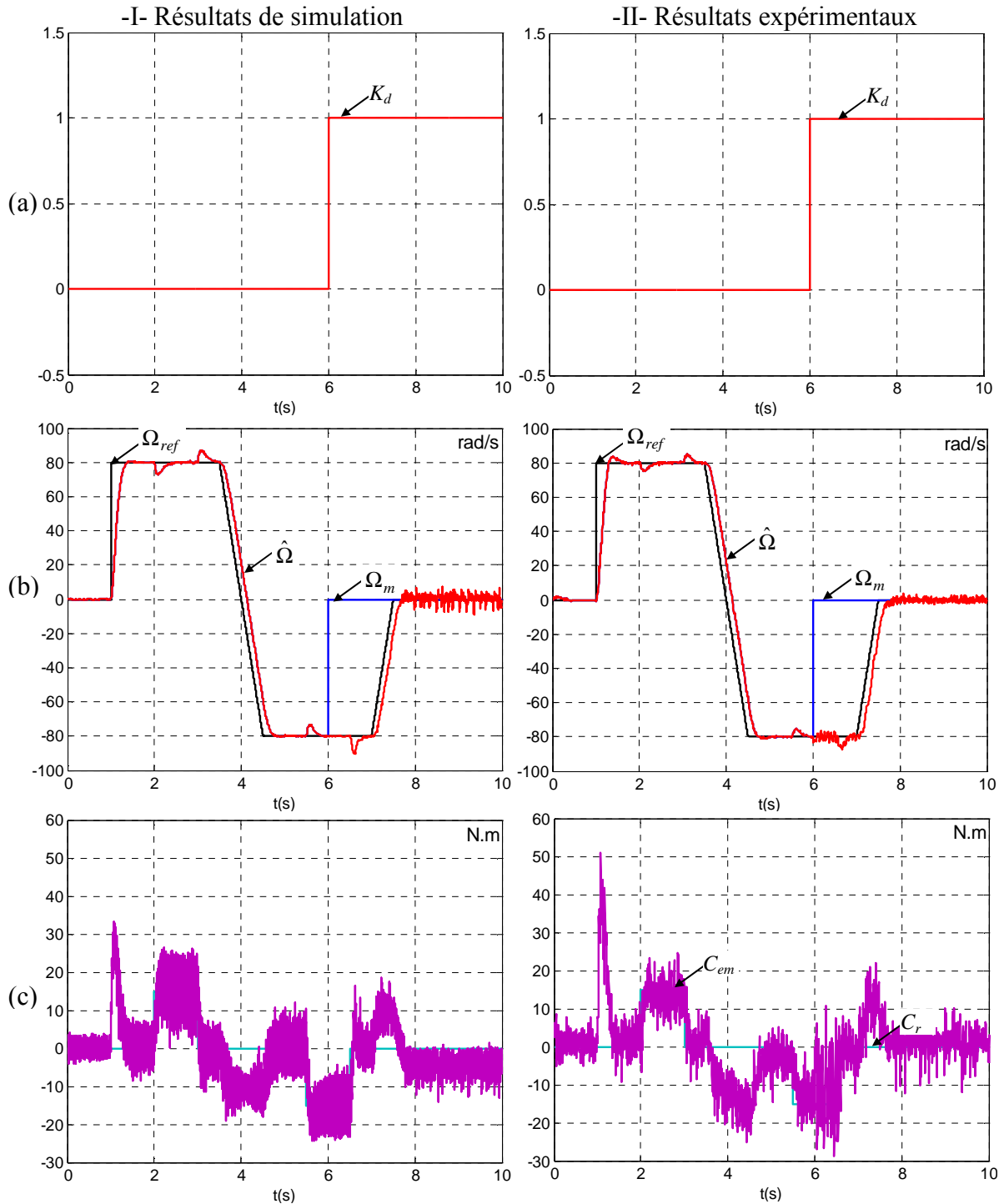
Figure 4. 23. Fonctionnement en supervision et application d'un défaut simulant la perte d'information à la sortie du capteur de vitesse à l'instant t=6.0 s (a) : le marqueur permettant la détection et la reconfiguration, (b) : allures de la vitesse avant et après défaut, (c) : allure du couple électromagnétique avant et après défaut.
