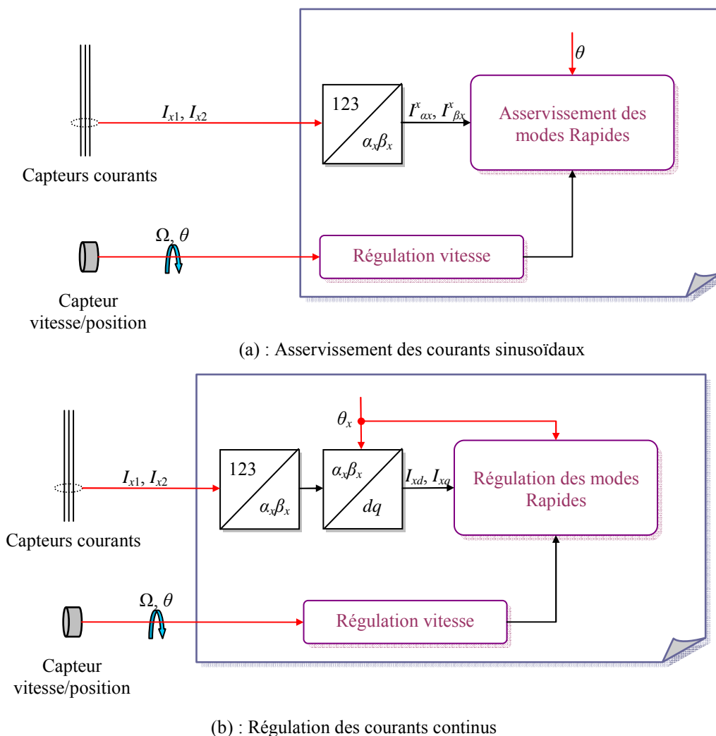
Figure 1. 5. Commande basée sur la régulation des modes rapides.
