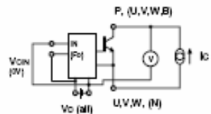
Fig. 1 V_{ce(sat)} Test
