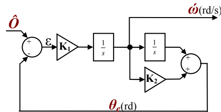
Figure 4. 6. Principe de calcul de la vitesse utilisant l'algorithme de l'ATO après simplification.
