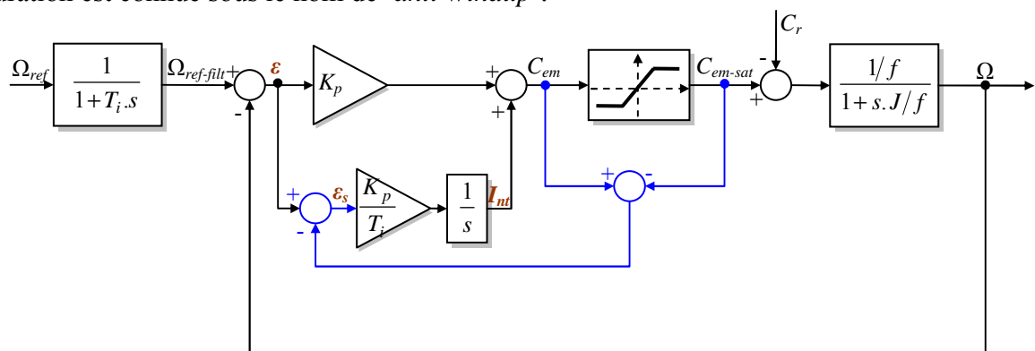
Figure2. 6. Structure du régulateur IP avec un anti-windup de la régulation de la vitesse mécanique.
