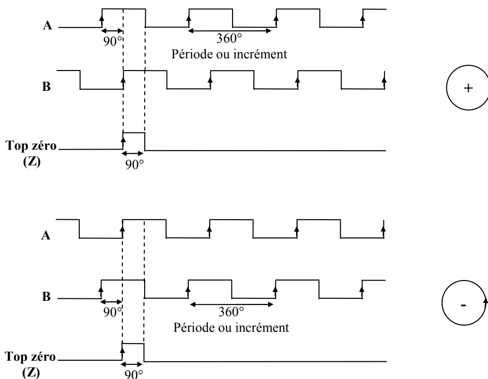
Figure 1. 13. Les signaux recueillis à la sortie du codeur incrémental.
