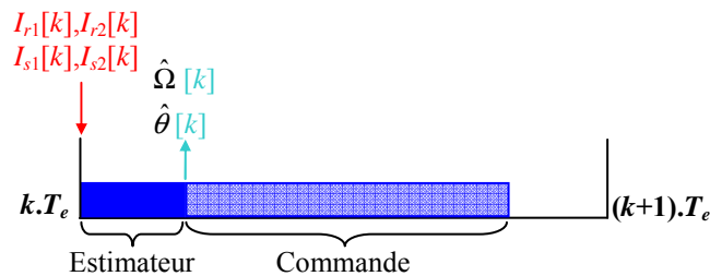
Figure 4. 10. Chronogramme quand le fonctionnement est sans capteur de vitesse/position.
