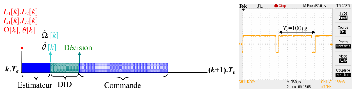
Figure 4. 15. Chronogramme quand le fonctionnement est en mode supervision.
