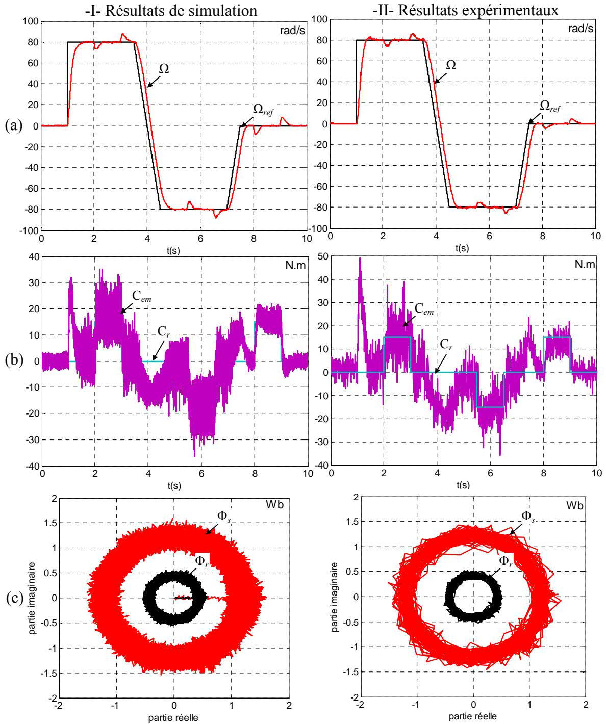
Figure 3. 14. Résultats de simulation et résultats expérimentaux obtenus sans capteurs statoriques (a) : allure de la vitesse ; (b) : allure du couple électromagnétique et (c) : allures des flux statoriques et rotoriques.
