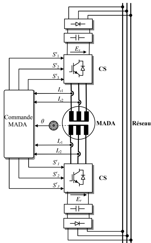
Figure 2. 1. Structure du système étudié.
