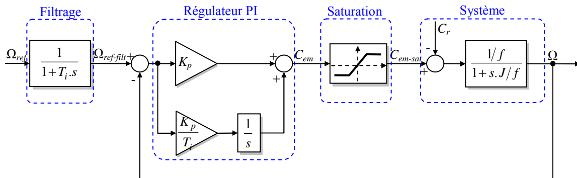
Figure2. 5. Structure de régulation de la vitesse mécanique.
