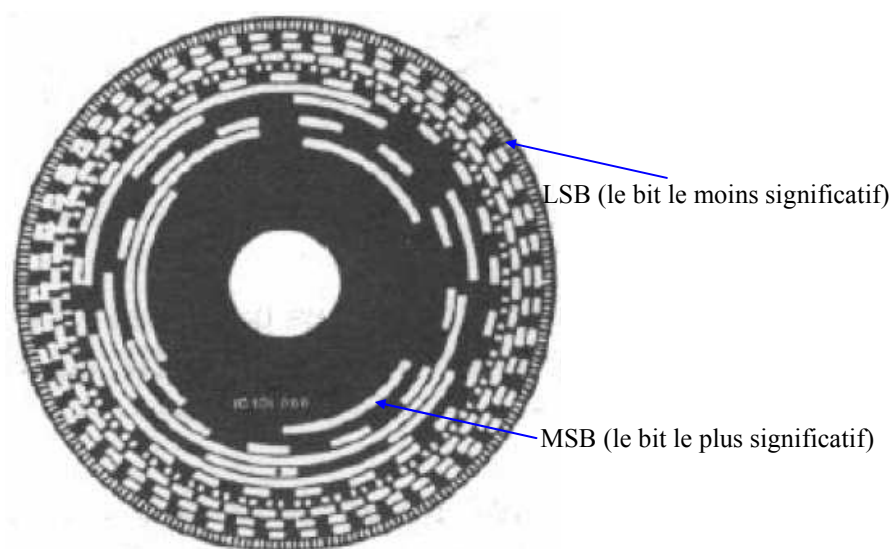
Figure 1. 15. Le disque du codeur absolu [12].
