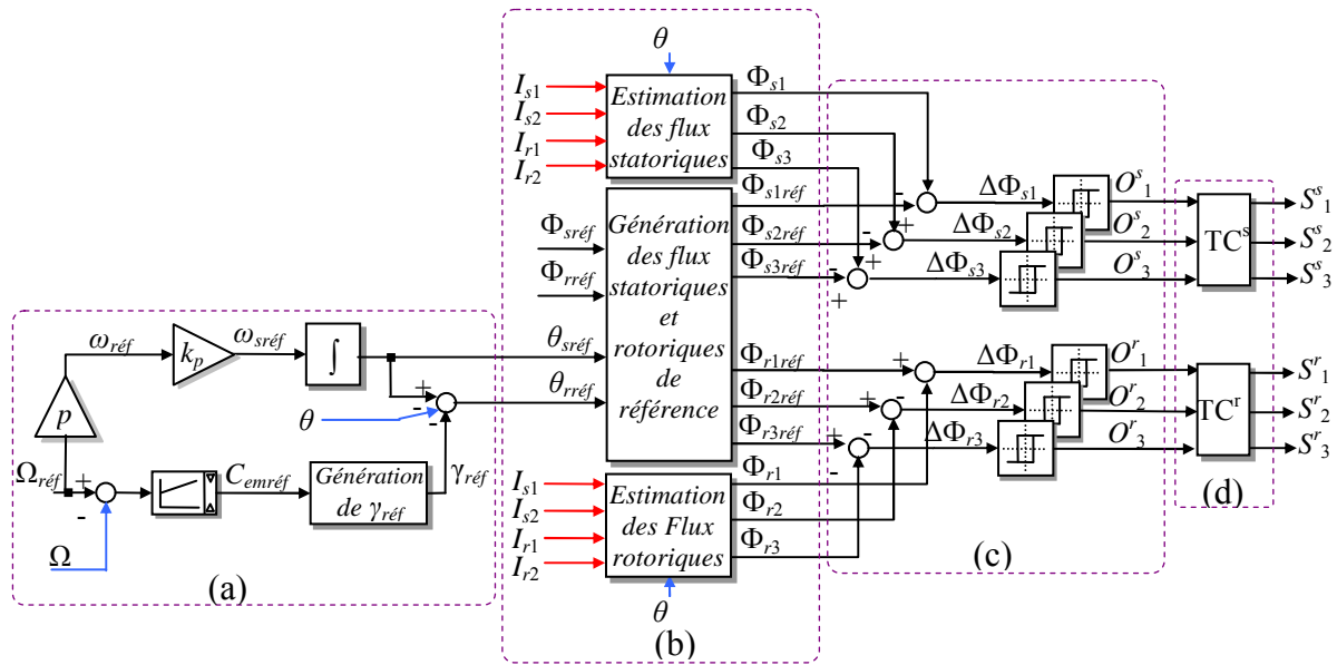
Figure2. 4. Commande optimisée de la vitesse mécanique et du vecteur flux pour une MADA.
