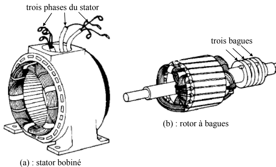
Figure 1. 19. Représentation des structures (a) : du stator et (b) : du rotor bobiné de la MADA [21].
