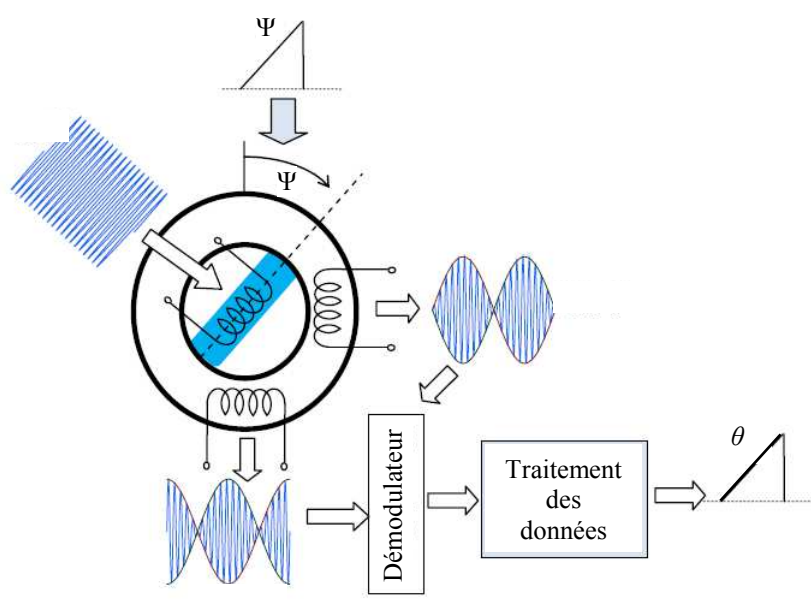
Figure 1. 11. Principe du capteur résolveur [16].
