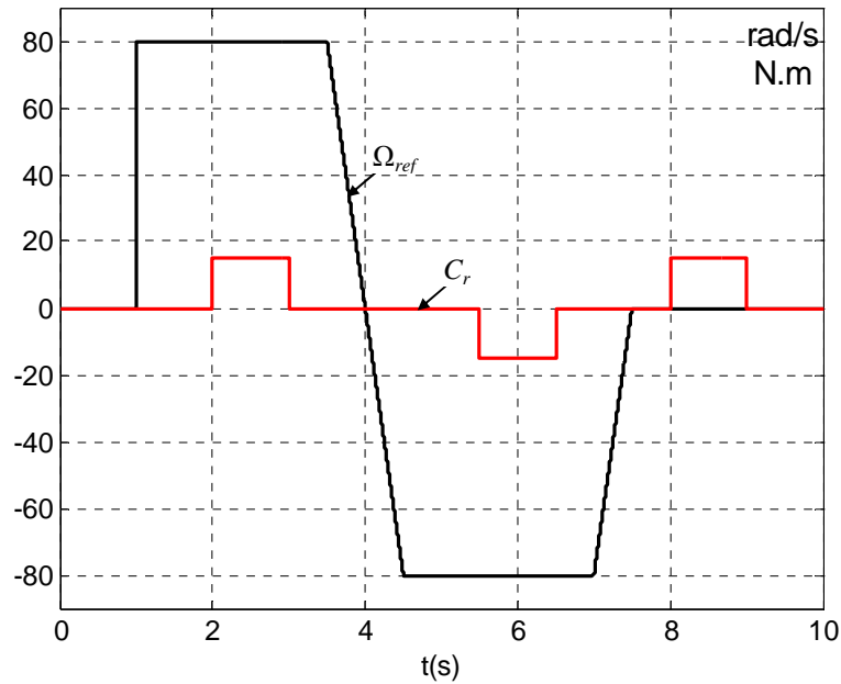
Figure 3. 11. Le cycle de fonctionnement imposé à la machine.
