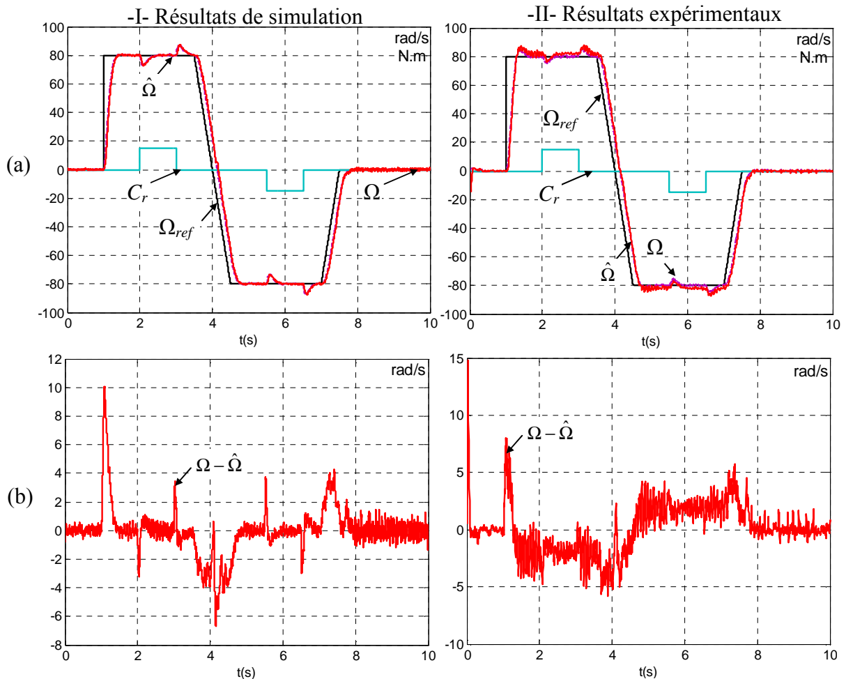
Figure 4. 8. Fonctionnement en BO de l'estimateur
