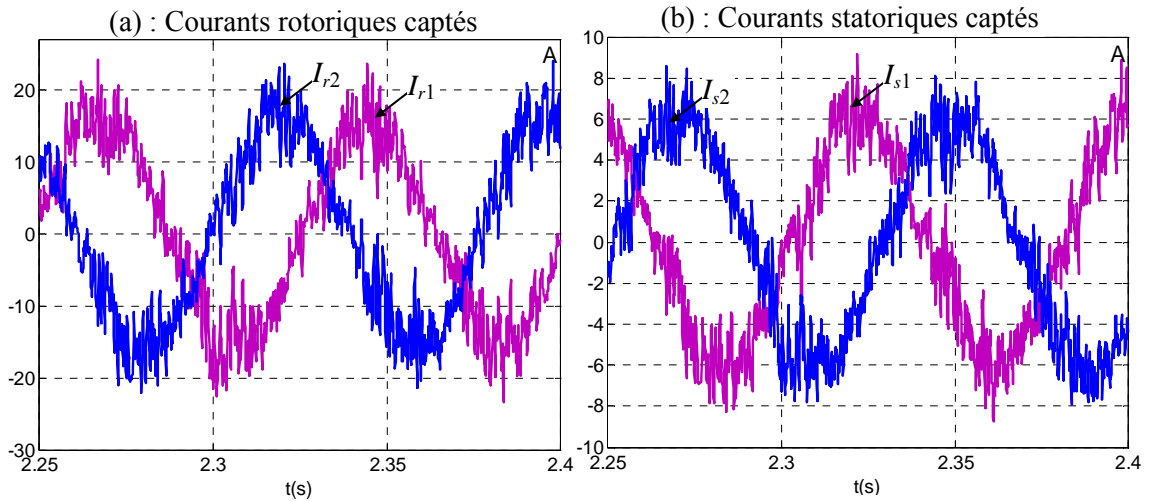
Figure2. 14. Les courants statoriques et rotoriques captés sur la maquette.
