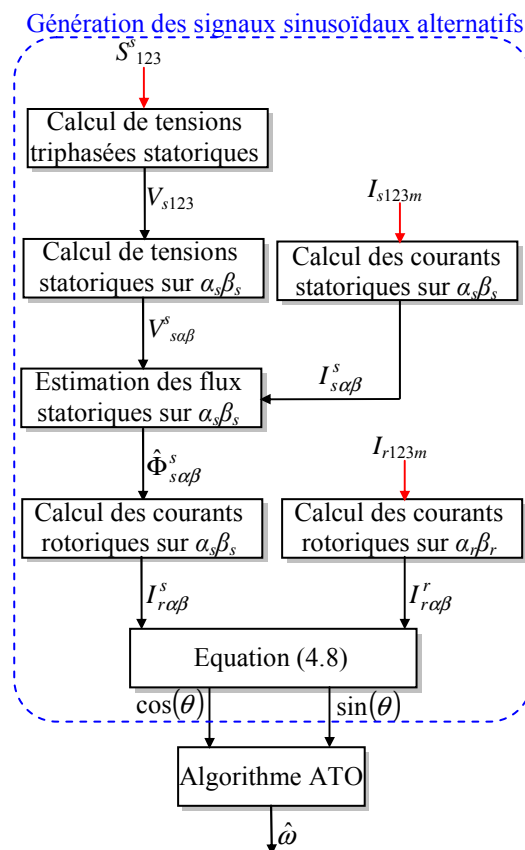
Figure 4. 3. La méthodologie suivie appliquant l'algorithme ATO.
