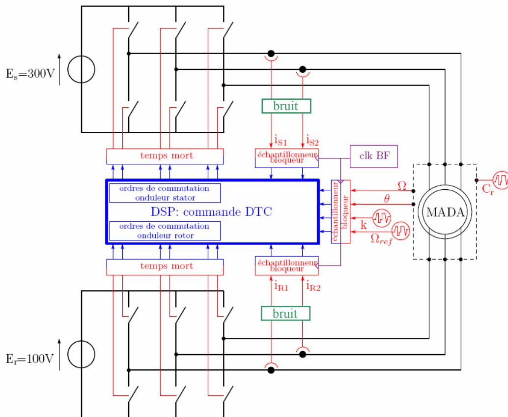
Figure2. 7. Schéma de simulation du système.
