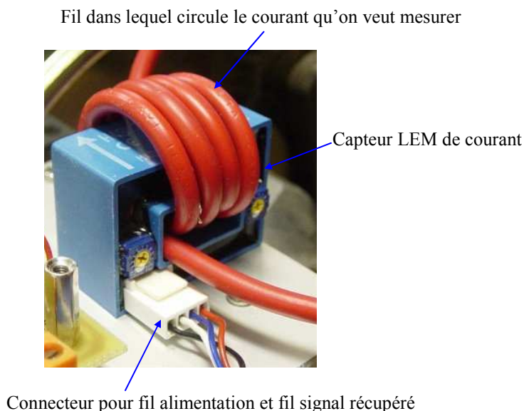
Figure 1. 10. Exemple d'un capteur à effet Hall de type LEM monté en circuit [15].
