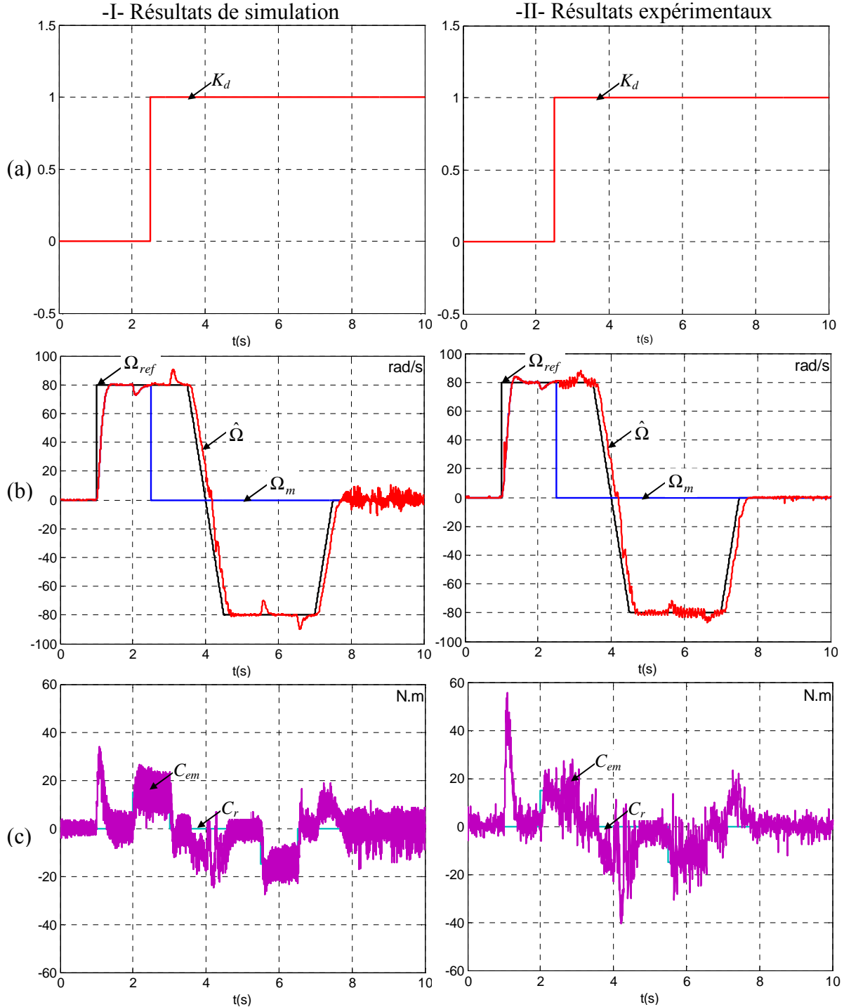
Figure 4. 22. Fonctionnement en supervision et application d'un défaut simulant la perte d'information à la sortie du capteur de vitesse à l'instant t = 2.5s (a) : le marqueur permettant la détection et la reconfiguration, (b) : allures de la vitesse avant et après défaut, (c) : allure du couple électromagnétique avant et après défaut.
