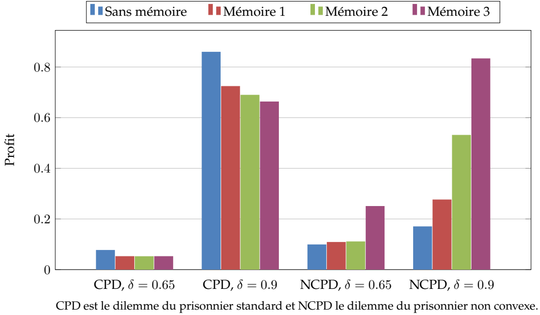
FIGURE 1.1 : Profit moyen après n = 2 \cdot 10^6 étapes
