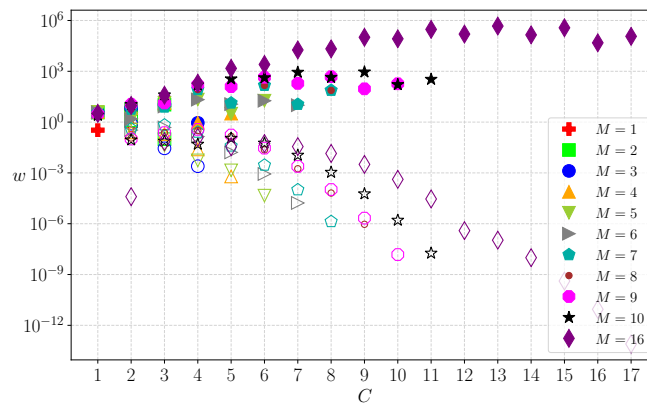
FIGURE 4.6 – Amplitudes des coefficients : Comparaison pour différents ordres M = [1, 16] entre les deux cas de régression LSE (symboles pleins) et RLS (symboles vides).
