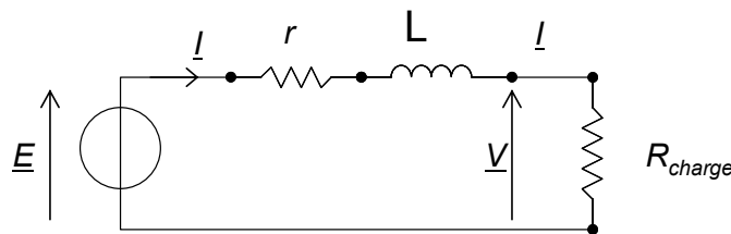
figure IV.54 : circuit électrique monophasé équivalent représentatif du montage.
