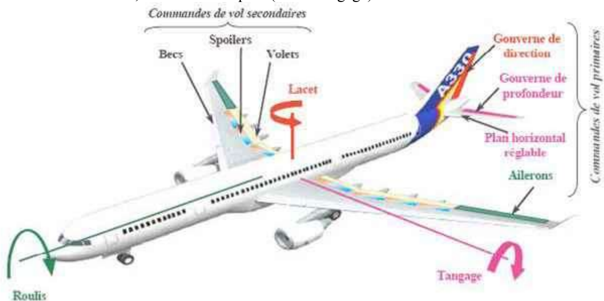
figure I-1 : axes et gouvernes de l'avion.
