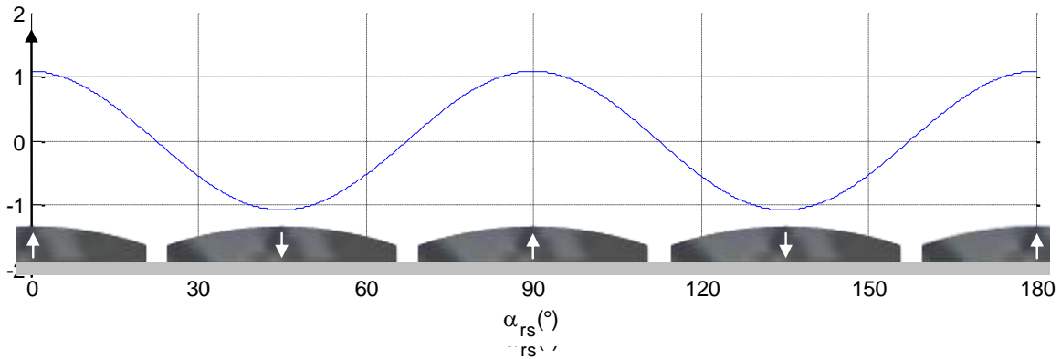
figure III.18 : distribution spatiale des aimants d'une couronne rotorique avec \beta_r = \pi/(2.p)
