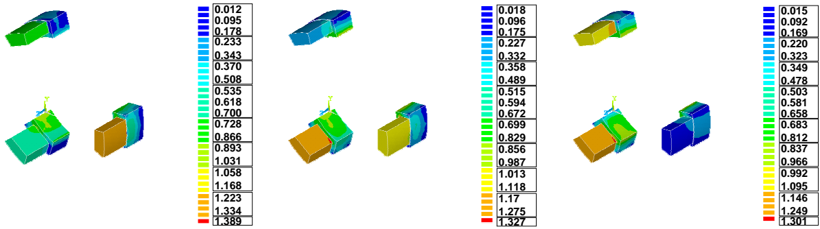
figure IV.9 : évolution de l'induction magnétique dans les plots pour 3 positions (0° ; 11.25° ; 22.5°)
