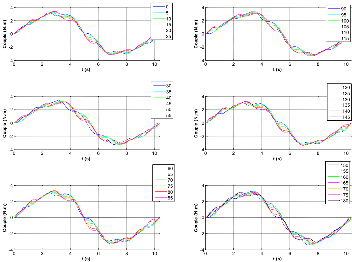
figure IV.47 : Variation du couple moteur en fonction du temps pour différentes positions électriques du stator (tous les 5° électriques).
