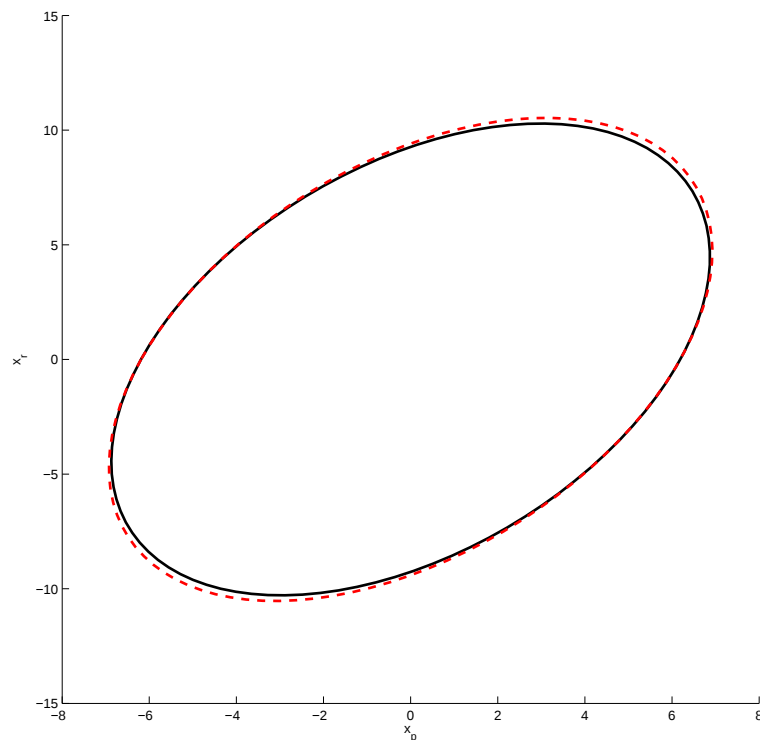
Figure 8: Domaine de stabilité du système saturé avec (ligne continue noire) ou sans réinitialisation (ligne pointillée rouge)
