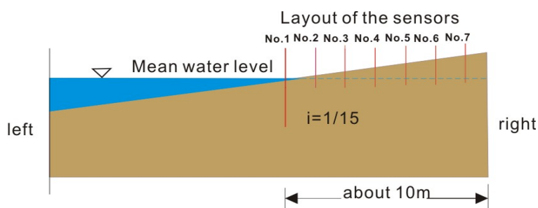
Figure 10 : Schéma de l'arrangement des capteurs capacitifs dans la zone de swash en coupe vertical. Le Capteur N°1 est le plus proche de l'eau libre.
