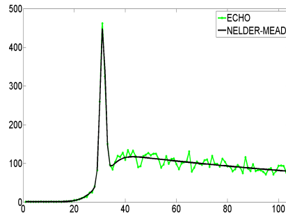
FIG. 4.6 – Forme d'onde avec swh = 10m et un pic sur le front de montée.
