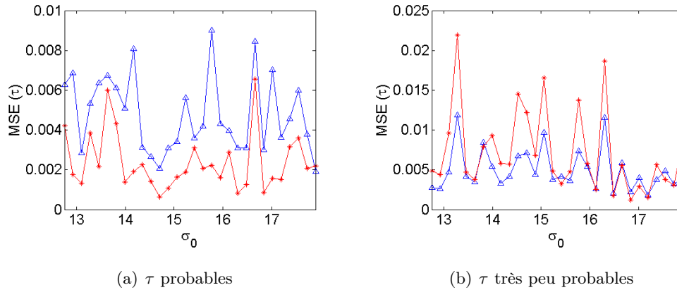
FIG. 2.5 – Comparaison des MSEs en fonction de \sigma_0 : \text{---}* MCMC et \text{---}\triangle MLE
