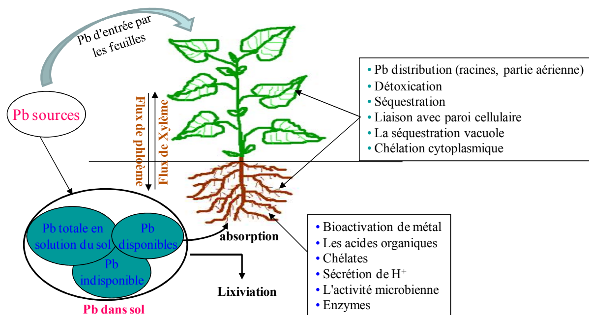
Figure-1. Comportement biogéochimique du plomb dans le sol, l'absorption par les racines et l'accumulation ainsi que les mécanismes de détoxification adoptée par les plantes contre la toxicité du plomb.
