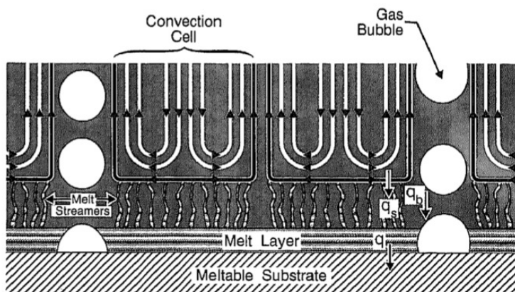
FIG. I.7: Représentation de l'interface entre le corium et le béton proposée par Epstein [53]
