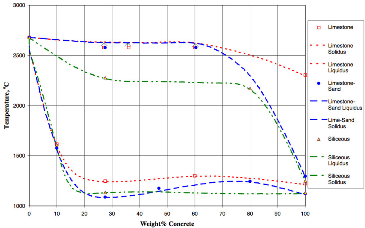
FIG. I.3: Diagramme de phases pseudo-binaires pour les mélanges \text{UO}_2\text{-ZrO}_2\text{-béton} (calcaire ( cf. limestone), siliceux ( cf. siliceous), silico-calcaire ( cf. limestone-sand)) [129].
