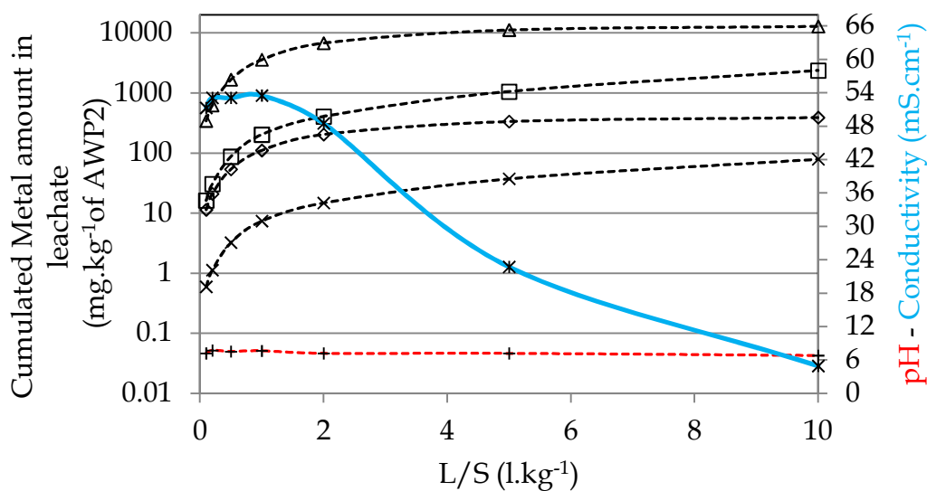
Figure 93 : Percolated amount of calcium (---□---), phosphorus (---◇---), sulfur (---Δ---) and strontium (---×---) from column percolation test of AWP2 blend in function of leaching time, pH (---+---) and conductivity (---+---)
