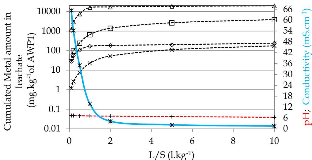
Figure 92 : Percolated amount of calcium (---□---), phosphorus (---◇---), sulfur (---Δ---) and strontium (---×---) from column percolation test of AWP1 blend in function of leaching time, pH (---+---) and conductivity (---+---)
