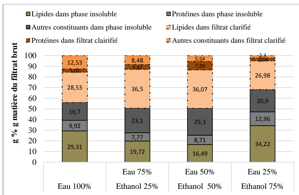
Figure III-14 : Composition de la matière sèche des filtrats bruts obtenus par extraction aqueuse et hydro-éthanolique des graines de neem en extracteur-séparateur bi-vis BC 21
