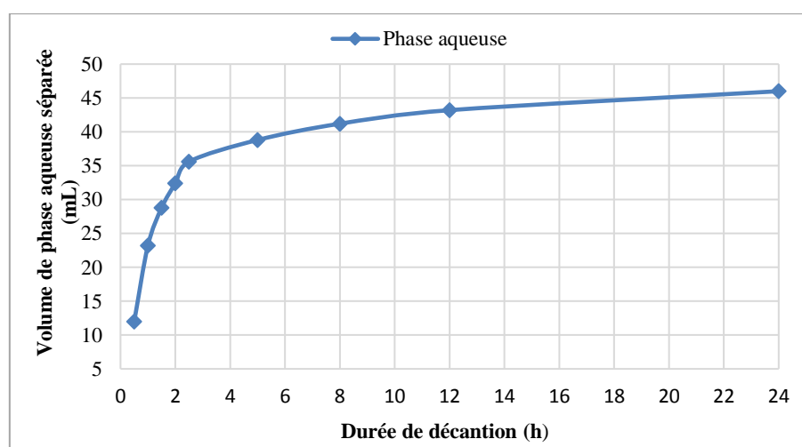
Figure IV-4 : Cinétique de la décantation en éprouvette du filtrat à température ambiante après homogénéisation sous pression
