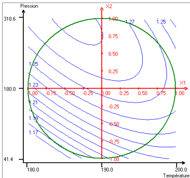
Figure VI-13 : Courbes d'isoreponses de la densité du matériau obtenu par thermopressage du raffinat d'extrusion des graines de neem en fonction de la pression et de la température pour un temps de pressage de 2 minutes
