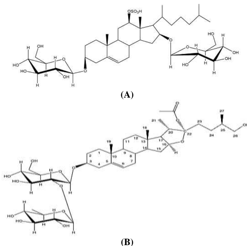
Figure I-3 : Structure des saponines, balanitine 1 (A) et balanitine 2 (B) isolées des graines de Balanites aegyptiaca (Speroni et al. , 2005)
