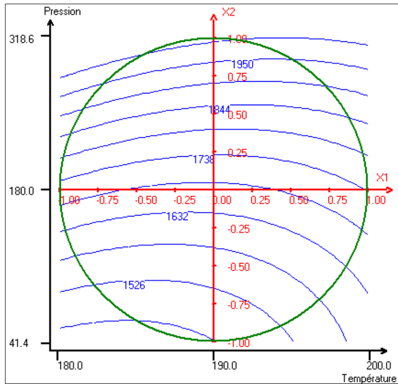
Figure VI-12 : Courbes d'isoreponses du module d'élasticité en flexion du matériau obtenu par thermopressage du raffinat d'extrusion des graines de neem en fonction de la pression et de la température pour un temps de pressage de 2 minutes
