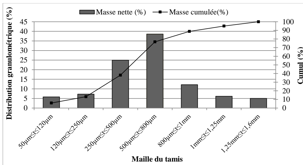
Figure IV-6 : Distribution granulométrique des particules du raffinat solide obtenu par fractionnement aqueux des graines de neem en extrudeur bi-vis de type Clextaral BC 21
