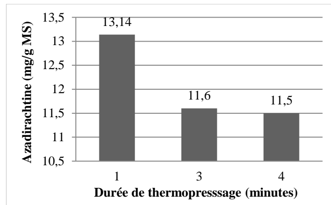
Figure IV-24 : Teneur en azadirachtine des matériaux thermopressés (200°C, 200 kg/cm 2 ) à partir du raffinat d'extrusion des graines de neem
