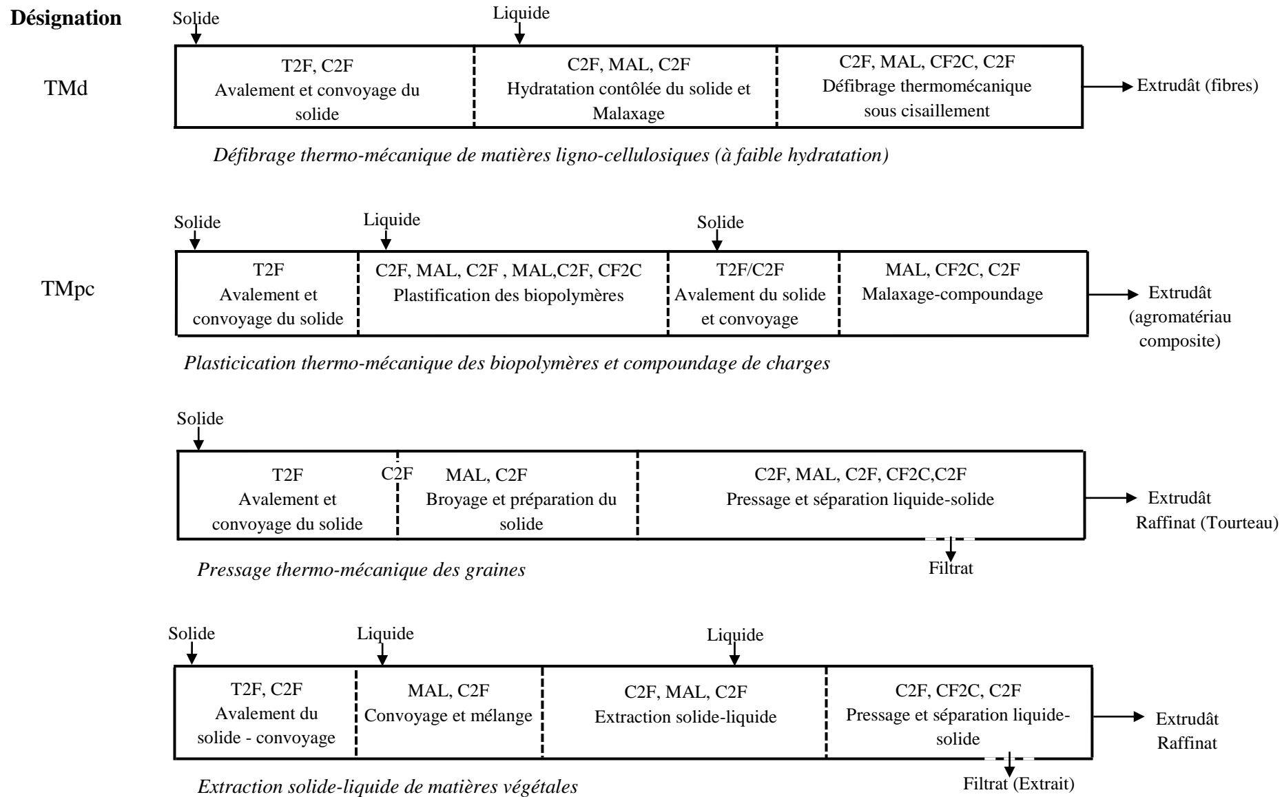
Figure I-10 : Exemples d'opérations unitaires, configurations et de profils de vis mis en œuvre dans le fractionnement de matières végétales
