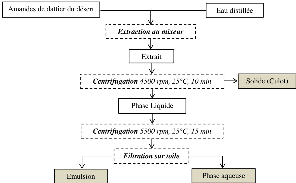
Figure V-3 : Schéma du fractionnement aqueux des amandes de dattier du désert au Mixeur
