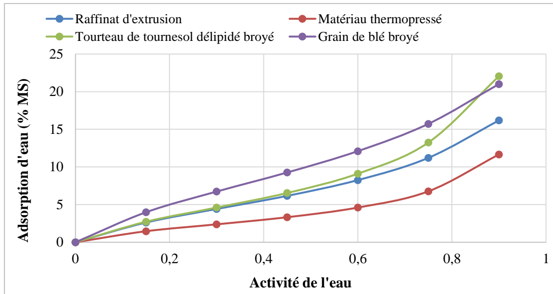
Figure IV-23 : Comparaison du tracé des isothermes d'adsorption d'eau d'après le modèle GAB pour le raffinat d'extrusion des graines de neem, le matériau thermopressé (200°C, 200 kg/cm 2 , 4 min), le tourteau de tournesol délipidé broyé et le grain de blé broyé
