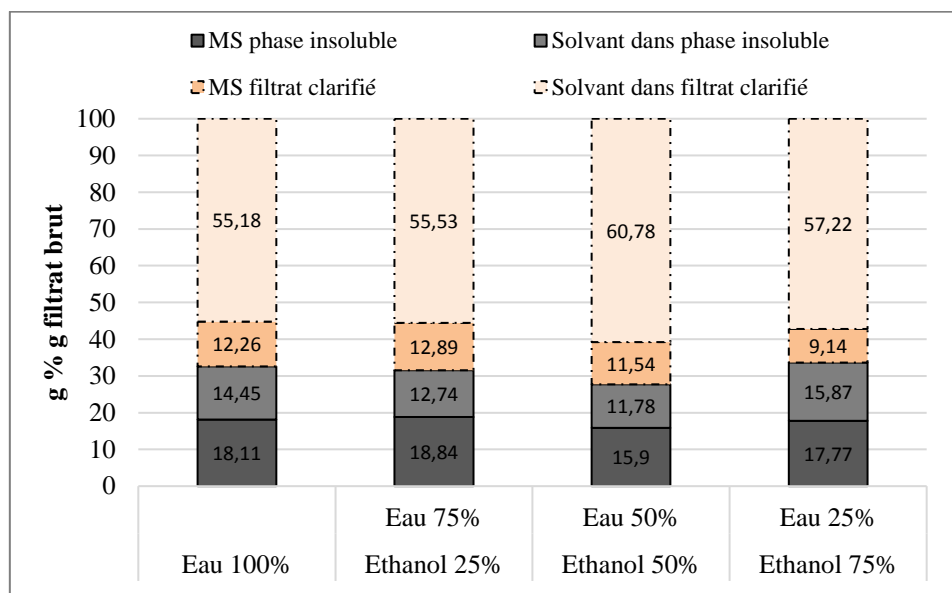
Figure III-12 : Répartition des phases des filtrats bruts obtenus par extraction aqueuse et hydro-éthanolique des graines de neem en extracteur-séparateur bi-vis BC 21
