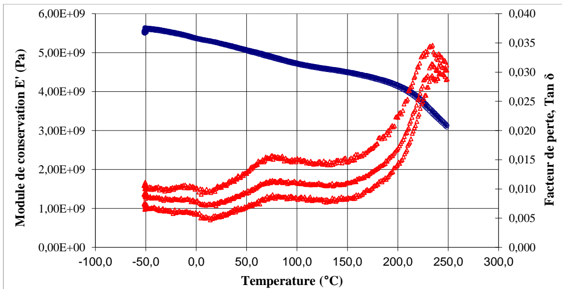
Figure IV-9 : Spectres DMA du raffinat solide issu du fractionnement des graines de neem en extrudeur bi-vis de type Cleextral BC 21 : évolution du module de conservation E' et du facteur de perte \text{Tan } \delta , en fonction de la température pour trois fréquences (1 Hz, 5 Hz et 10 Hz)
