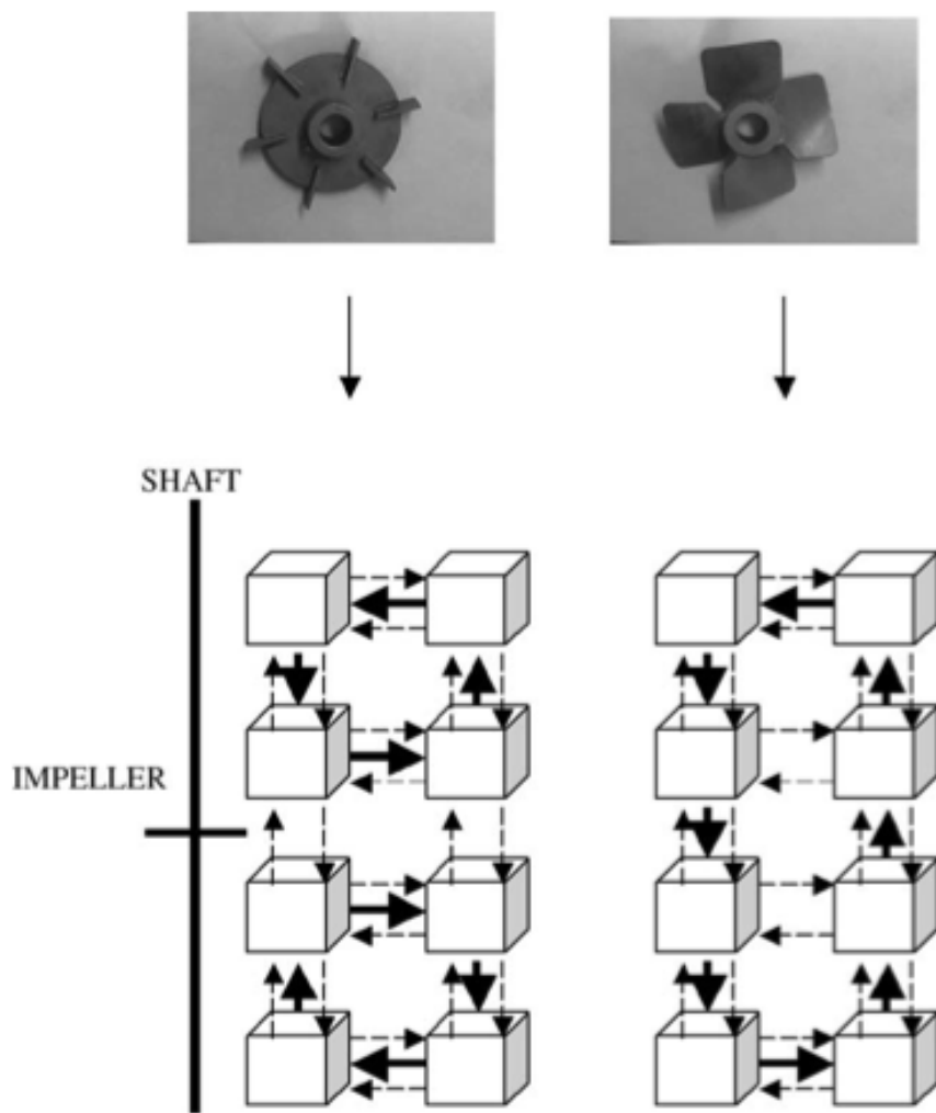
FIGURE 1.8: Schéma simplifié de l'association de compartiment dans le cas d'une turbine radiale (RDT6 à gauche) et axiale (A315 à droite) (Delvigne et al., 2005a). Les flèches --> et <-- représentent les flux diffusifs et \rightarrow les flux convectifs.
