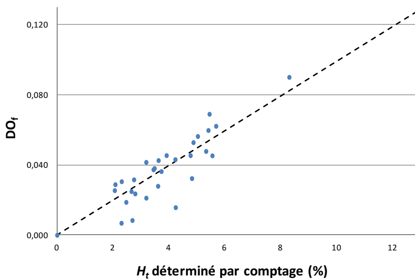
FIGURE 3.2.2: Mesure de l'hématocrite de tube à partir de la densité optique. Variation de la densité optique ( DO_f ) avec l'hématocrite déterminé par comptage, mesurée sur les canaux de section 20\mu\text{m} \times 20\mu\text{m} (points bleus). Nous avons déterminé DO_f = 0,0099 \times H_t (courbe pointillée).
