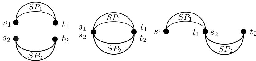
Figure 1.2 – La composition en série (droite) et la composition en parallèle (milieu) de deux graphes série-parallèles SP_1 et SP_2 (gauche).
