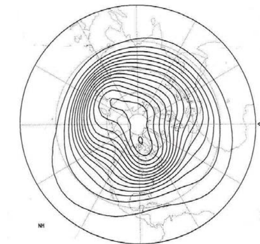
Figure 1.12 – Moyenne temporelle sur six hivers DJF de la hauteur de géopotentielle à 250 hPa dans l'hémisphère nord. L'intervalle entre deux contours est de 100 m. Cette figure est issue de James (1994).
