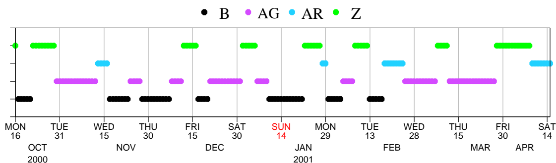
Figure 2.12 – Exemple d'association d'un régime à une date pour l'hiver étendu du 16 octobre 2000 au 15 avril 2001. Les points noirs représentent le régime du blocage, les points violet le régime de l'anticyclone groenlandais, les points bleus le régime de dorsale Atlantique et les points verts le régime zonal.
