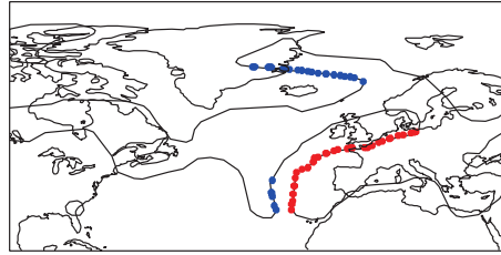
Figure 2.2 – Représentation des contours de PV à 2 pvu et 6 pvu en noir. Les ronds rouges montrent les zones du contour qui appartient à un déferlement anticyclonique et les ronds bleus les zones qui appartient à un déferlement cyclonique.
