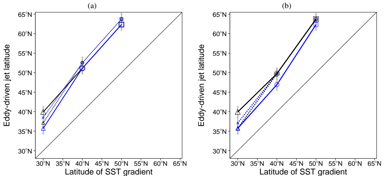
Figure 4.10 – Latitude de l'« eddy-driven » jet (latitude du maximum de la moyenne zonale et temporelle du vent zonal à 850 hPa) en fonction de la latitude à laquelle est centré le front de SST pour a) les expériences T0 et b) les expériences T1. Les codes de couleur et les symboles sont identiques à ceux de la figure 4.7. Les barres d'erreur sont indiquées en gris et représentent \pm 1,5^\circ .
