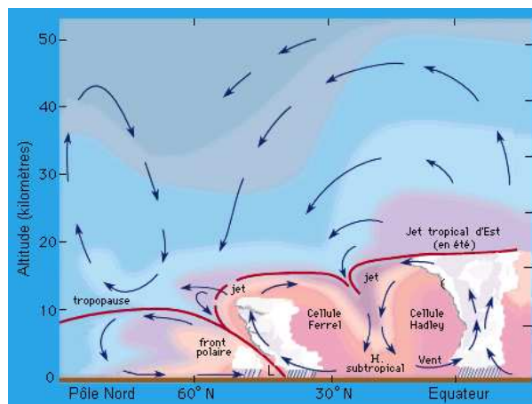
Figure 1.4 – Représentation schématique des différentes circulations atmosphériques autour de l'hémisphère nord. Cette image est issue du site internet http://www.astrosurf.com/luxorion/meteo-massesdair.htm .
