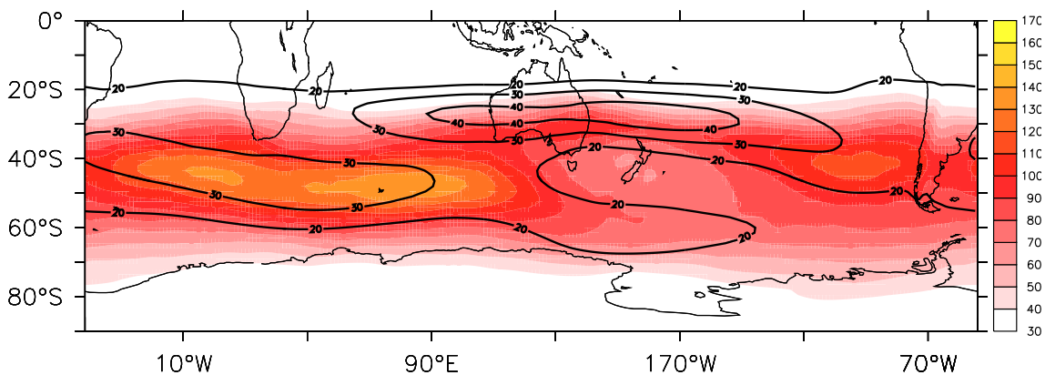
Figure 4.24 – Energie cinétique haute fréquence en \text{m}^2 \cdot \text{s}^{-2} (plages colorées) et vent zonal (contours noirs, premier contour : 20 \text{ m} \cdot \text{s}^{-1} , intervalle : 10 \text{ m} \cdot \text{s}^{-1} ) à 300 hPa dans l’hémisphère sud sur JJA de 1958 à 2001 sur les 44 ans des réanalyses ERA40.
