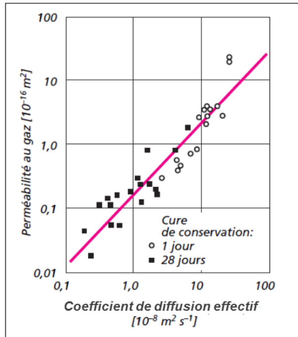
Fig.I. 8: Perméabilité au gaz du béton en fonction du coefficient de diffusion (tiré de Hermann, 2000)
