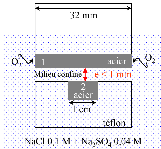
Figure IV-10 : Schéma de la cellule à couche mince utilisée pour reproduire les conditions rencontrées lors de la corrosion caverneuse
