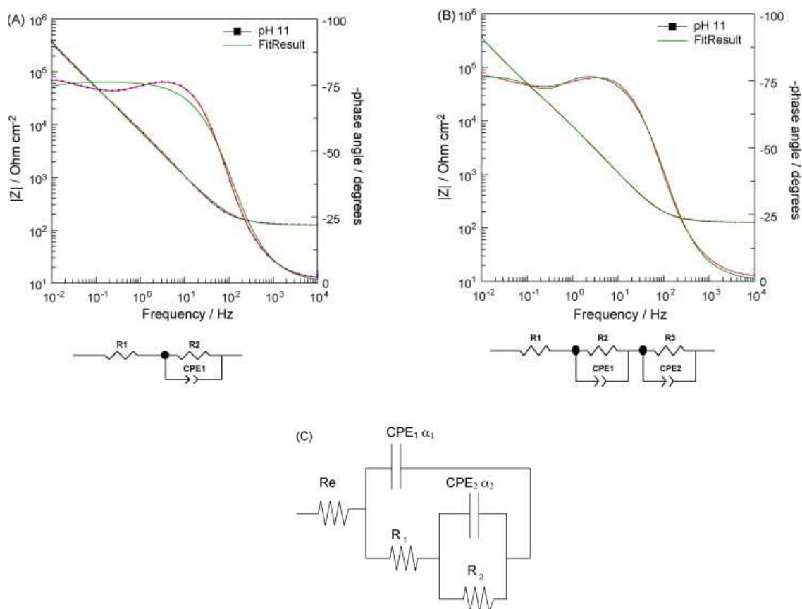
Figure I-4 : Résultats des ajustements obtenus pour l'acier inoxydable AISI 316 en milieu alcalin et aéré à l'aide de circuits électriques équivalents composés de : (a) un élément R//CPE, (b) deux éléments R//CPE en série et (c) deux éléments R//CPE en parallèle [Fre10]
