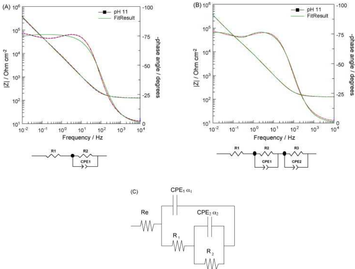
Figure I-4 : Résultats des ajustements obtenus pour l'acier inoxydable AISI 316 en milieu alcalin et aéré à l'aide de circuits électriques équivalents composés de : (a) un élément R//CPE, (b) deux éléments R//CPE en série et (c) deux éléments R//CPE en parallèle [Fre10]
