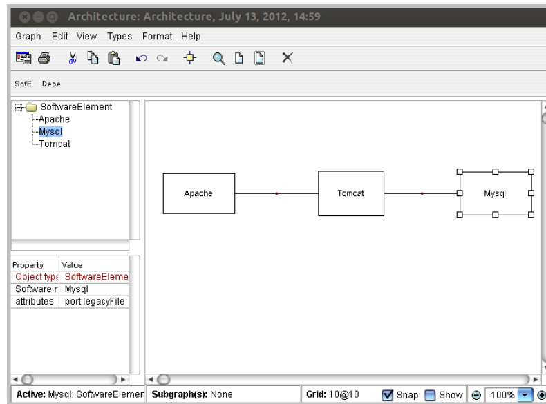
FIGURE 6.16 – Éditeur généré avec MetaEdit+
