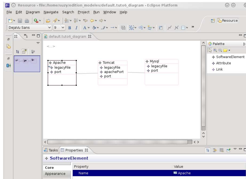
FIGURE 6.8 – Éditeur généré
