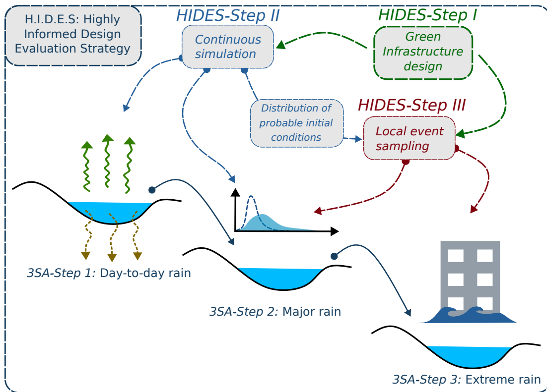
Figure E.2: Cadre d'évaluation des techniques de gestion à la source des eaux pluviales HIDES ( Highly Informed Design Evaluation Strategy - stratégie d'évaluation informée des méthodes de dimensionnement).
