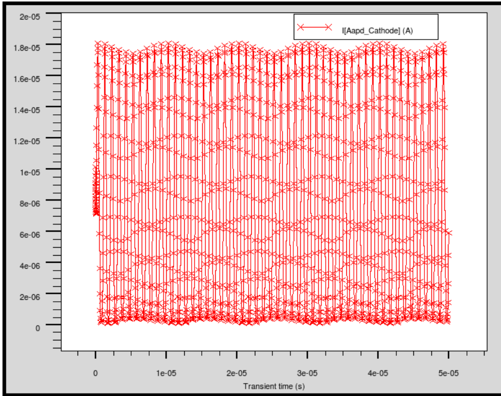
Figure III-ad : Simulation temporelle du mélange optoélectronique de l'APD N + P 1 .
