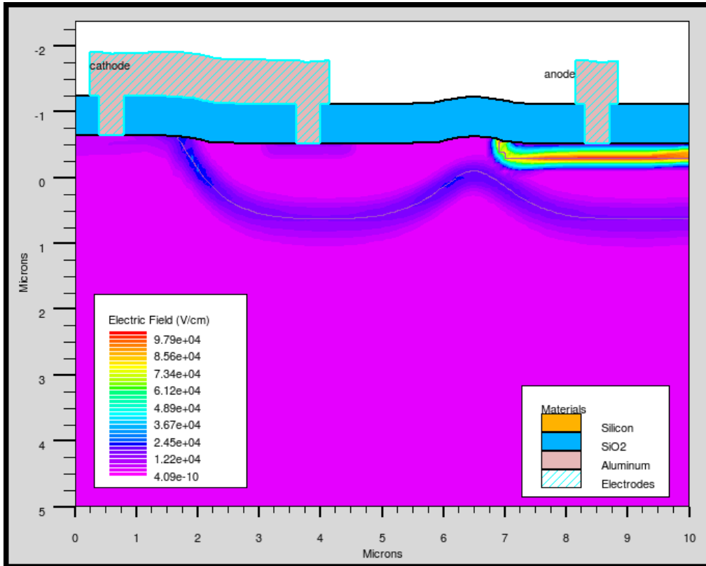
Figure III-i : Distribution du champ électrique au sein de l'APD P + N + NI pour une tension inverse de -5 V.
