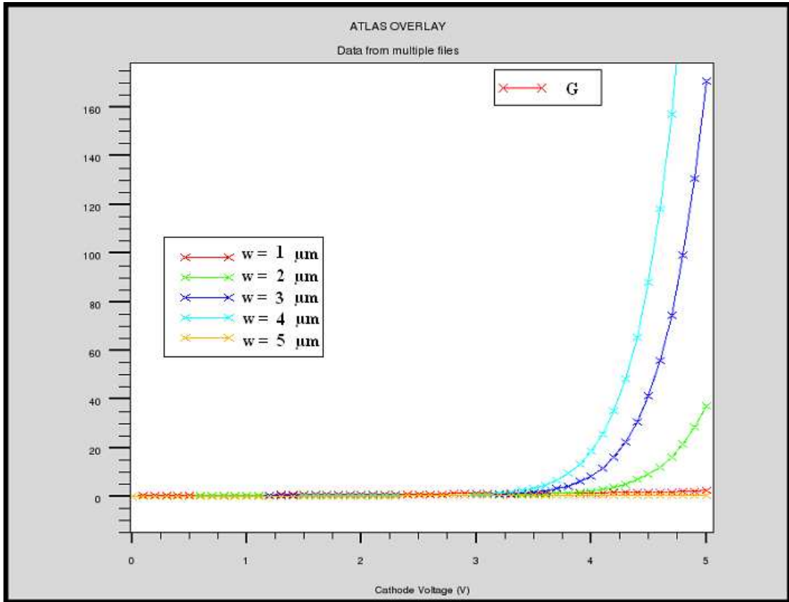
Figure III-bn : Gain photoélectrique de la photodiode MSM en fonction de la distance W pour un éclairement d'une puissance P_{opt} = 1 \mu W à \lambda = 400 \text{ nm} .
