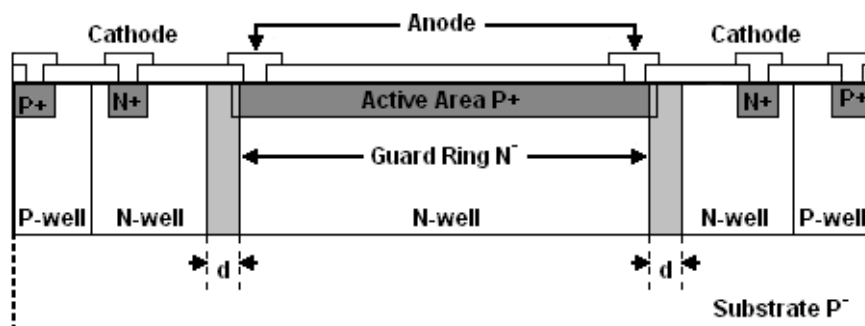
Figure IV-c : Vue en coupe de l'APD montrant l'influence de l'anneau de garde sur la résistance d'accès série.
