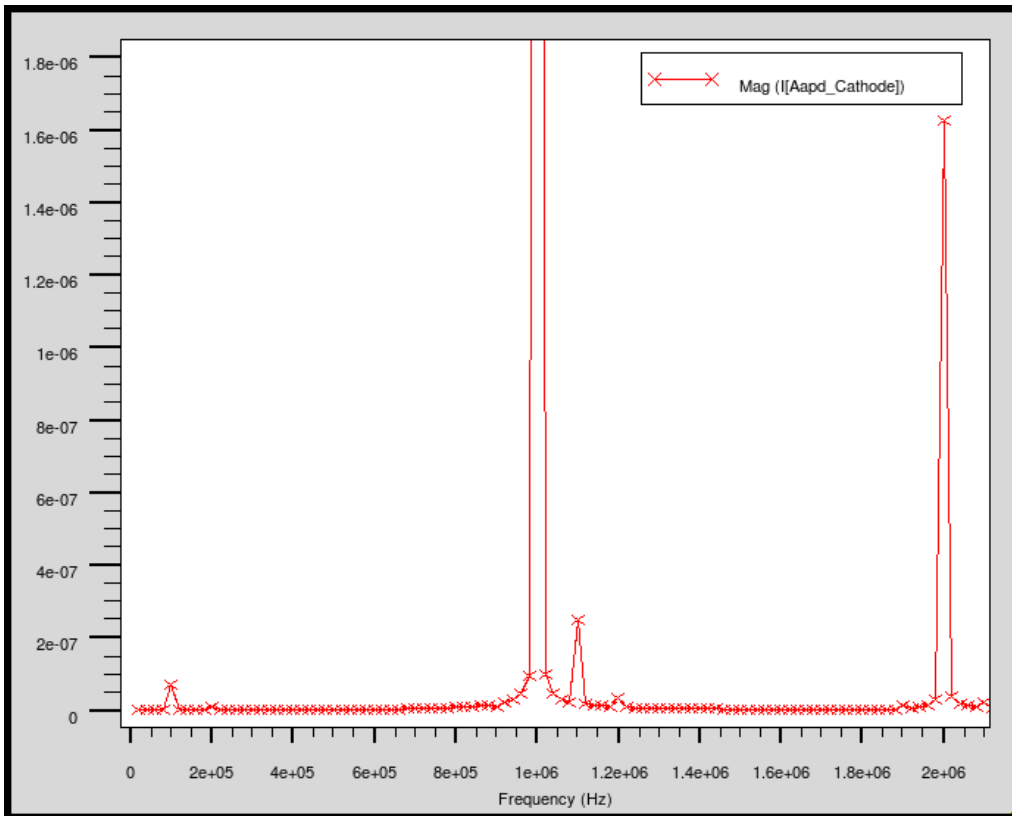
Figure III-ae : Transformée de fourrier du mélange optoélectronique de l'APD P + N 1 .
