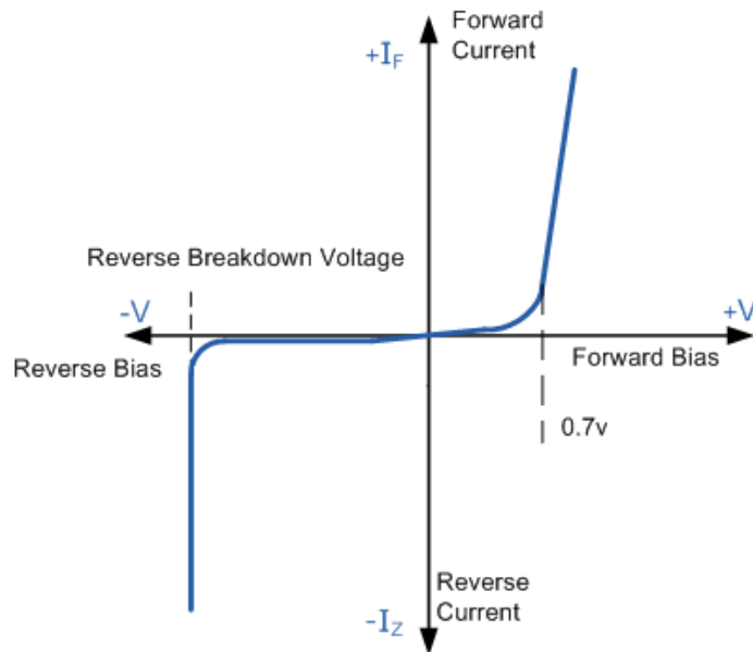
Figure II-d : Caractéristique électrique d'un claquage par effet zener.
