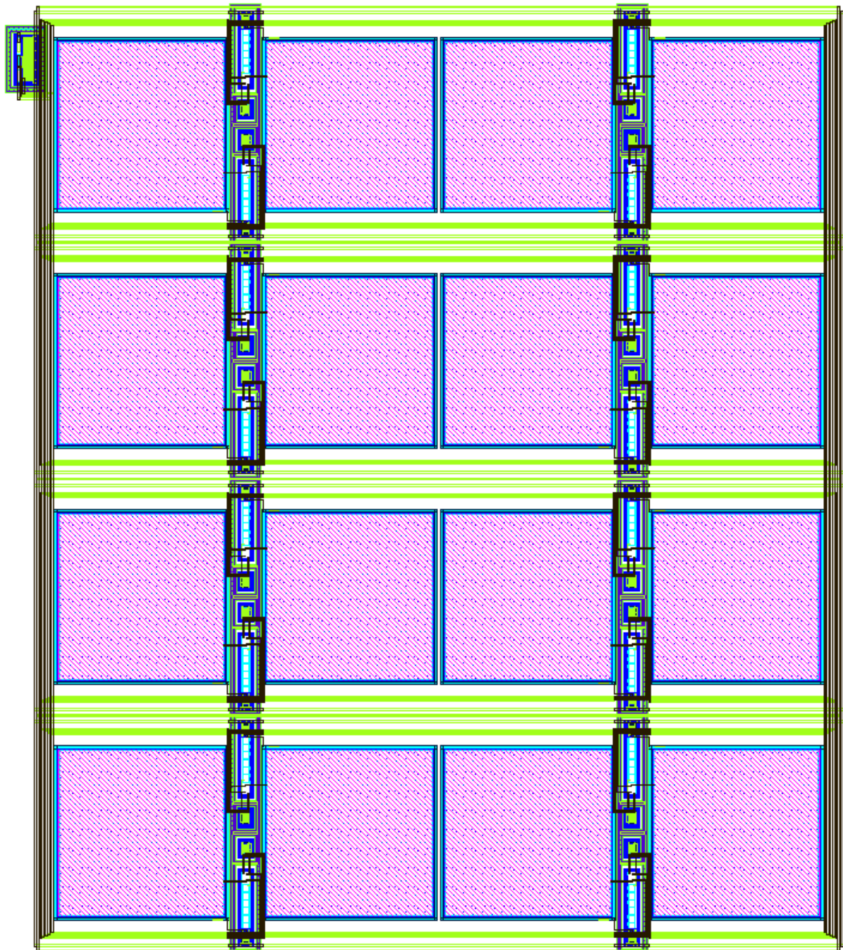
Figure IV-ad : Layout de la matrice d'APD. 1200 \mu\text{m} x 1000 \mu\text{m}
